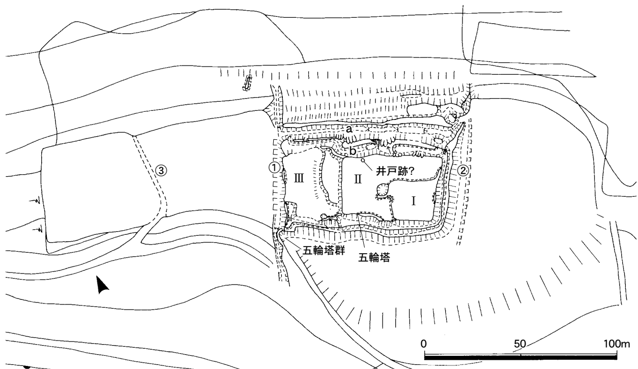
第7図 岡崎城跡縄張り図 (S=1/2,000)
