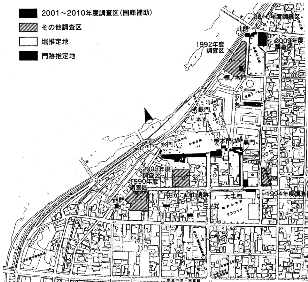
第8図 中津城本丸付近地形図 (S=1/5,000)
