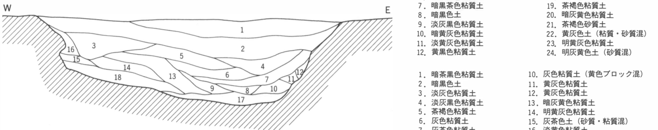
Fig. 4 3SD05土層図 (1/40)
