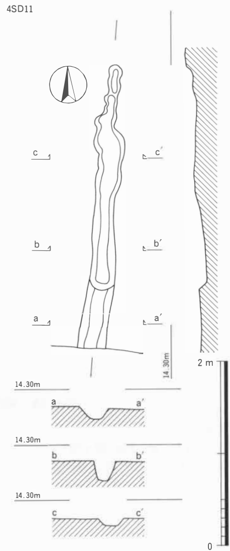
Fig. 18 4SD11実測図 (1/40)
