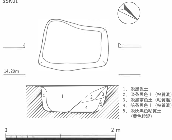
Fig. 5 3SK01実測図 (1/40)
