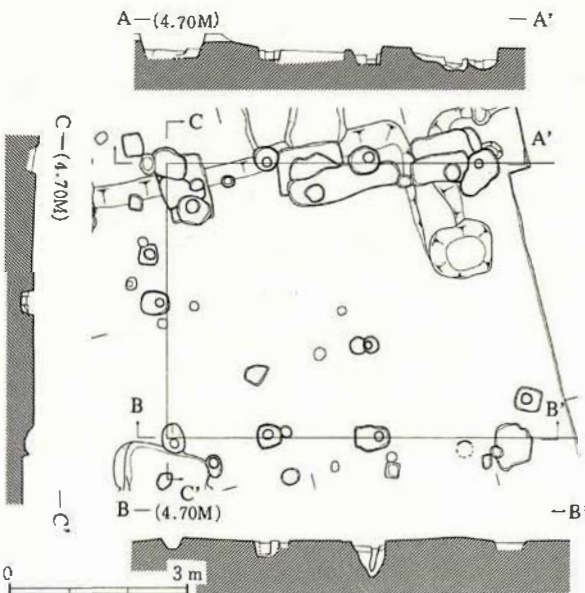
第10図 SB04建物跡
