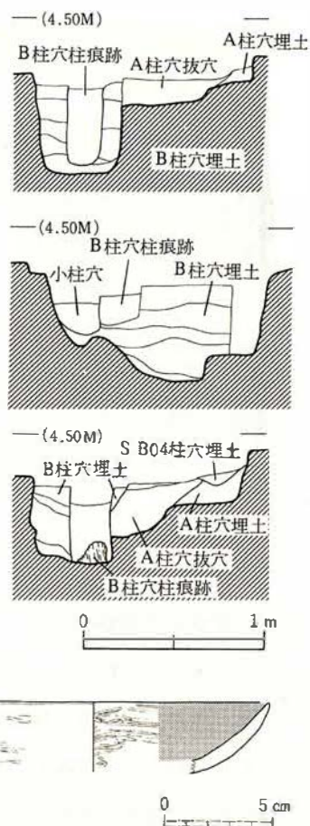
第7図 SB 01建物跡柱穴断面図と出土遺物
