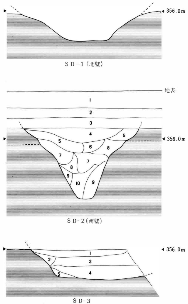
図5 溝跡の土層断面図 (1:40)
