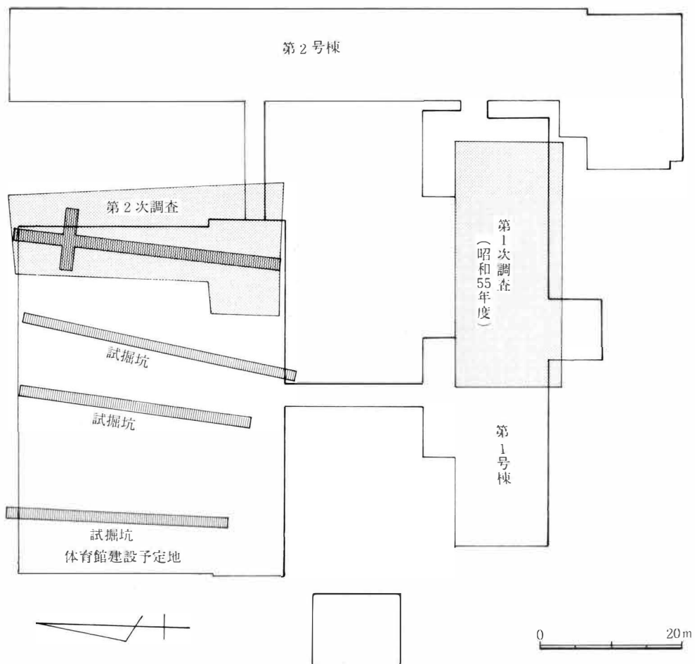
第4図 発掘調査範囲 (1:750)
