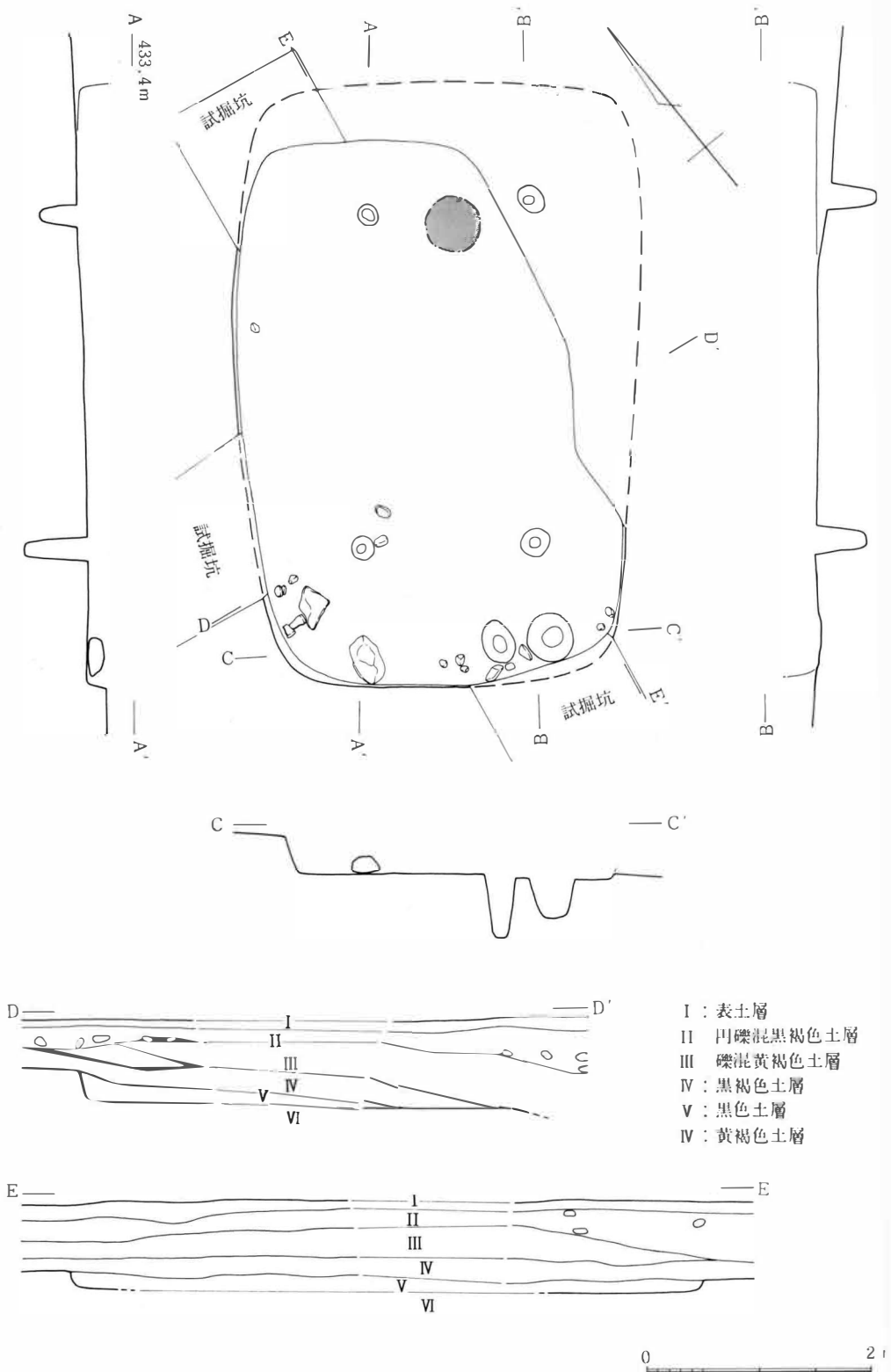
第7図 住居址実測図及び試掘時土層断面図 (1:60)
