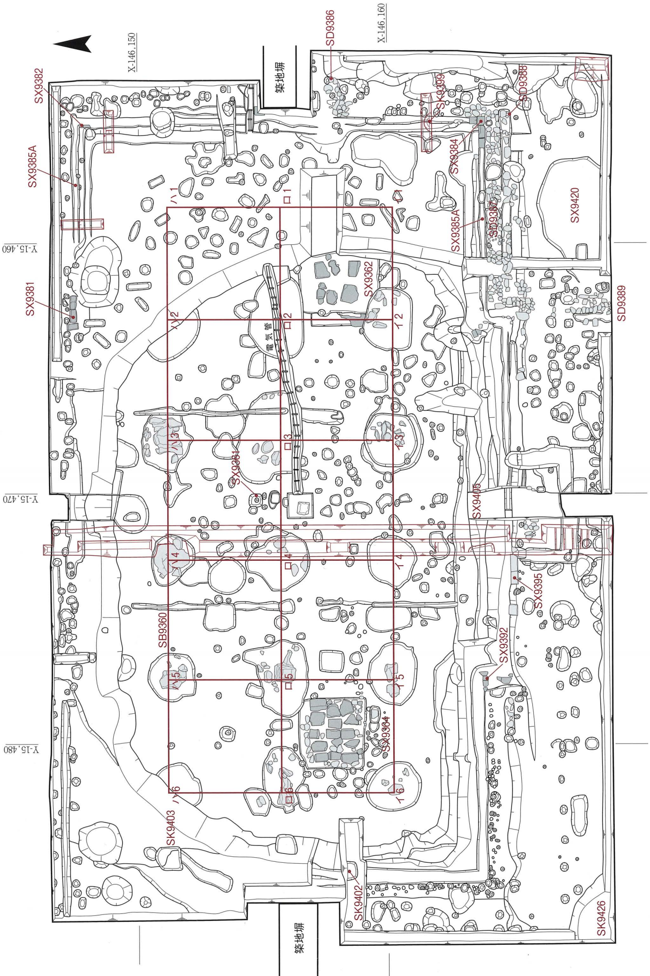
第7図 遺構平面図 (1 : 150)
