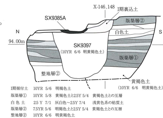
第9図 SK9397断面図 (1:30)
