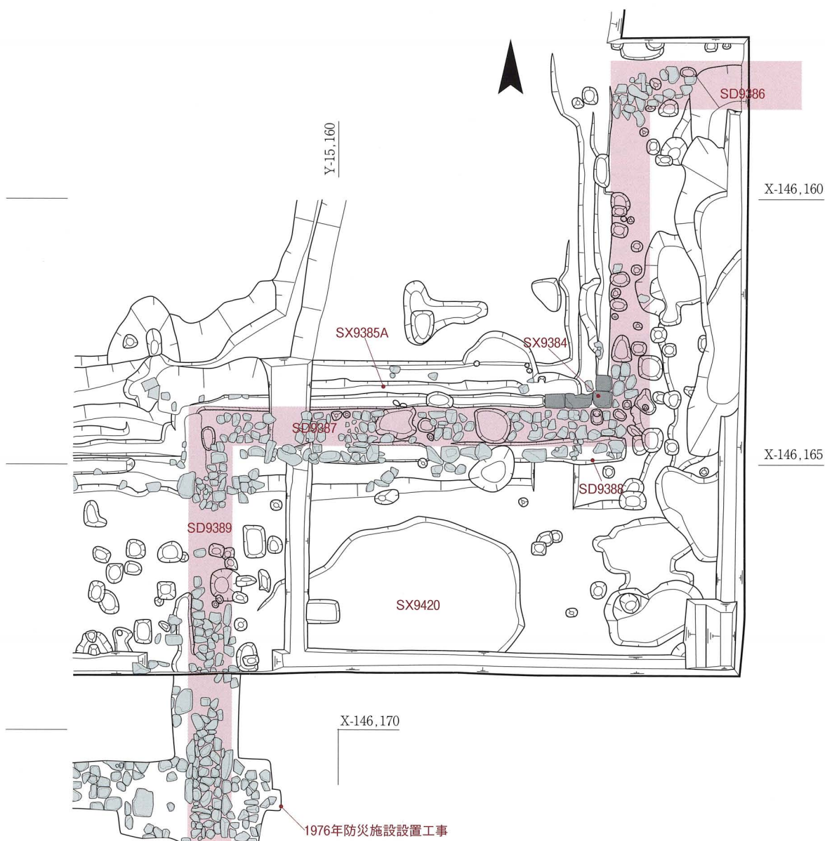
第23図 基壇南東部平面図 (1 : 100)
