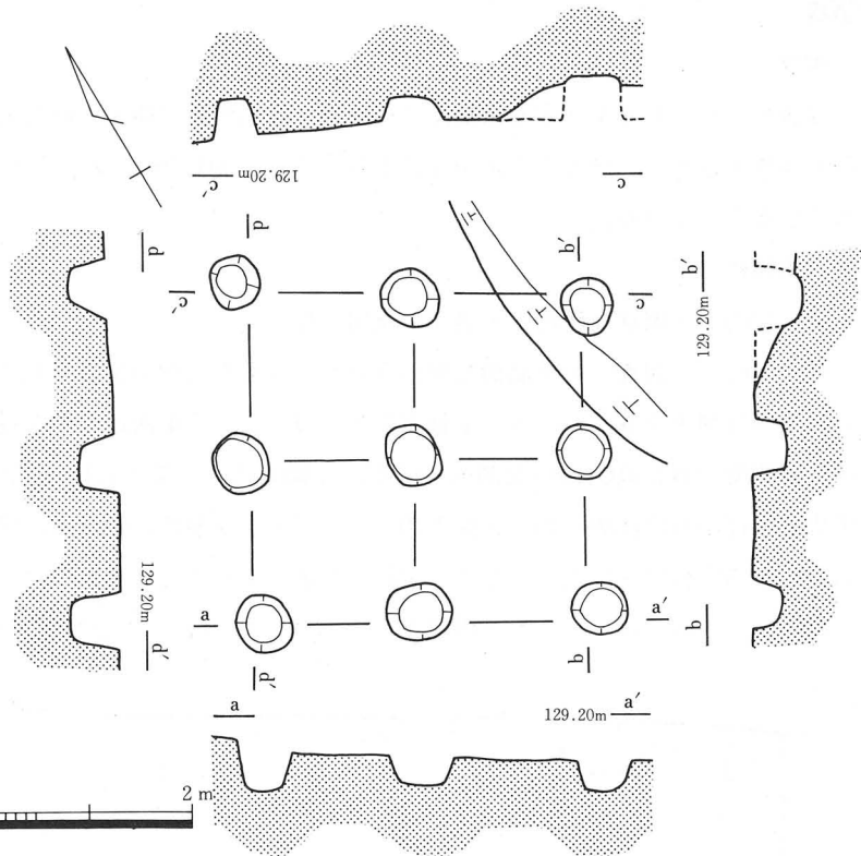
第4図 掘立柱建物遺構実測図(1/80)
