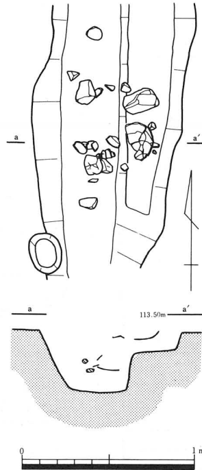
第23図 溝3 遺物出土状況図(2)
