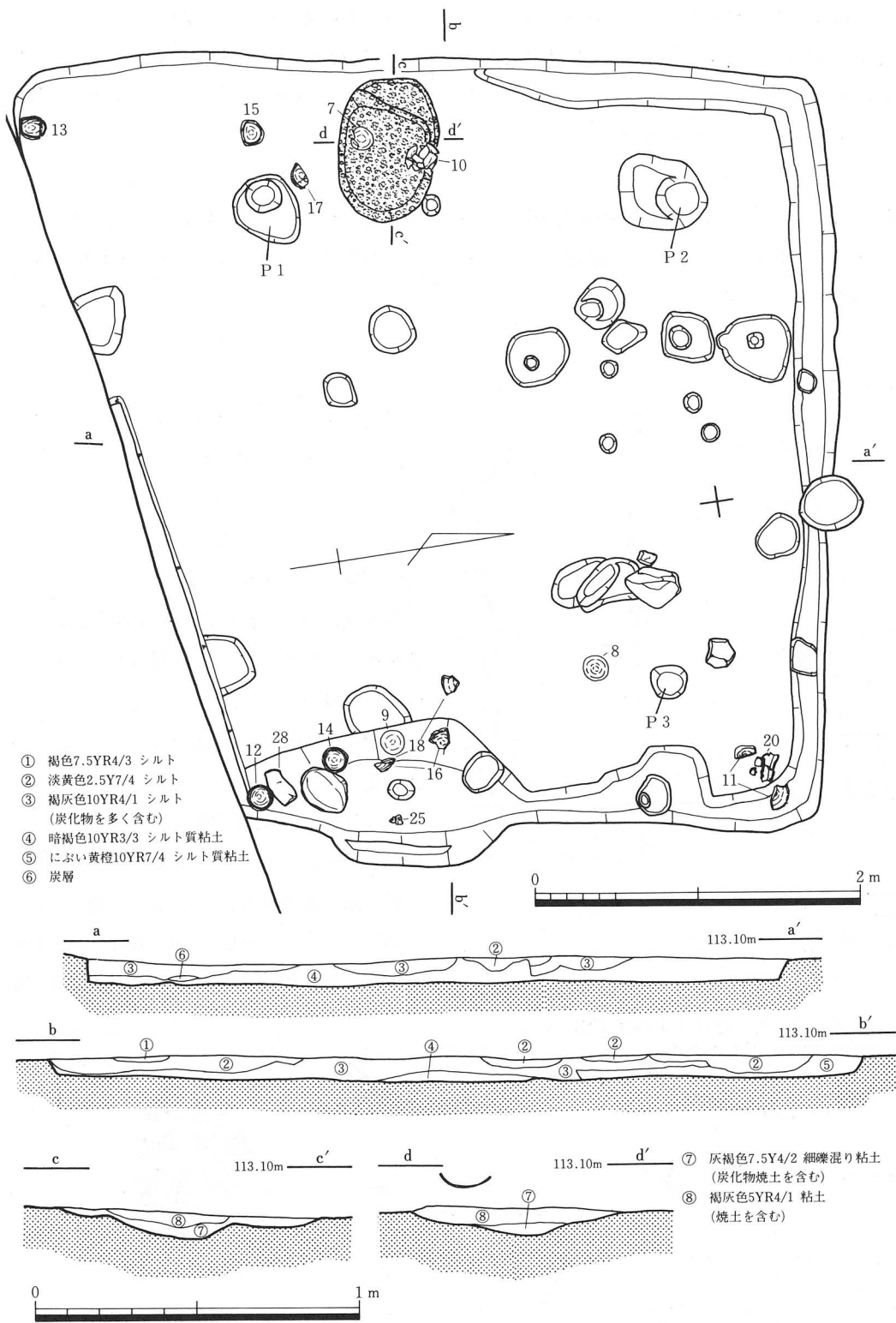
第14図 竪穴住居2遺構実測図及び竈状遺構断面図
