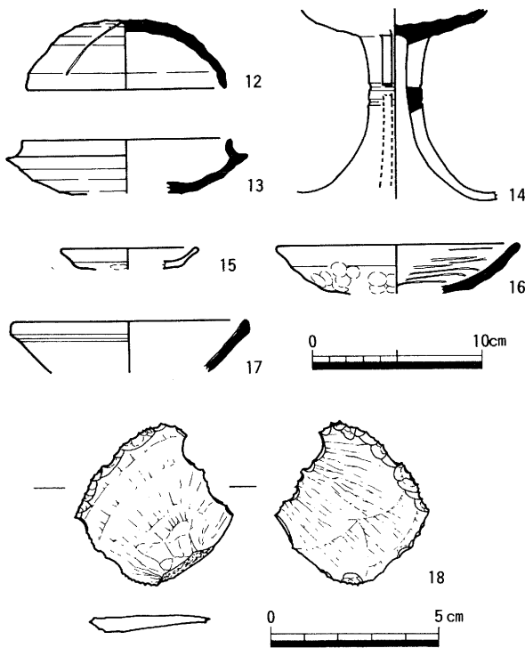
第6図 包含層出土遺物実測図
