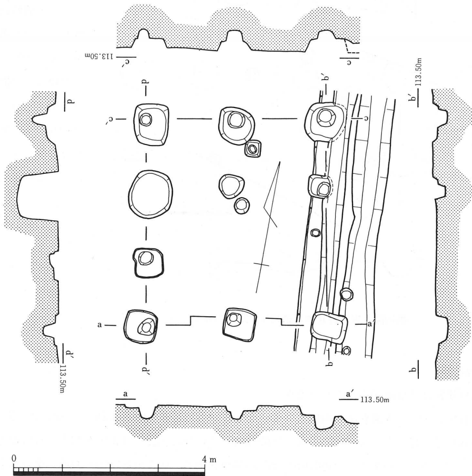
第8図 掘立柱建物1遺構実測図(1/80)
