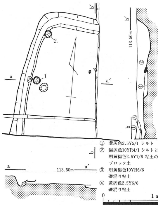
第11図 竪穴住居1 遺構実測図 (1/40)
