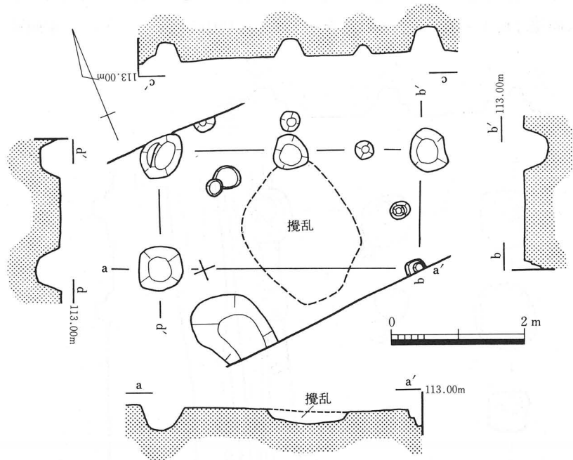
第10図 掘立柱建物3 遺構実測図 (1/80)
