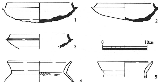
第12図 竪穴住居1 出土遺物実測図
