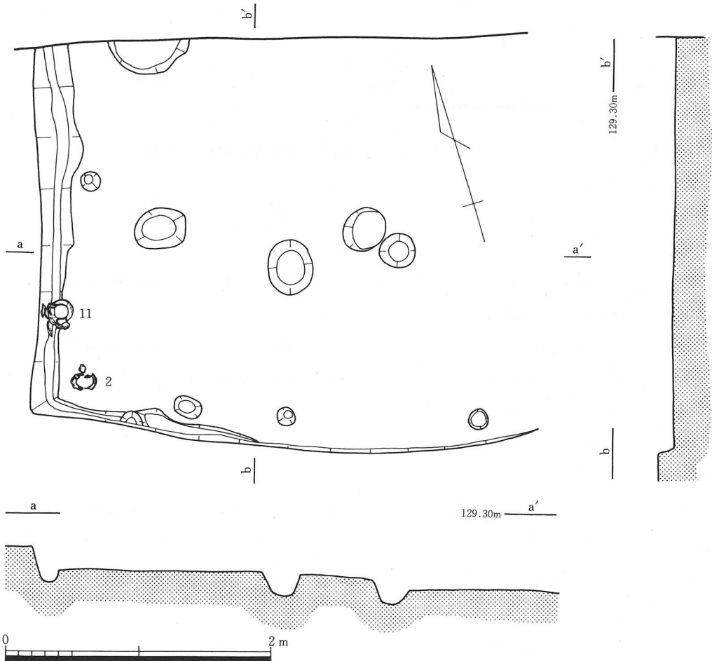
第3図 竪穴住居遺構実測図 (1/40)
