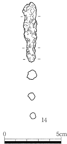
第6図 K S T 05-1 出土鉄器遺物実測 図(1/2)
