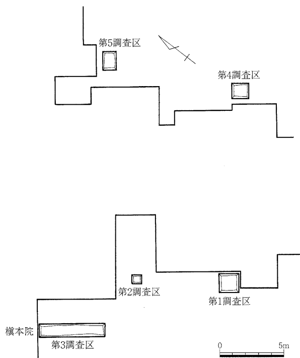
第7図 K S T06-1 調査区配置図 (1/300)
