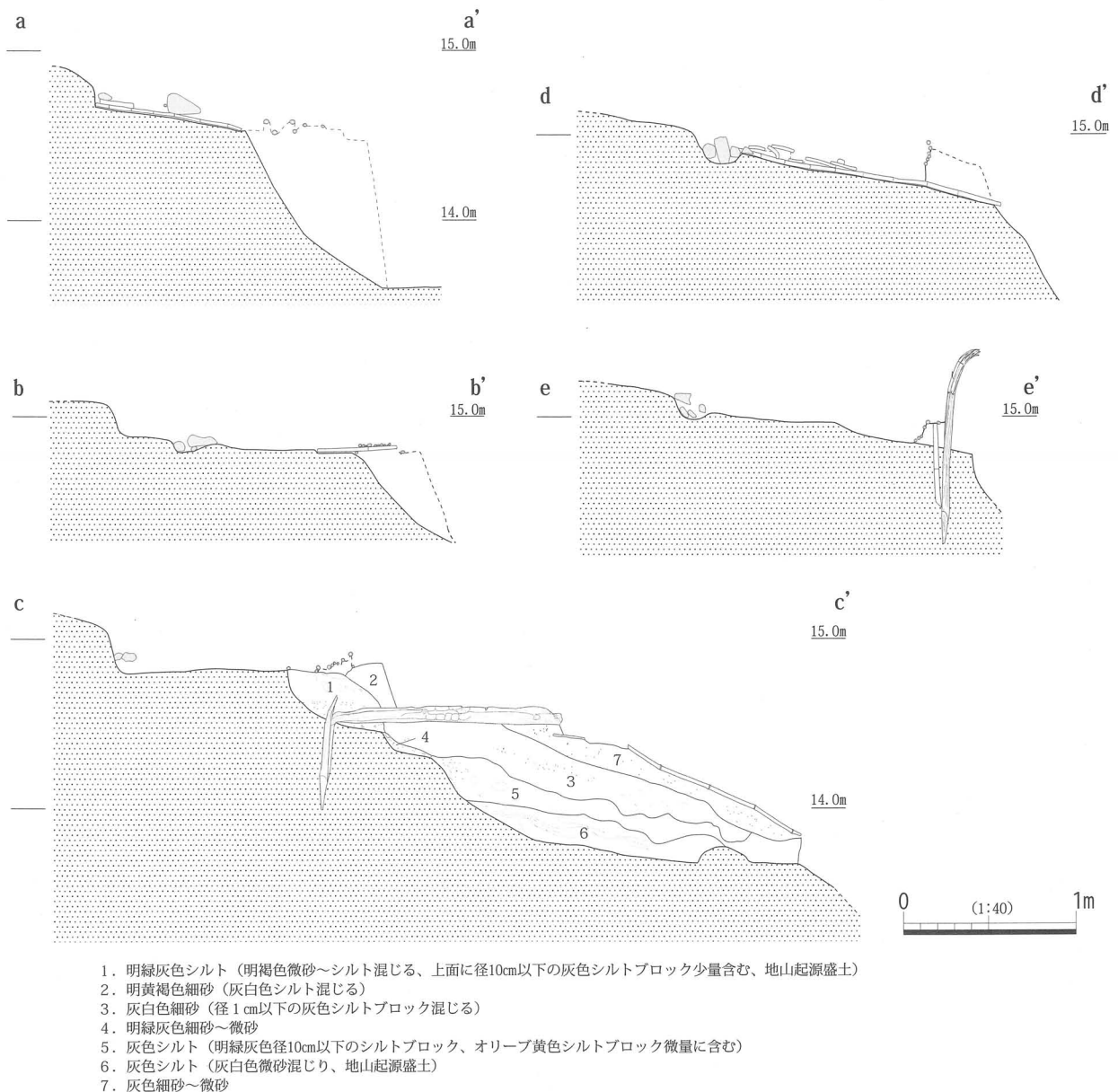
図 106 遺構 154 断面図
