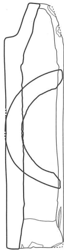
图 241 堀 83 出土丸瓦 (6)
