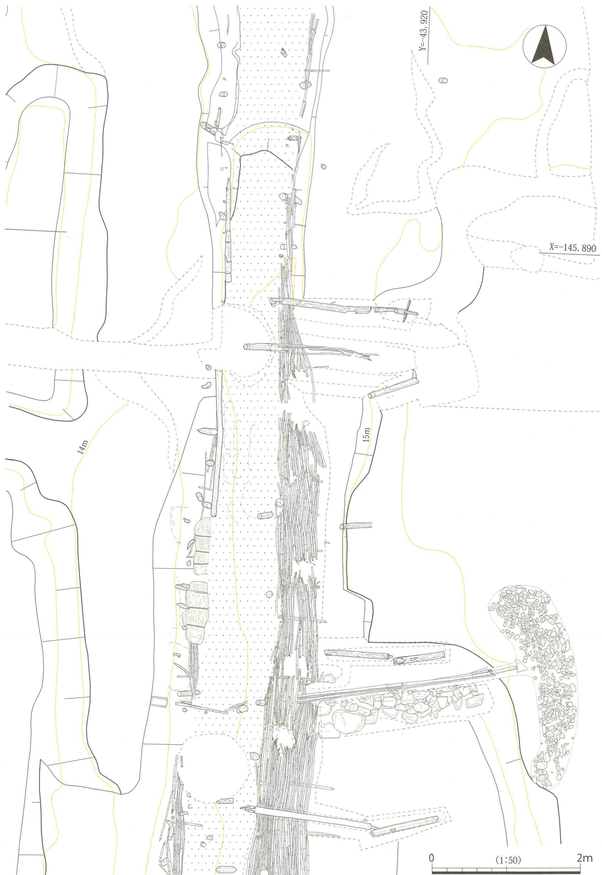
图 98 遺構 141 (北半)
