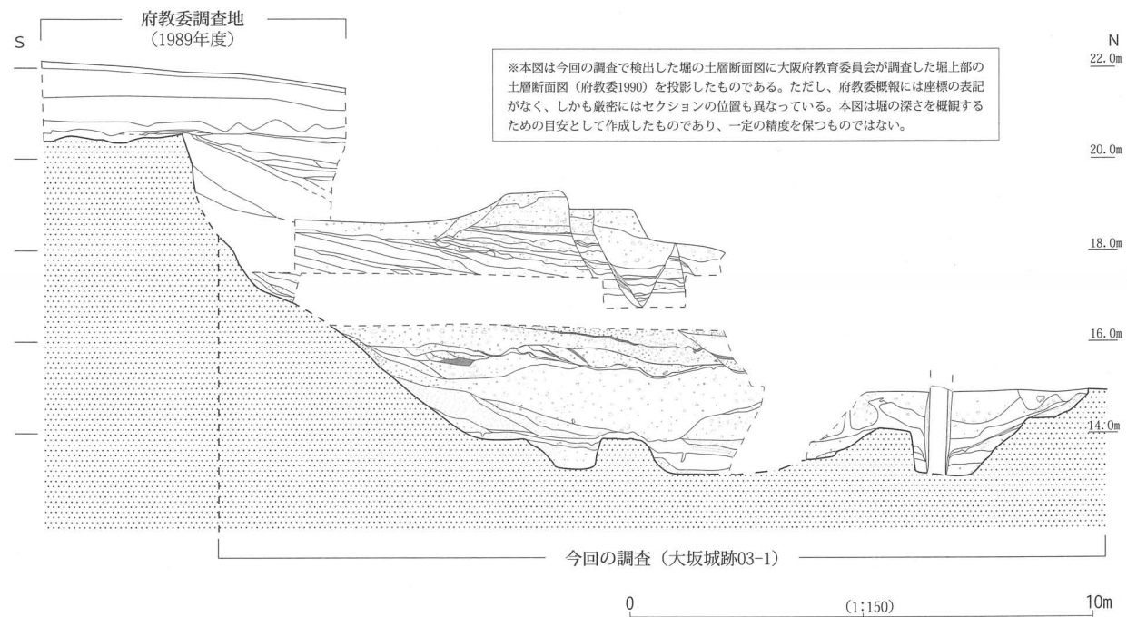
図 111 堀 83 断面図（3）
