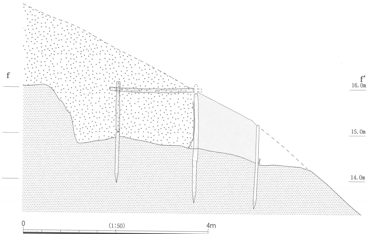
図 102 遺構 141 復元断面図
