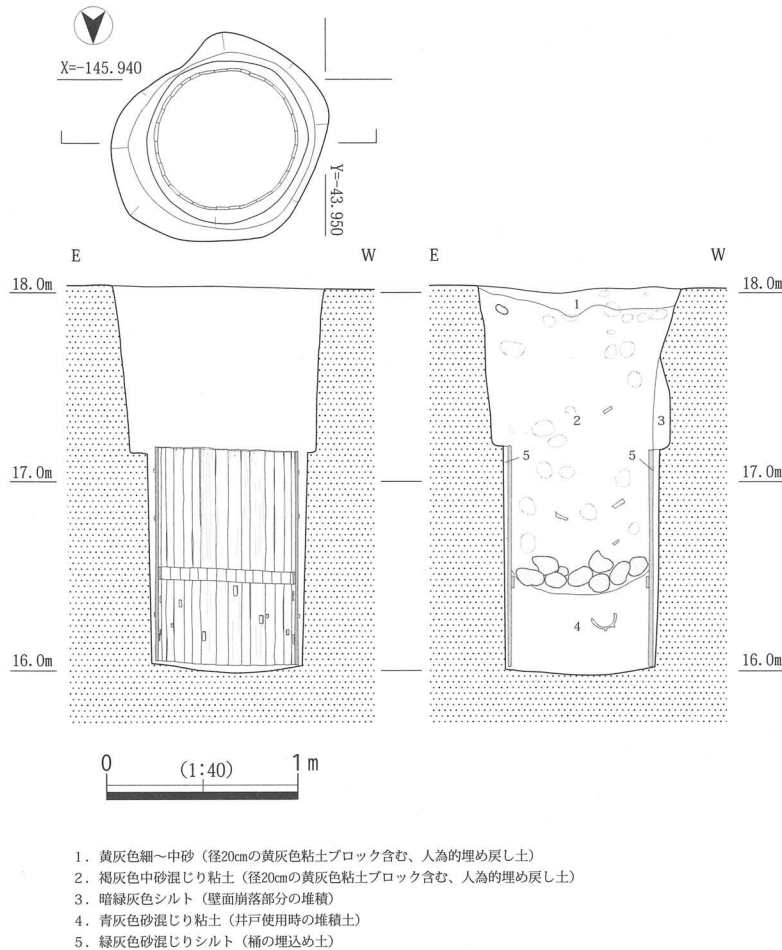
図 132 井戸 88
