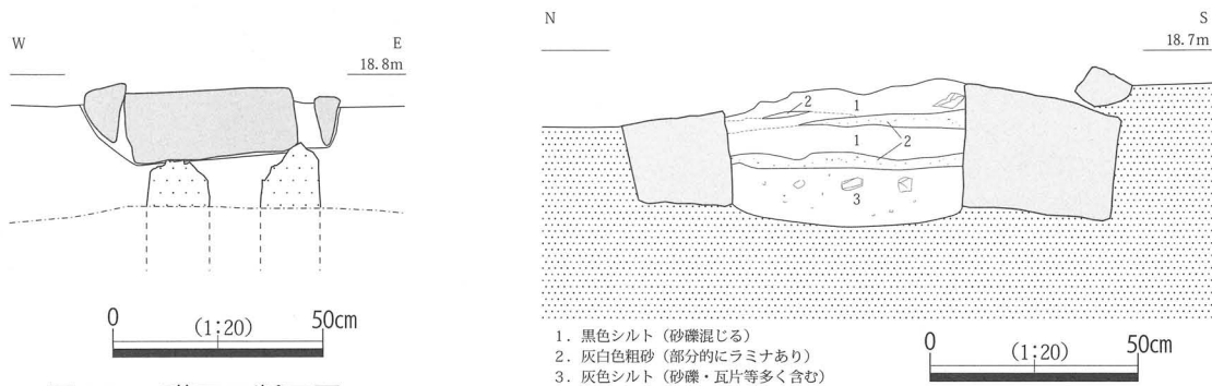
図 298 礎石7断面図
