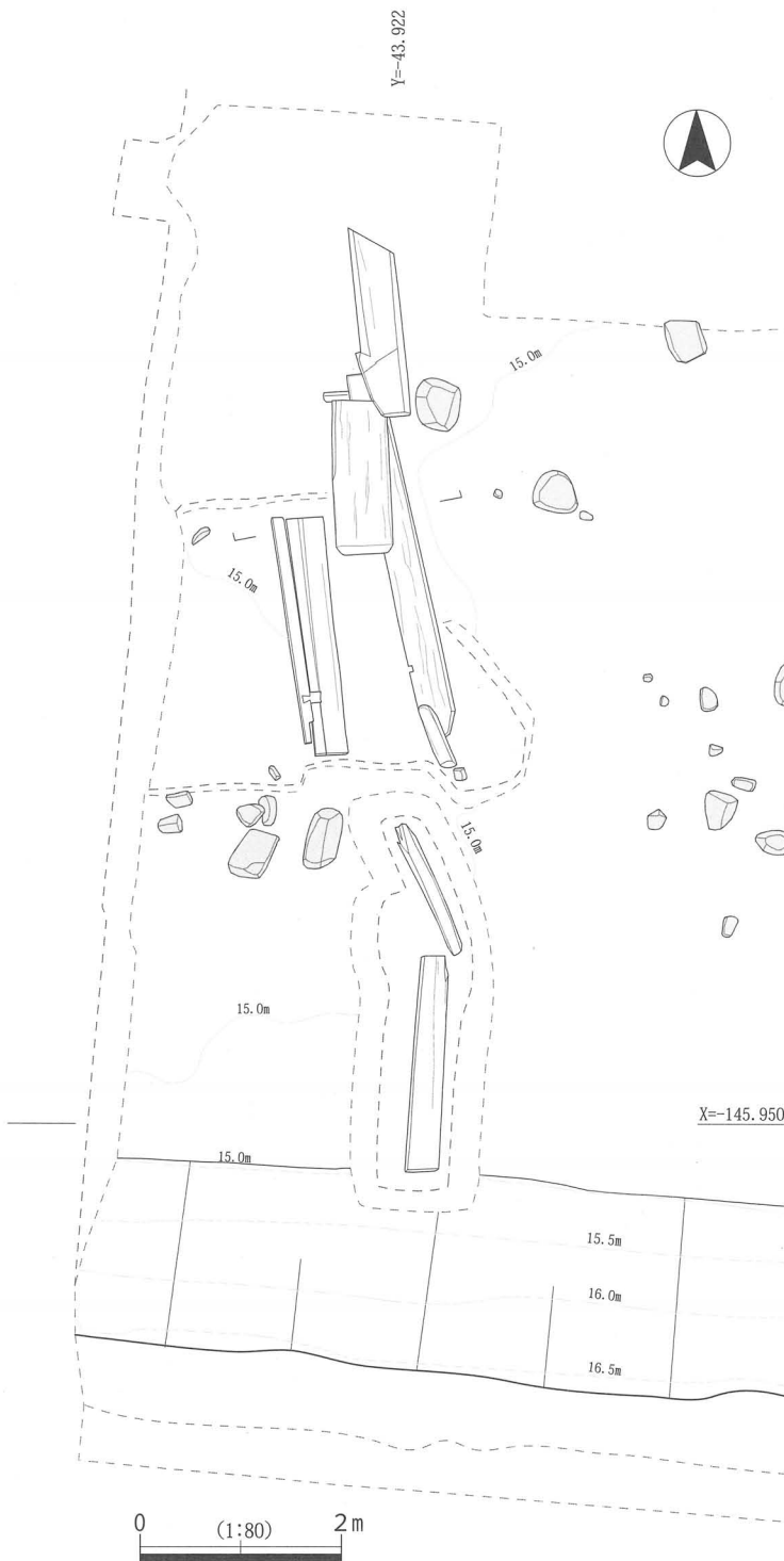
図 121 足場状遺構 114
