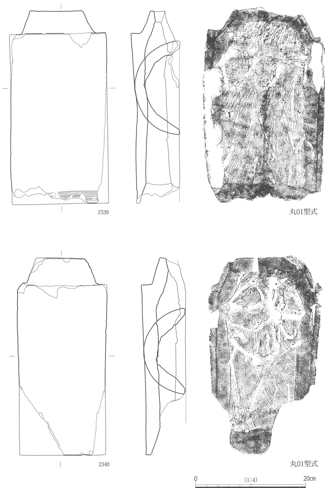
図 236 堀 83 出土丸瓦 (1)
