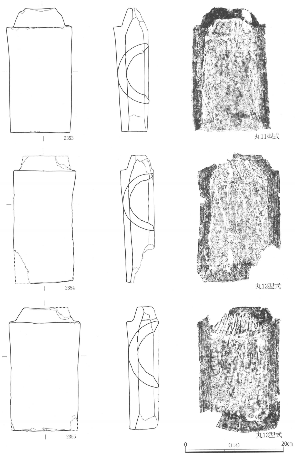
図 242 堀 83 出土丸瓦 (7)
