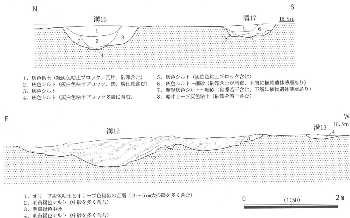
図 271 溝12・溝13・溝16・溝17断面図
