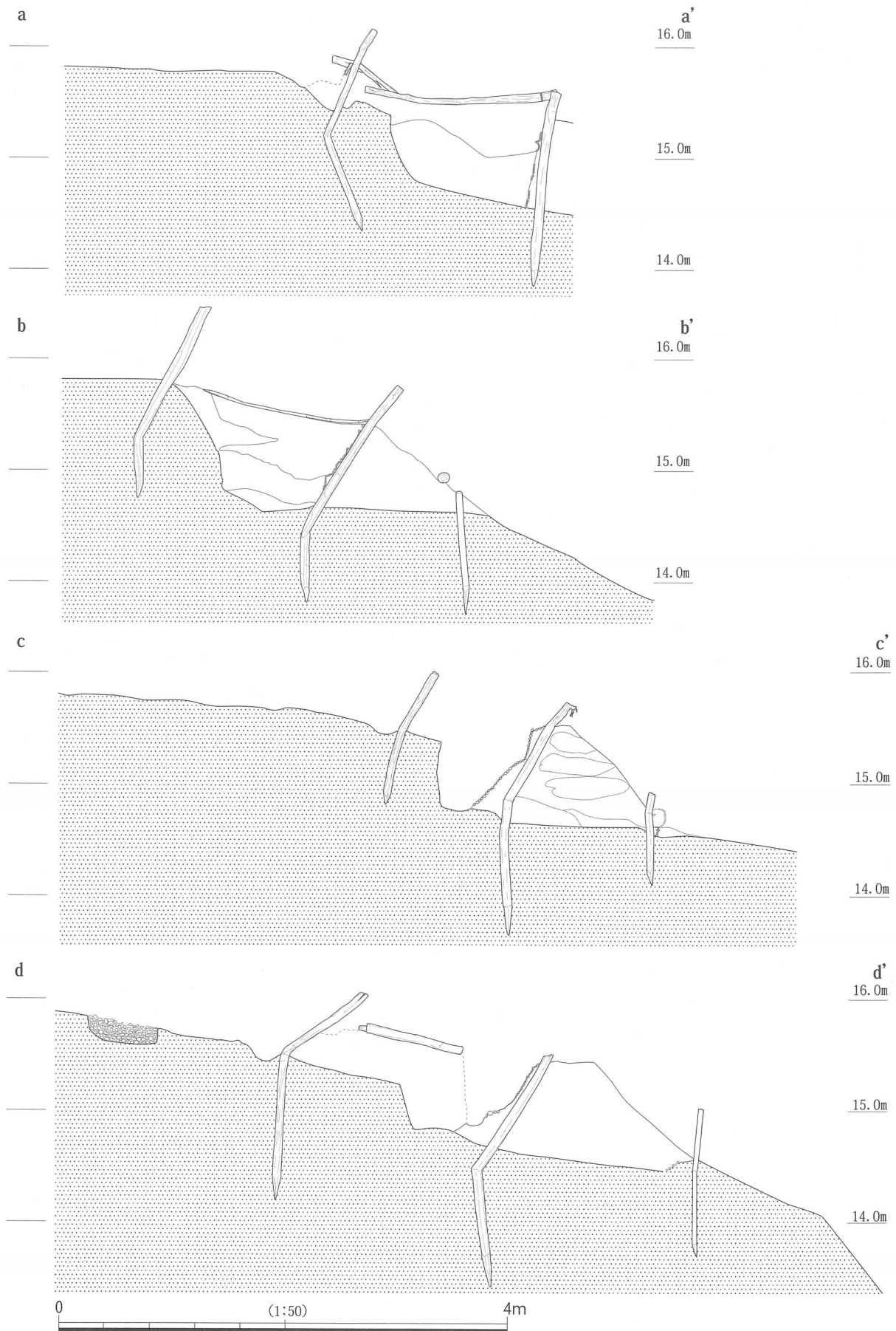
图 100 遺構 141 断面图 (1)
