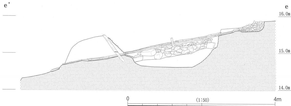
図 103 遺構 141 暗渠立面図
