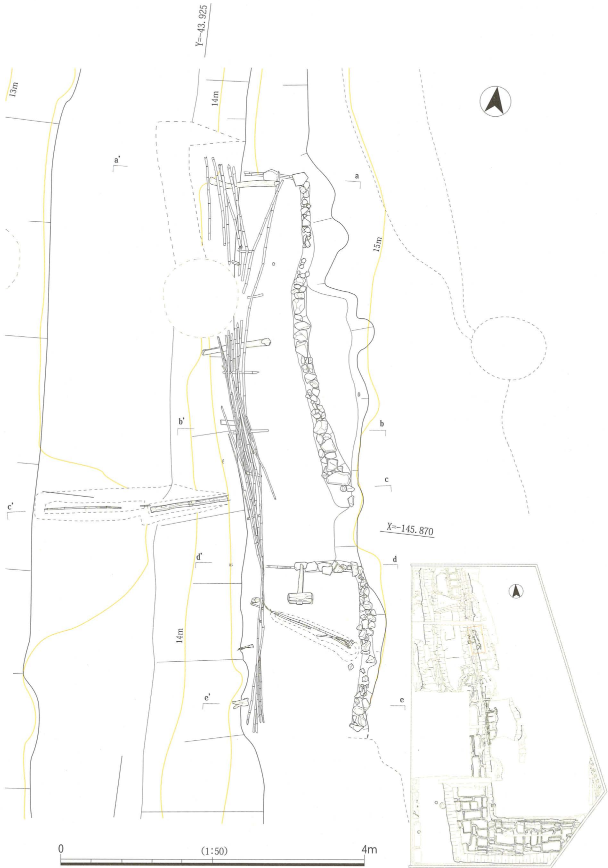
図 105 遺構 154
