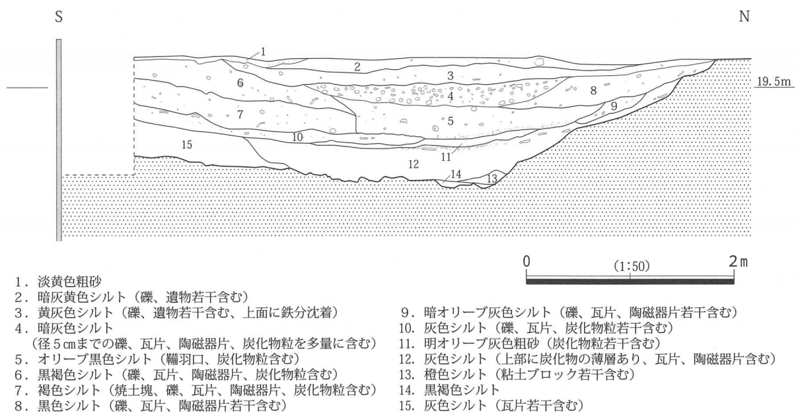
図274 土坑5断面図
