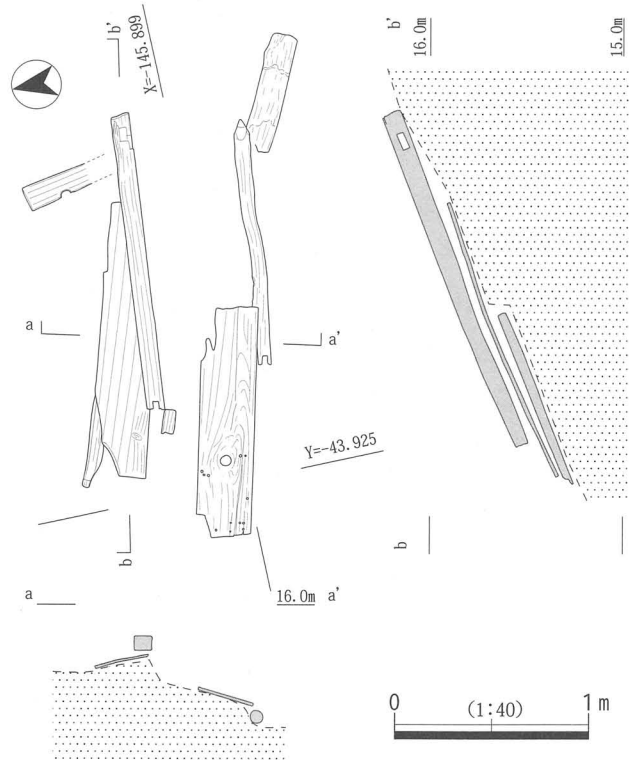
図 117 足場状遺構 98
