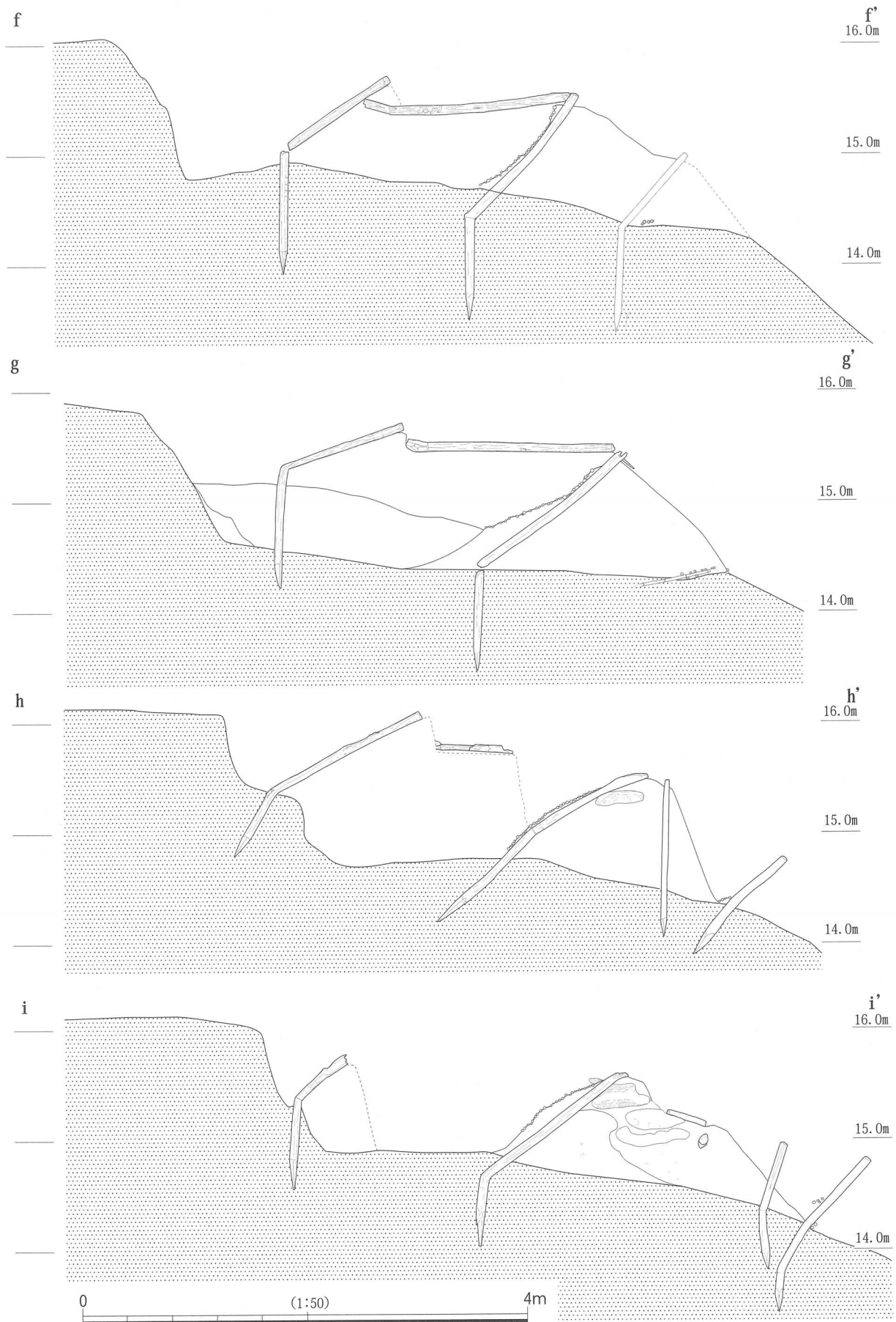
図 101 遺構 141 断面図 (2)
