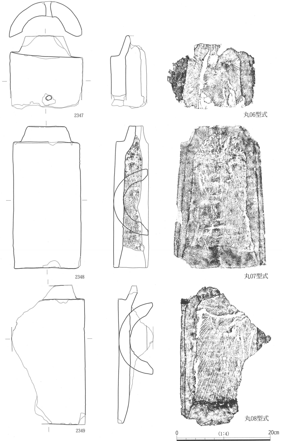
図240 堀83出土丸瓦(5)
