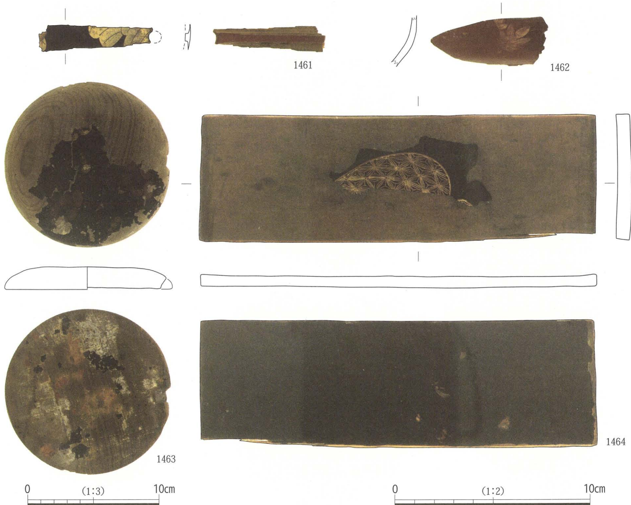
図 165 堀 83 出土漆器 (4)
