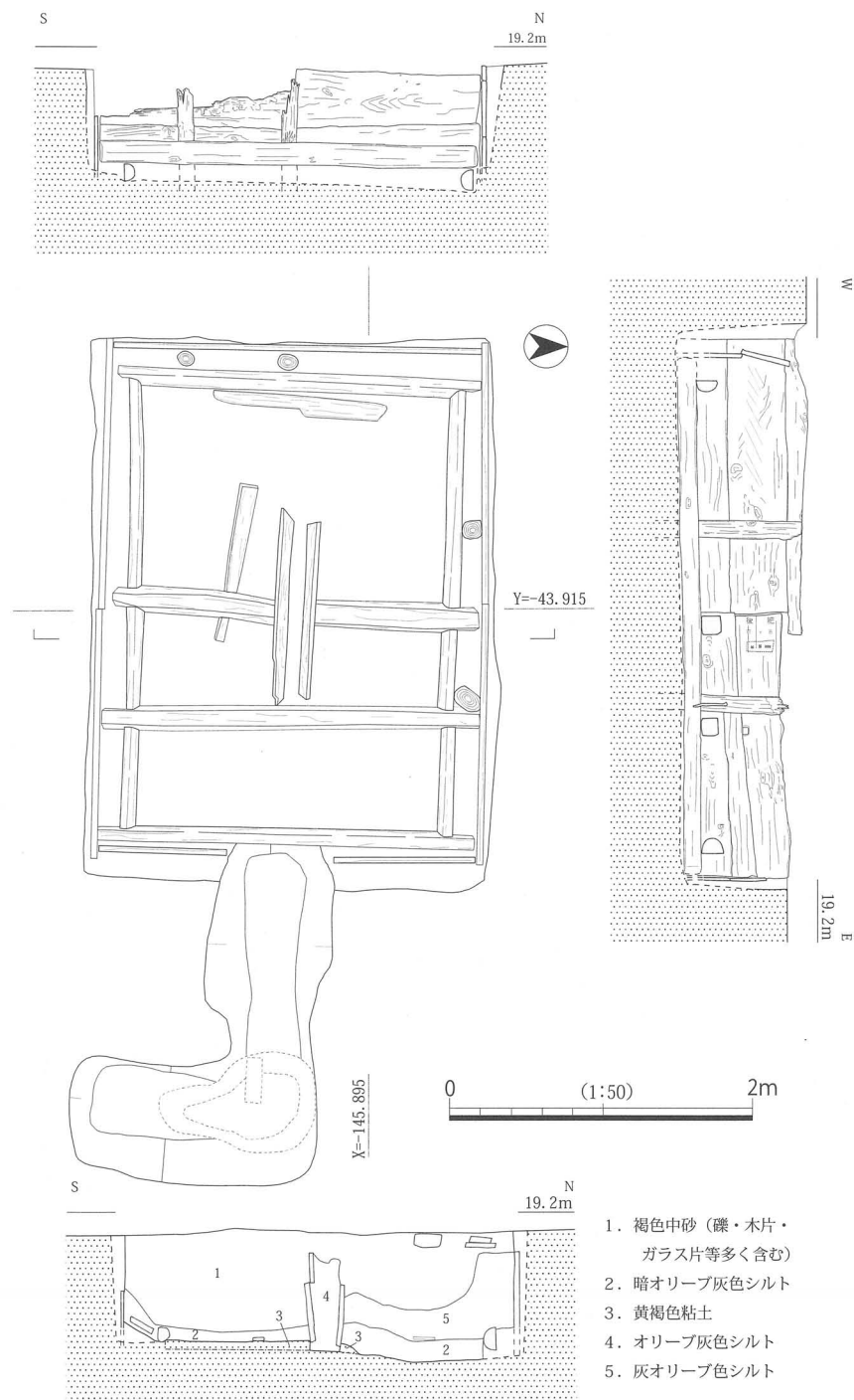
図 302 防空壕 32
