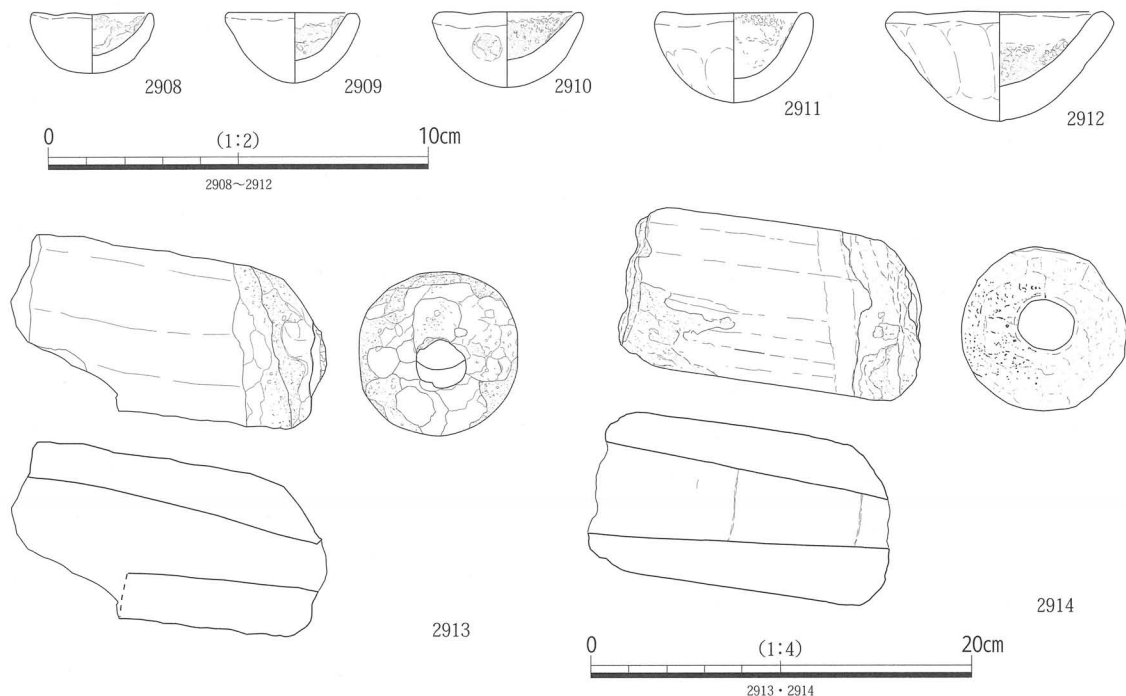
図 289 土坑 5 出土トリベ・鞆羽口
