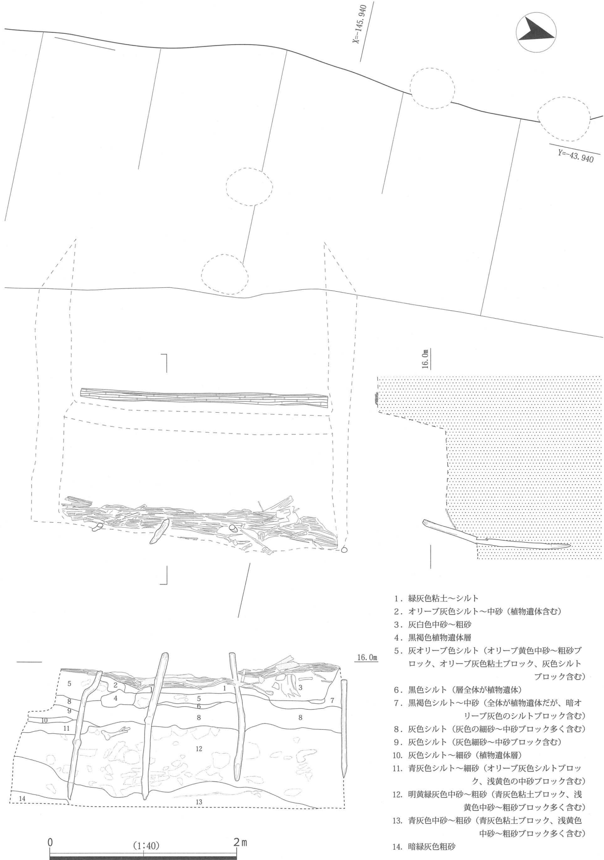
図 120 足場状遺構 108
