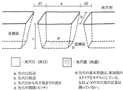
図18 矢穴模式図
