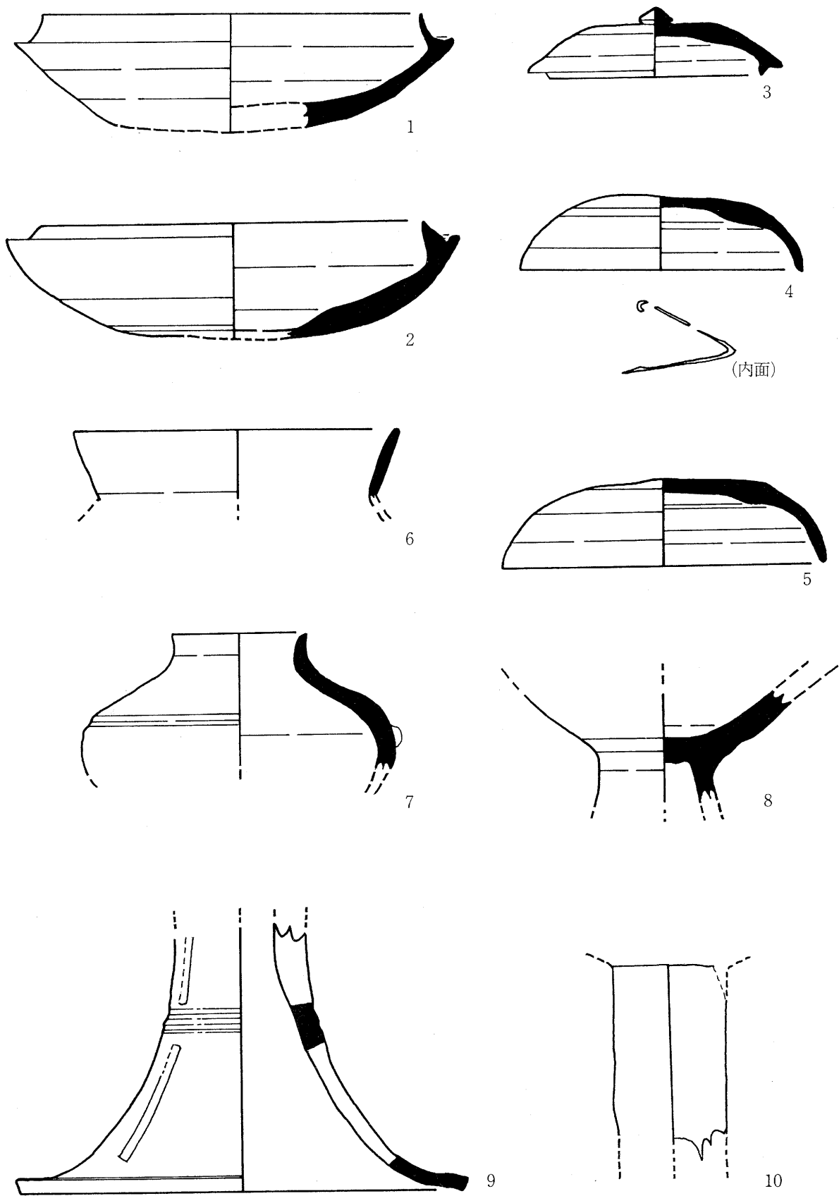
第12図 出土遺物実測図(1) (1:2)
