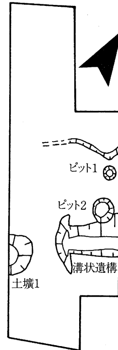
第6図 遺構平面図(1:100)
