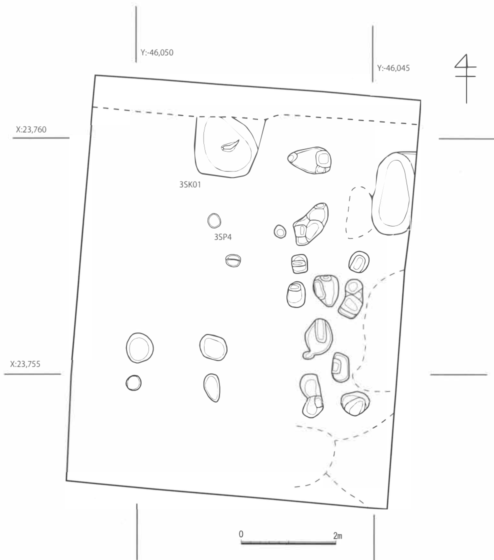
Fig.9 遺構全体図 (1/80)
