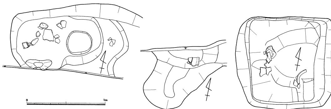
図6. 土壇2.9.8 遺物出土状況図
