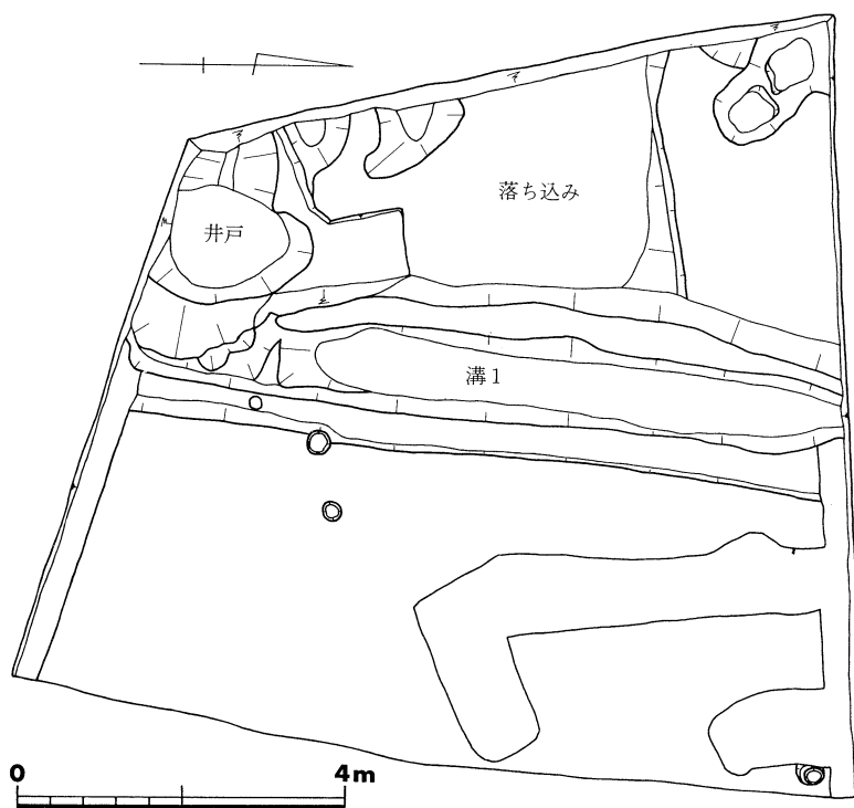
図10. 遺構平面図
