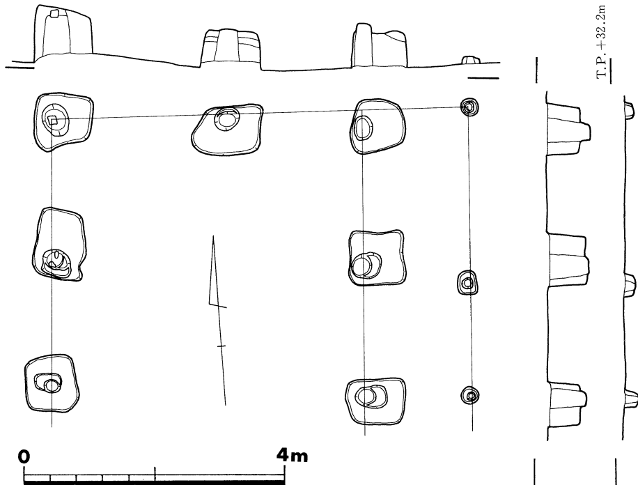
図12. 建物1 平面・断面図
