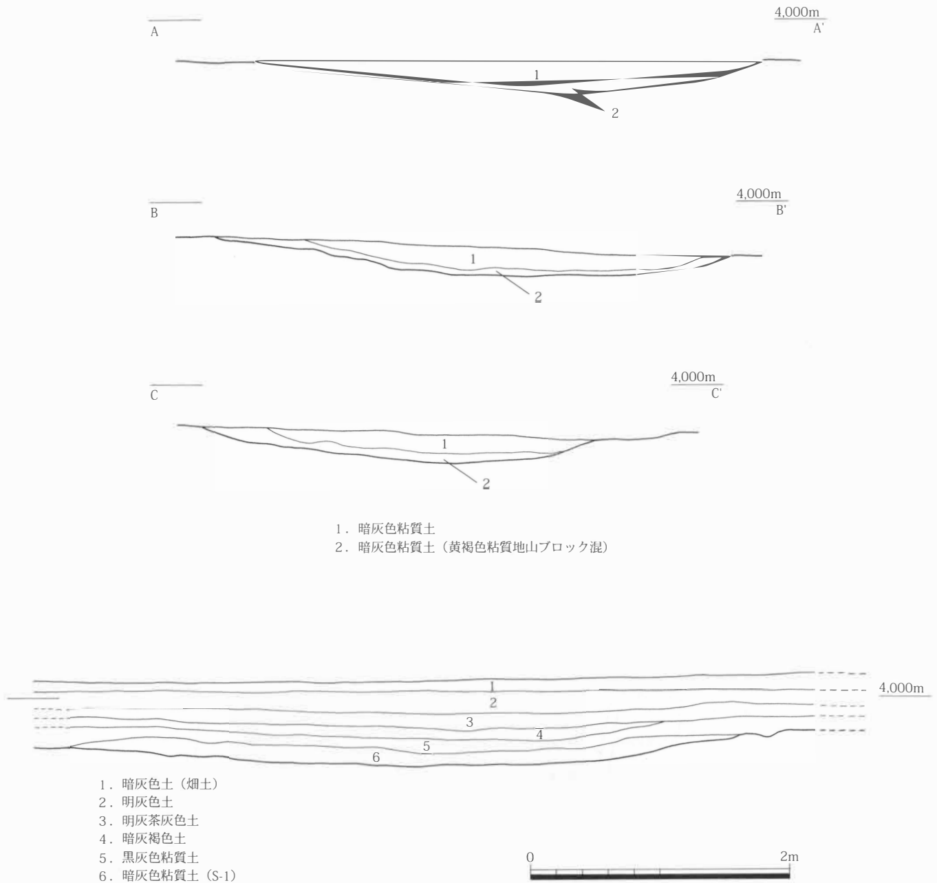
Fig.3 SD01 土層図 (1/40)
