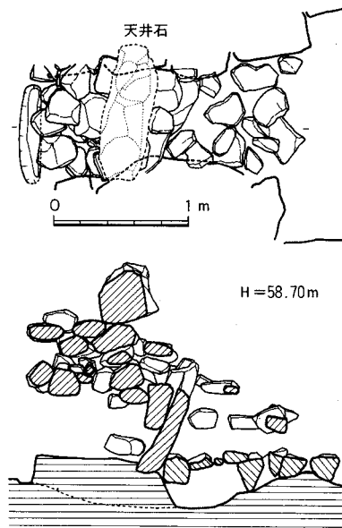
Fig. 9 C-2号墳閉塞施設実測図 (1/50)
