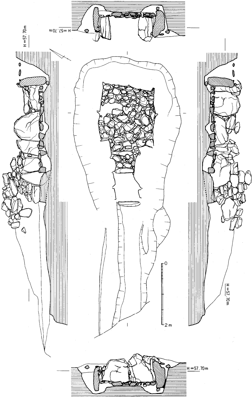
Fig. 7 C-2号填石室实测图 (1/60)
