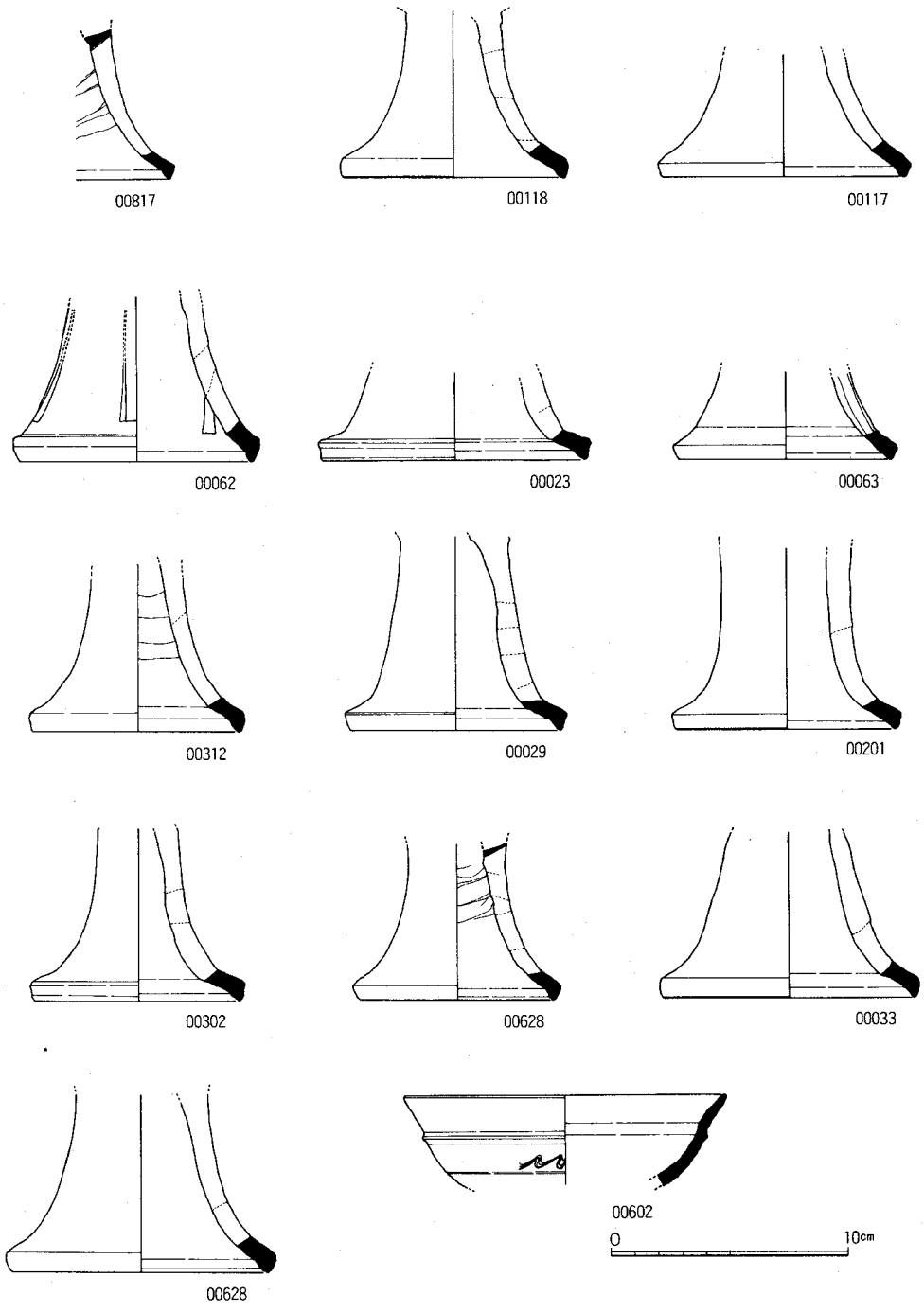
Fig. 18 窯址出土遺物実測図(2)(1/3)
