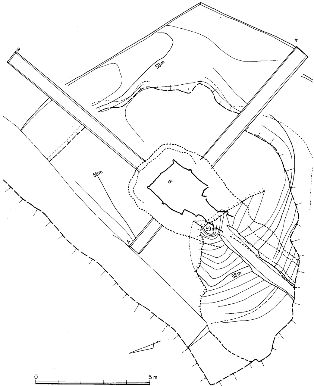
Fig. 5 C-2号墳墳丘遺存図 (1/100)
