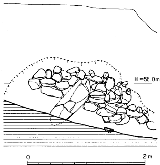
Fig. 15 窯体右壁面補強状況側面図 (1/40)
