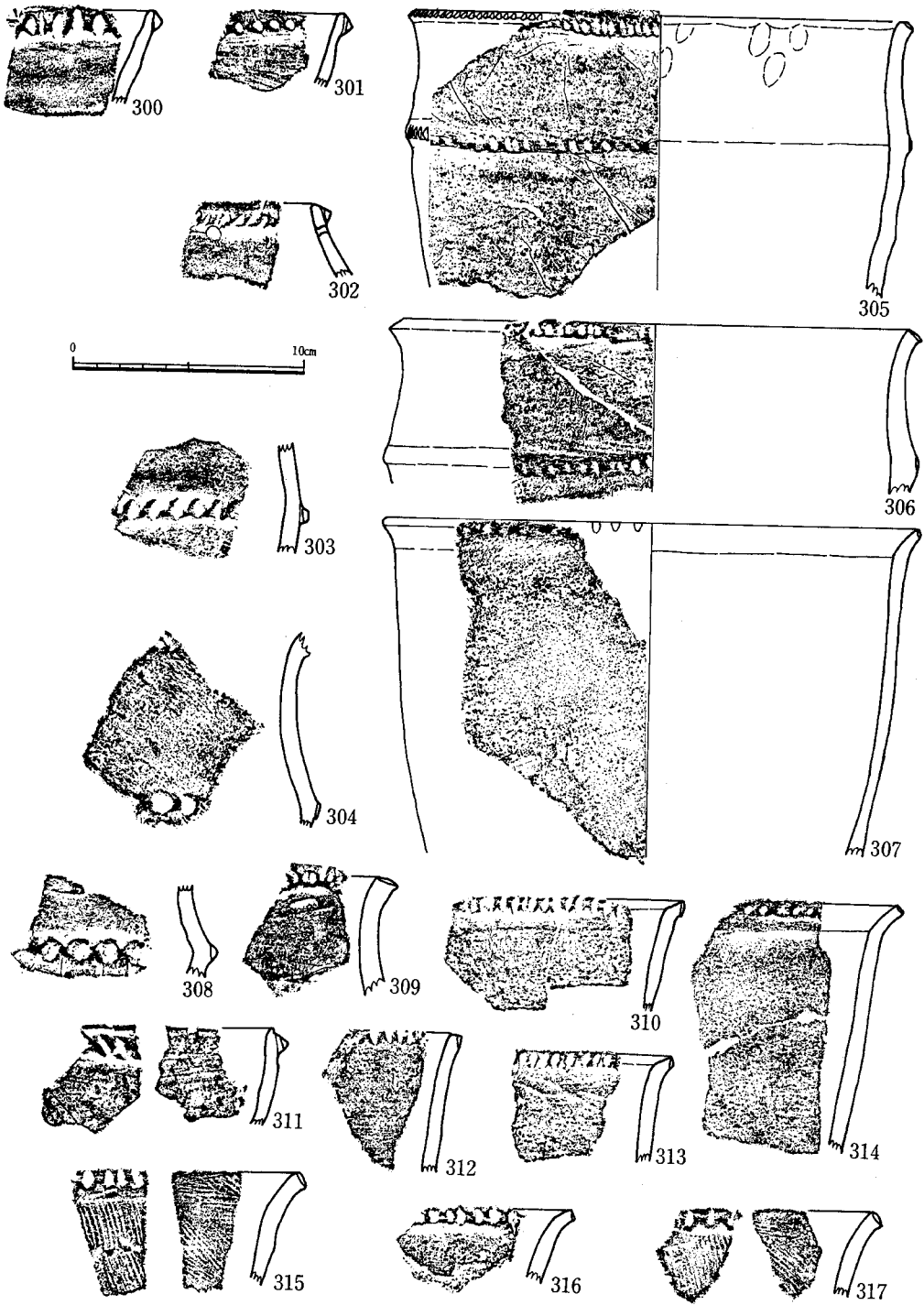
Fig.49 遺物実測図 XVIII
