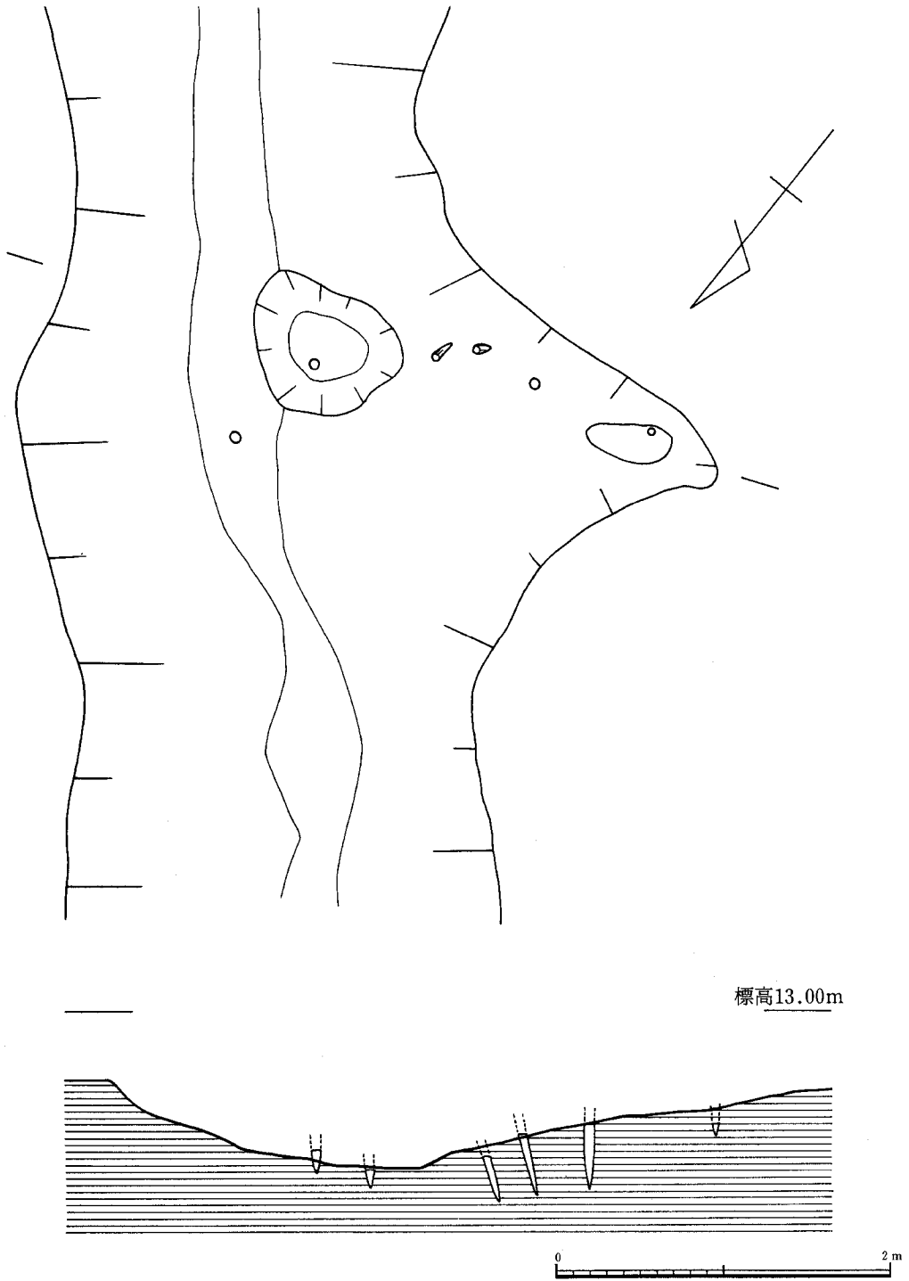
Fig.23 2号井堰・水口3実測図
