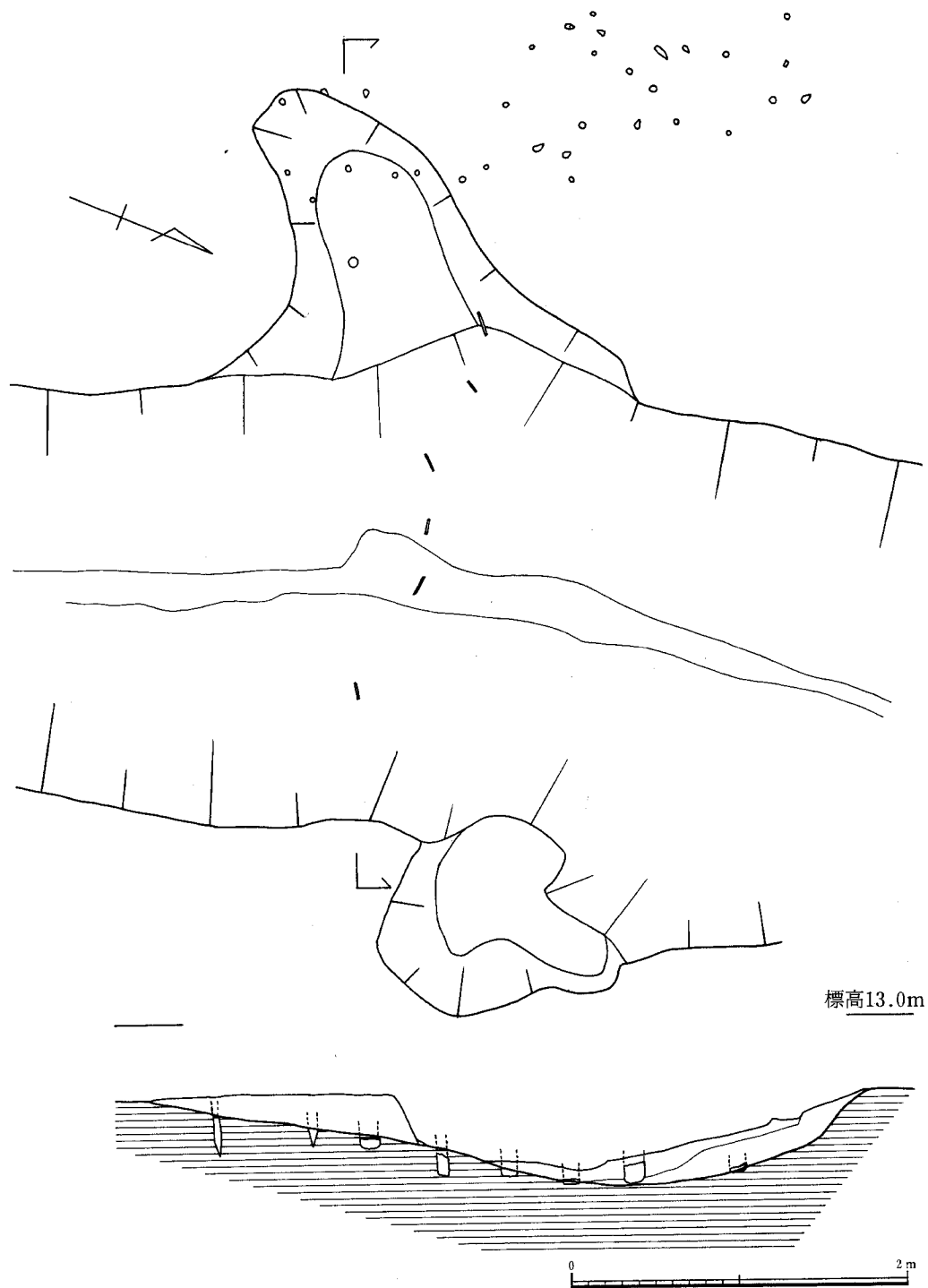
Fig.24 3号井堰・水口4.5実測図
