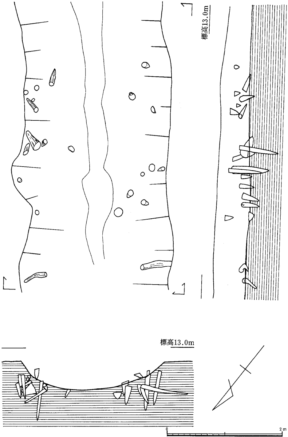
Fig.22 1号井堰実測図
