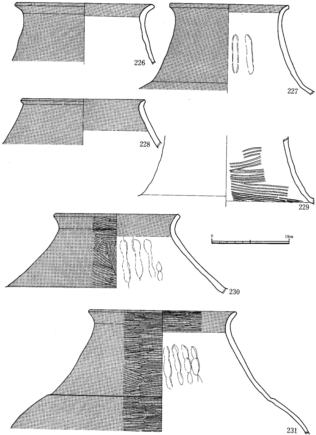
Fig.44 遺物実測図 XIII
