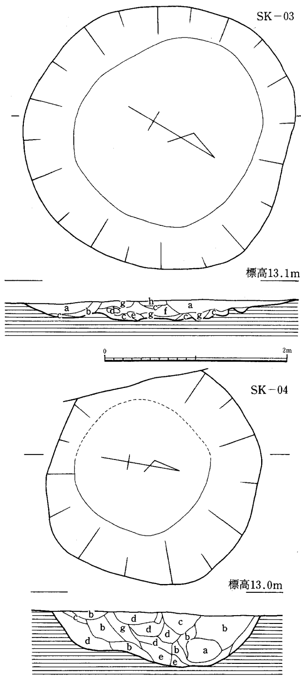
Fig.29 土坑(SK-03, 04)実測図
