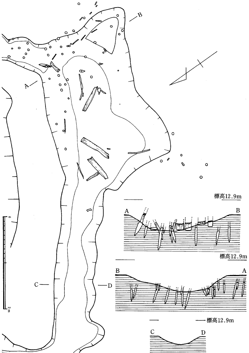
Fig.19 SD-03 実測図
