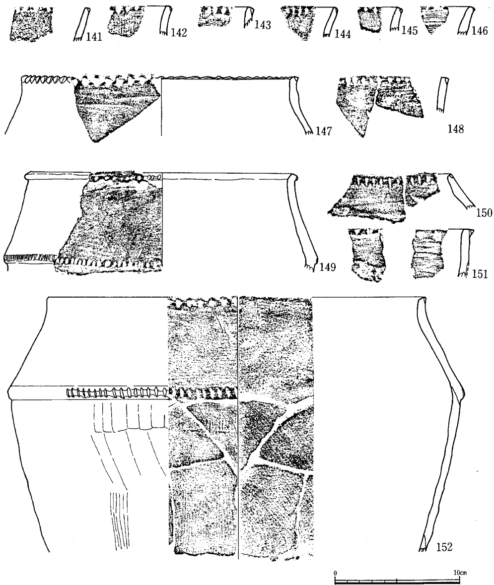
Fig.38 遺物実測図Ⅶ
