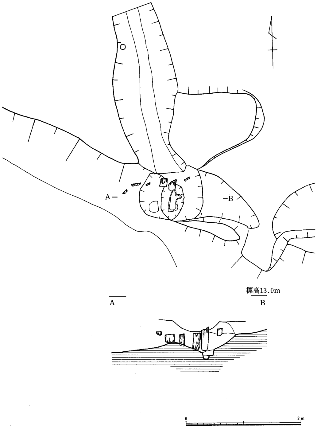
Fig.20 支線水路(SD-04)・堰実測図
