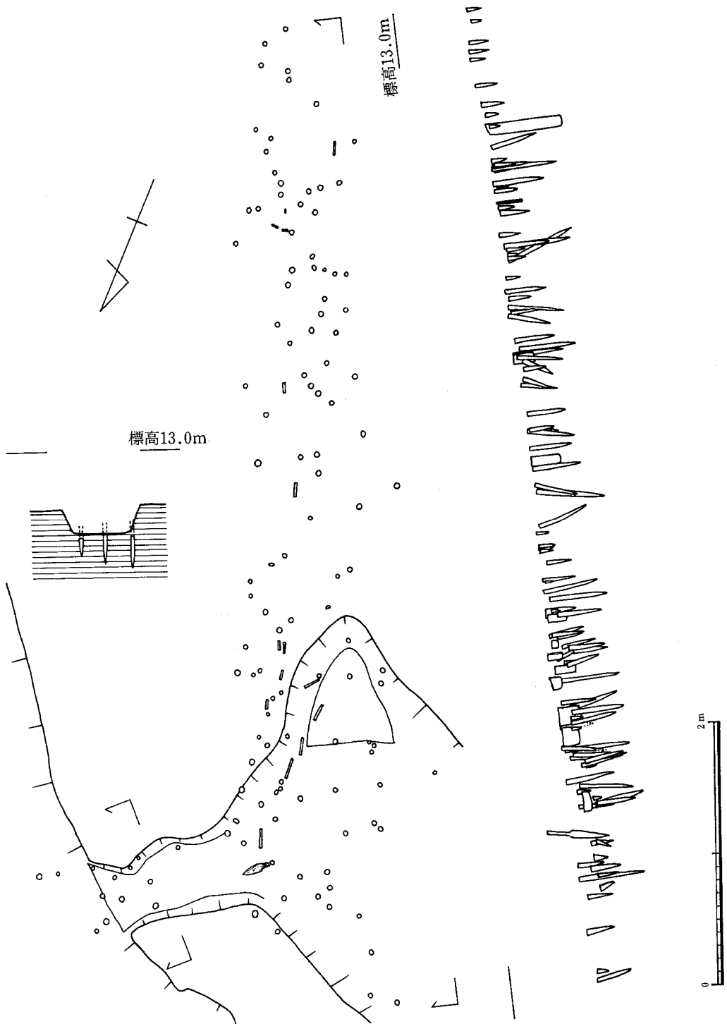
Fig.27 水口7実測図
