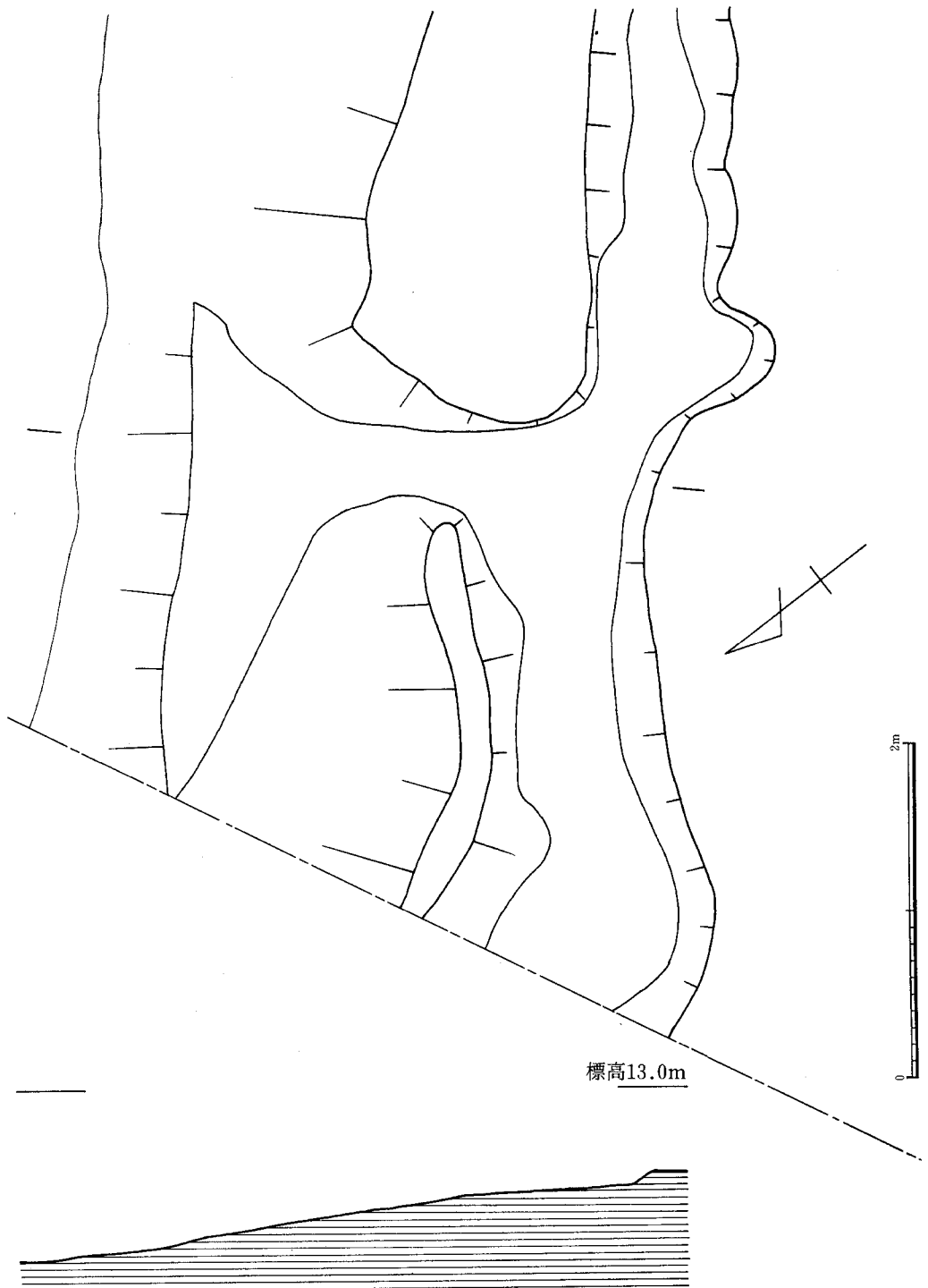
Fig.28 水口8実測図
