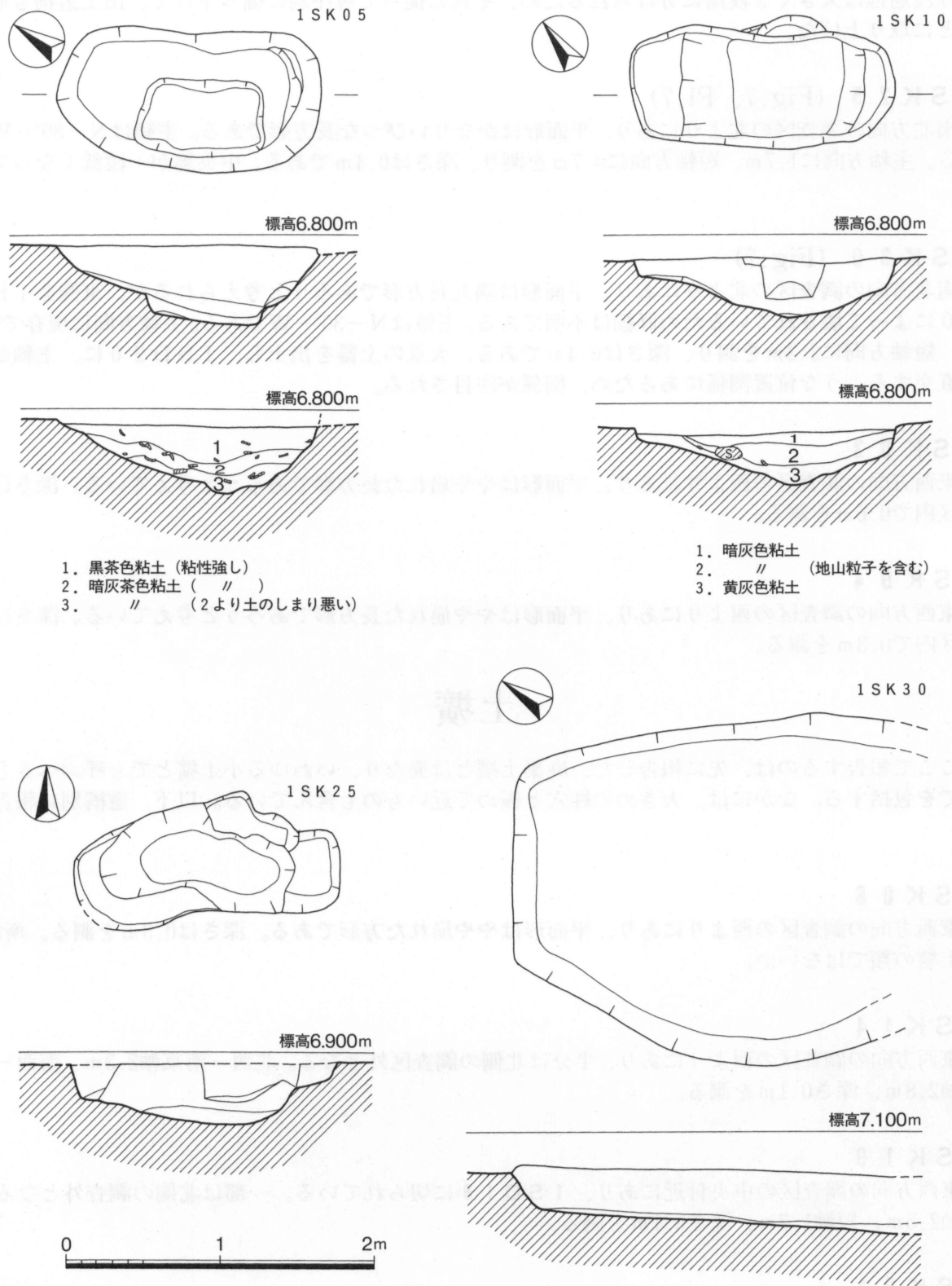
Fig.7 廃棄土壌実測図 (1/40)
