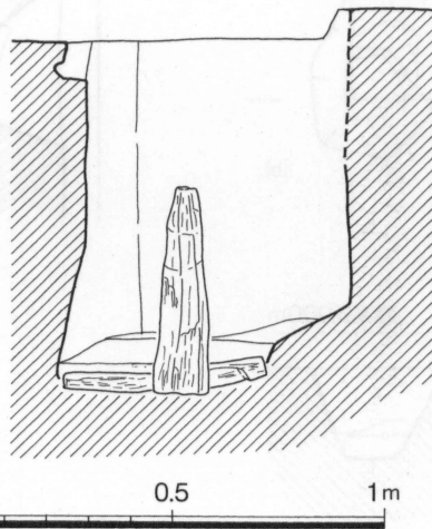
Fig.6 1SB26(a)柱根出土状況実測図 (1/20)
