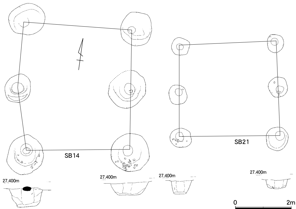
第7図 SB14・21平面図・断面図 (S=1/80)
