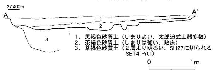
第6図 27号住居跡東西ベルト（S=1/50）
