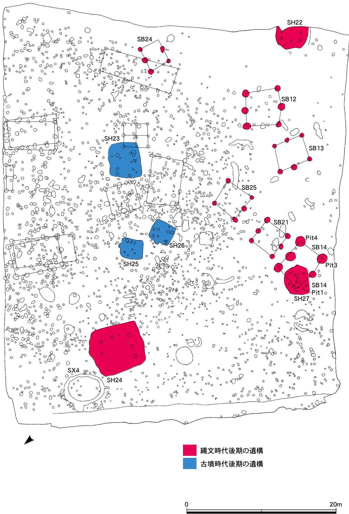
第5図 第5調査区遺構配置図 (S=1/300)
