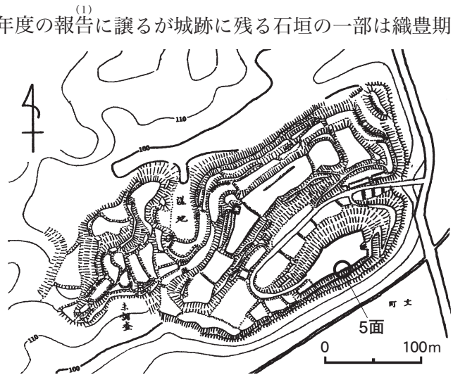
第28図 平田城跡縄張図（中村修身氏提供）
