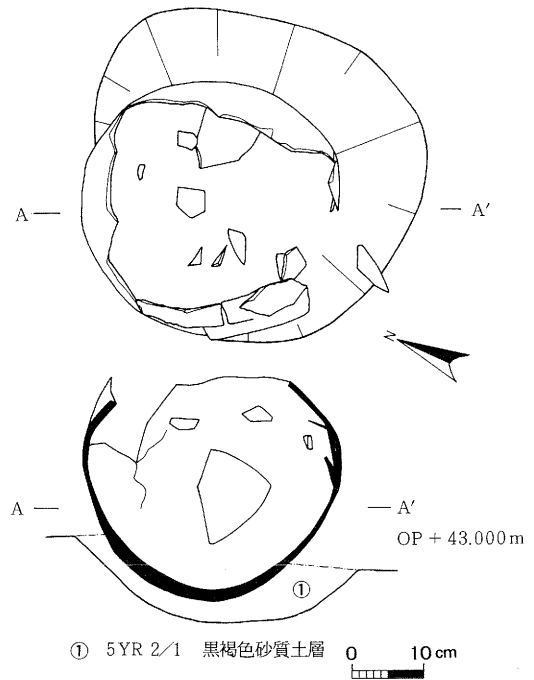
第14図 土壇54実測図
