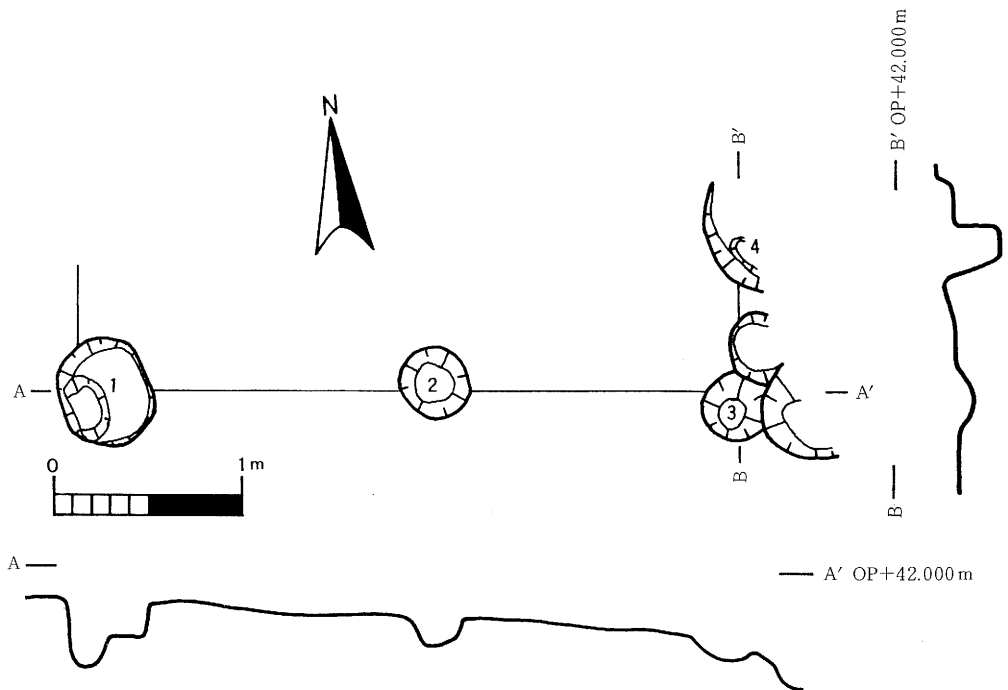
第8図 SB-01実測図
