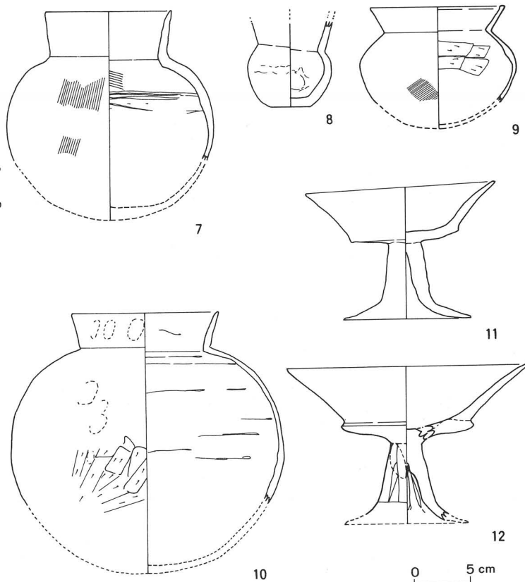
第17図 H-2区 遺物実測図
