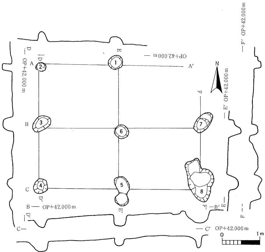
第9図 SB-02実測図
