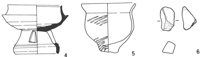
第16図 H-4区 遺物実測図
