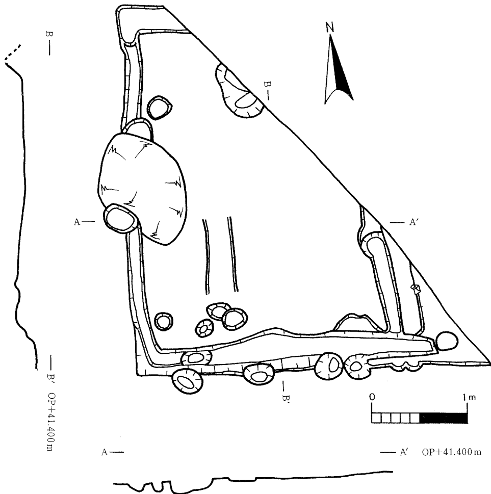
第12図 SH-03実測図
