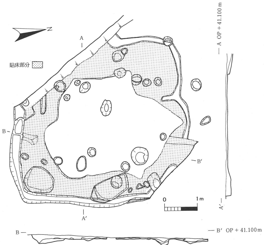
第10図 SH-01 実測図
