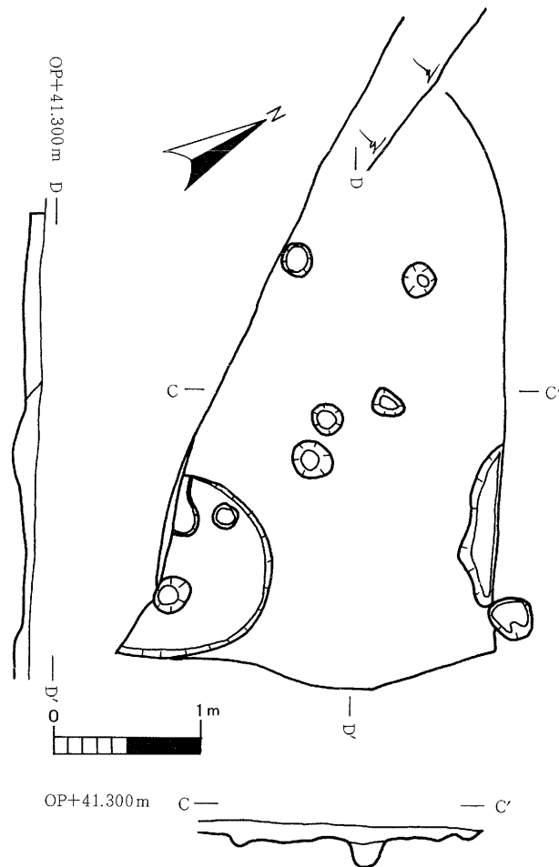
第11図 SH-02 実測図
