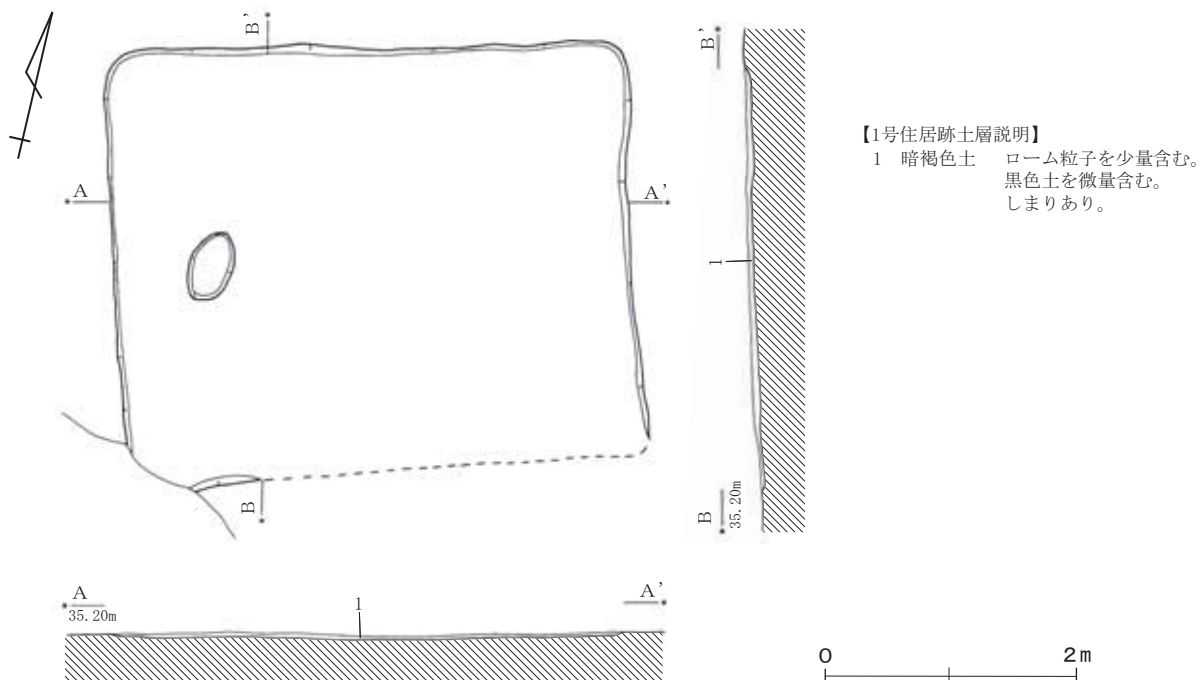
第4図 1号住居跡実測図
