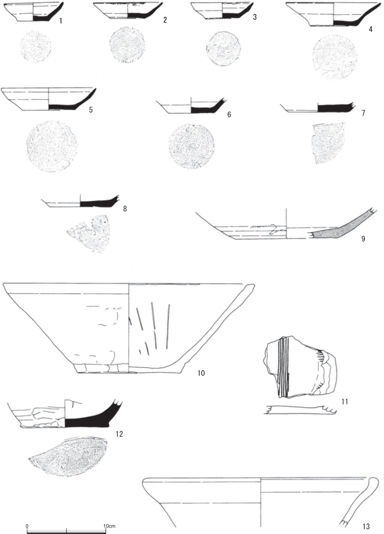
第15図 2号井戸跡出土遺物実測図(1)
