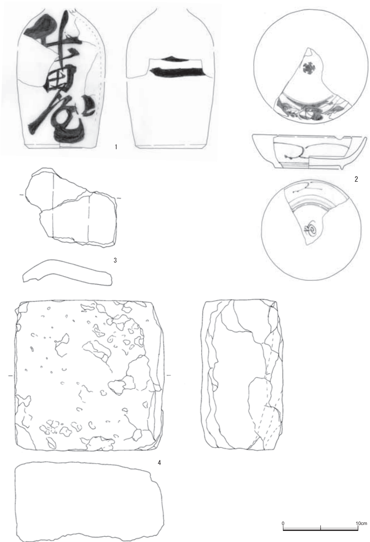
第30图 B区一括出土遺物実測図
