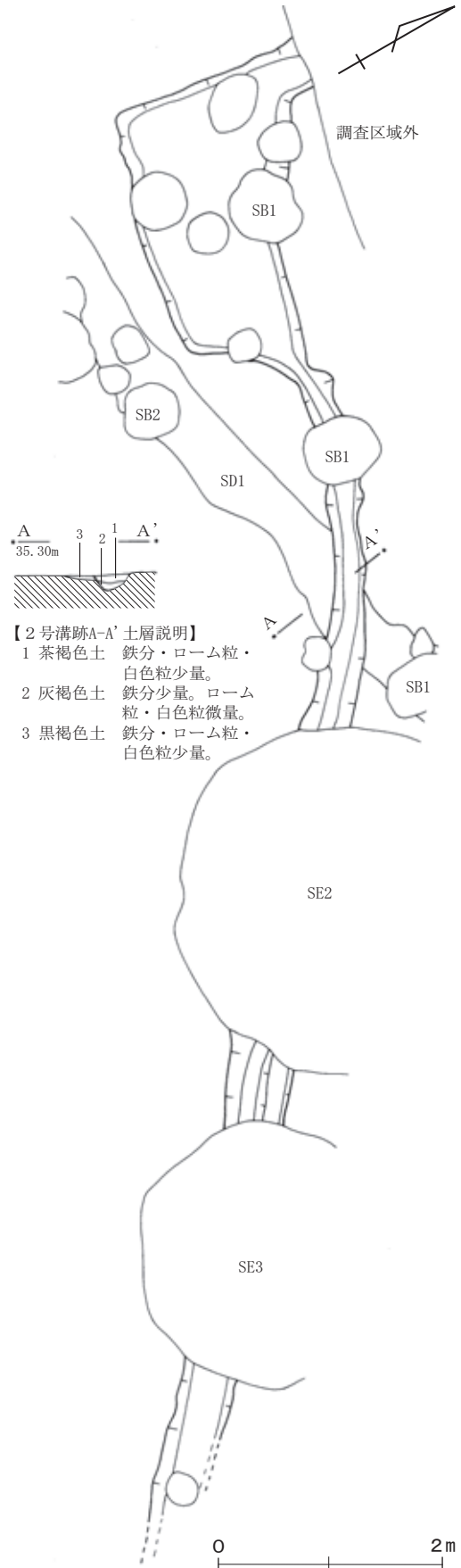
第29図 2号溝跡実測図
