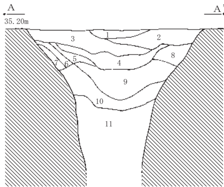
第9図 1号井戸跡実測図
