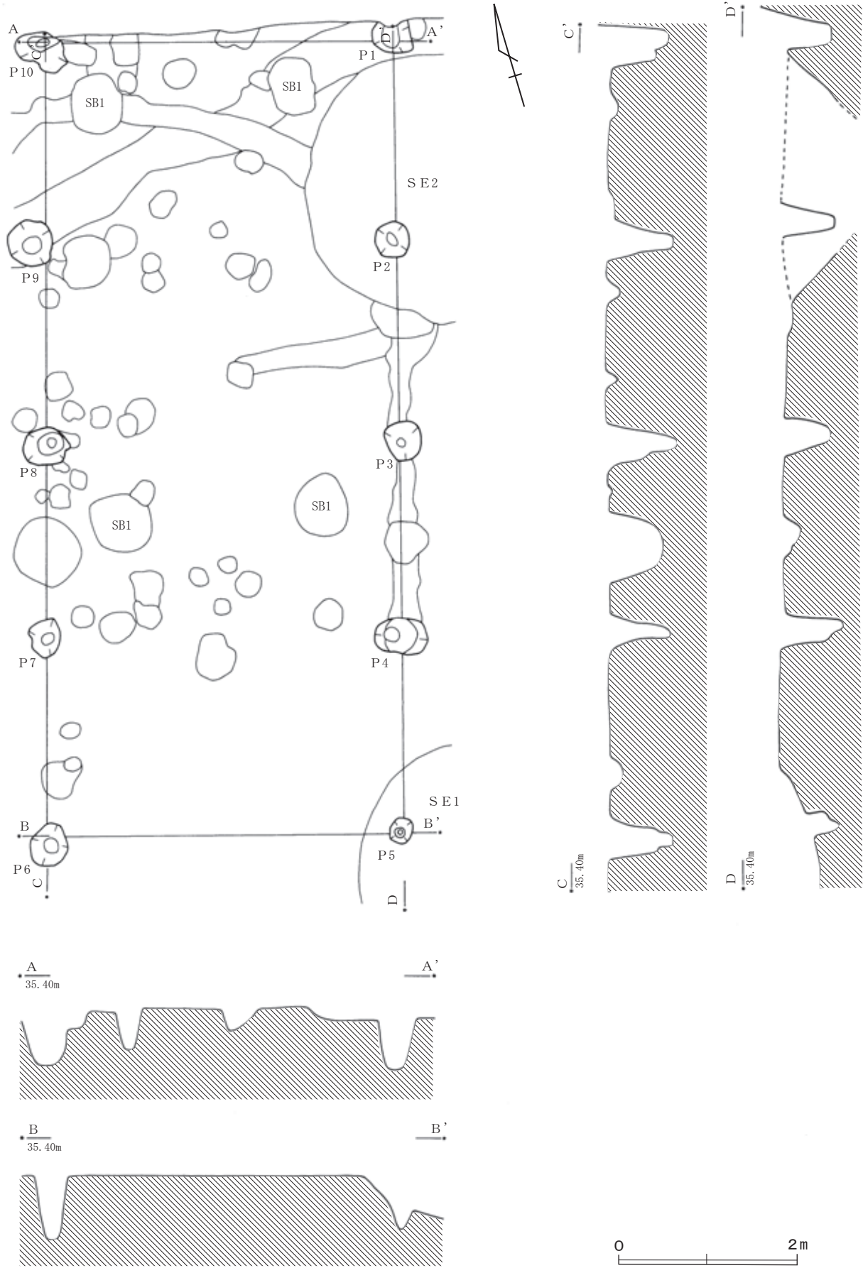
第8图 2号掘立柱建筑物迹实测图
