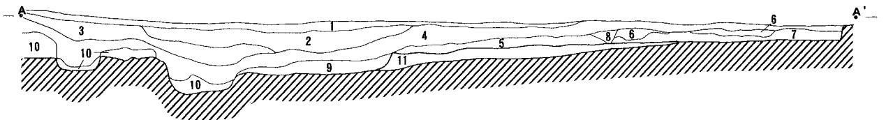
A-A' 土層断面
