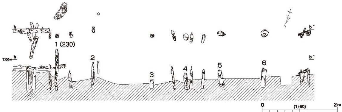
第23図 護岸施設詳細図
