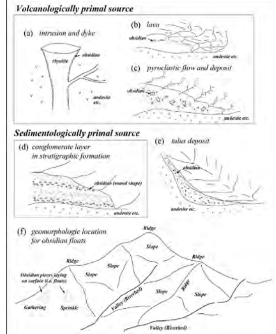
図4 黒曜石原産地の産状。(a) 火道，脈状の貫入岩，(b) 溶岩，(c) 火砕流堆積物，(d) 堆積性礫層，(e) 崖錐性堆積物，(f) 黒曜石転石の地形環境（斜面，尾根，河床）と，それらの散在の程度（集中，まばら）。
