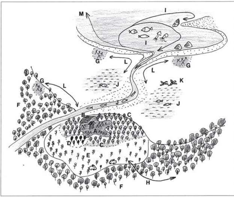
図5 縄文前期～中期の三内丸山集落生態系モデル (辻 2011)
