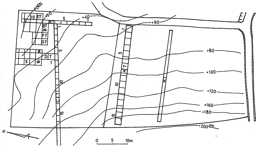
第5図 第2地区遺跡全体図
