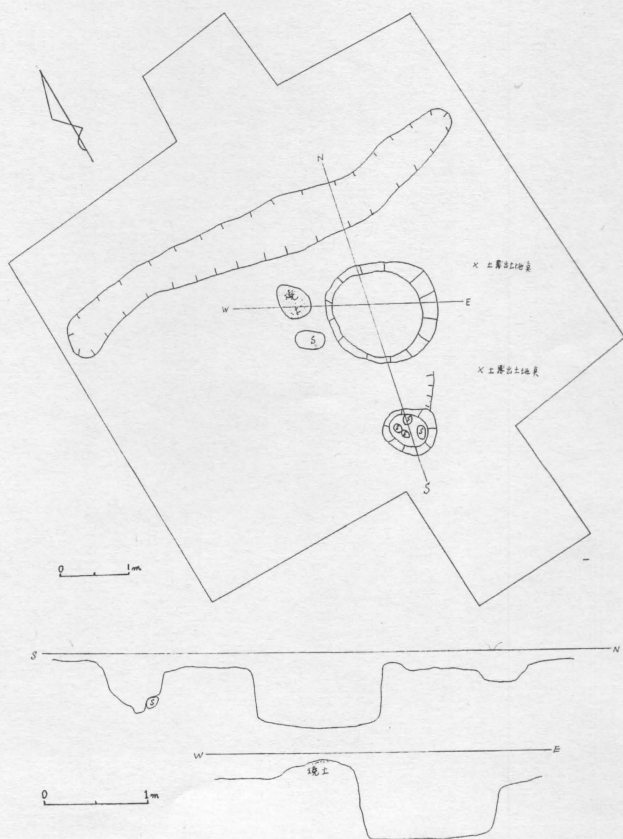
第4図 第I地区住居址実測図
