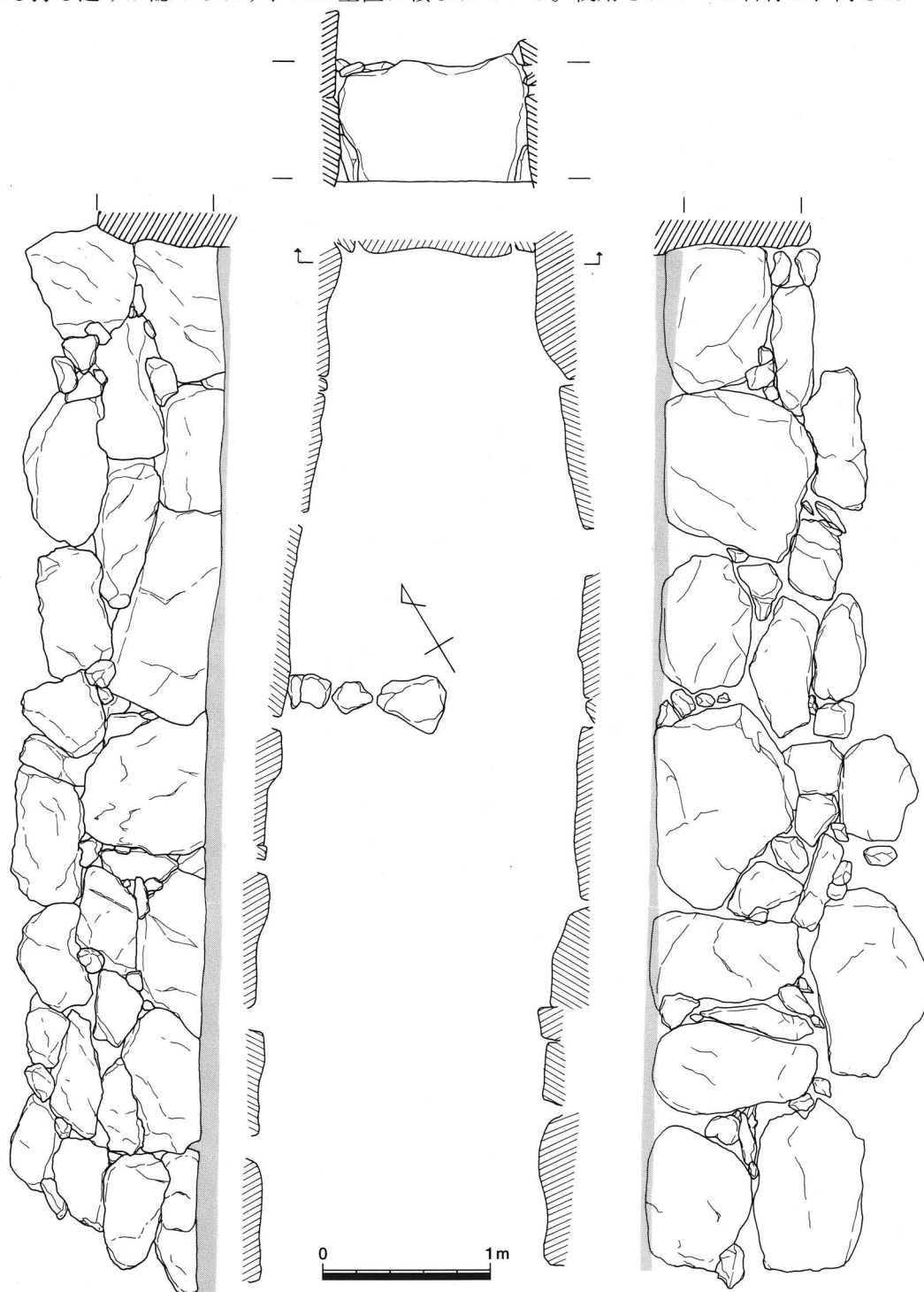
図5 石室(1/40)
