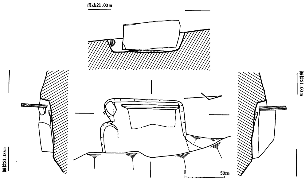
第11図 大見観音崎石棺群第5号石棺実測図
