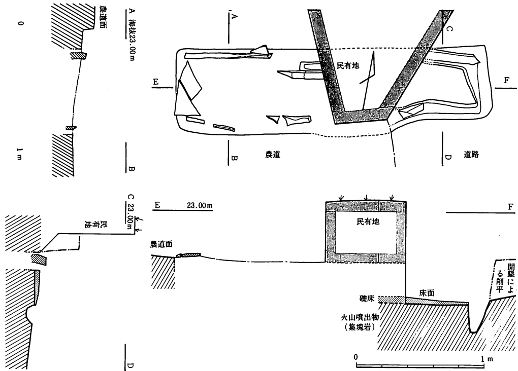
第12図 大見観音崎第6号石棺実測図
