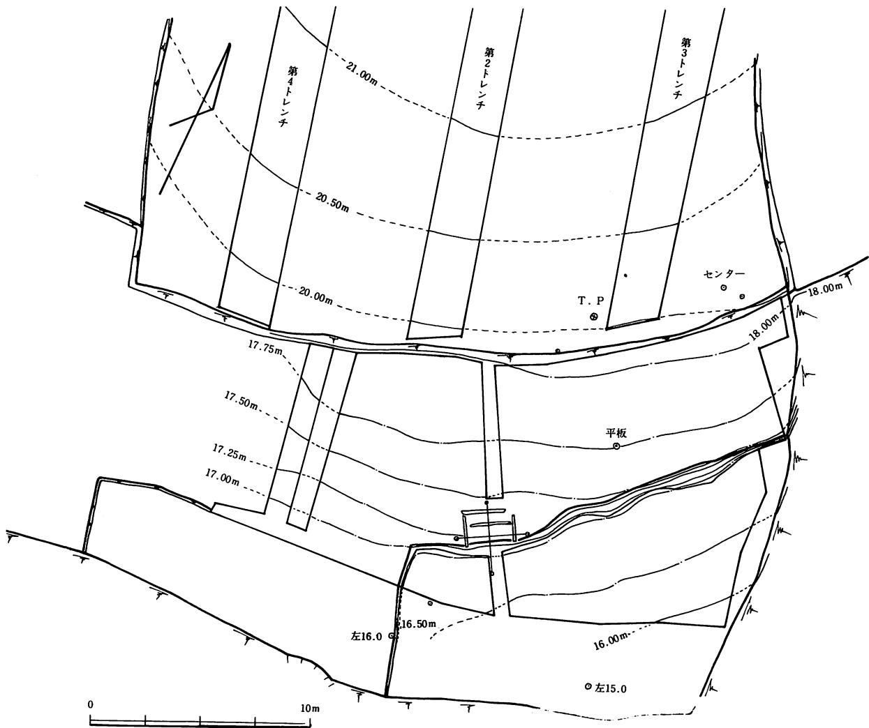
第21図 大串古墳石室周辺地形図（等高線は表土を排除後の面に引く）
