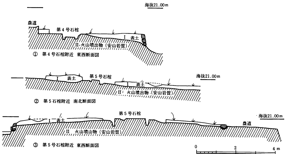
第32図 要古墳群第4・5号石棺周辺土層図
