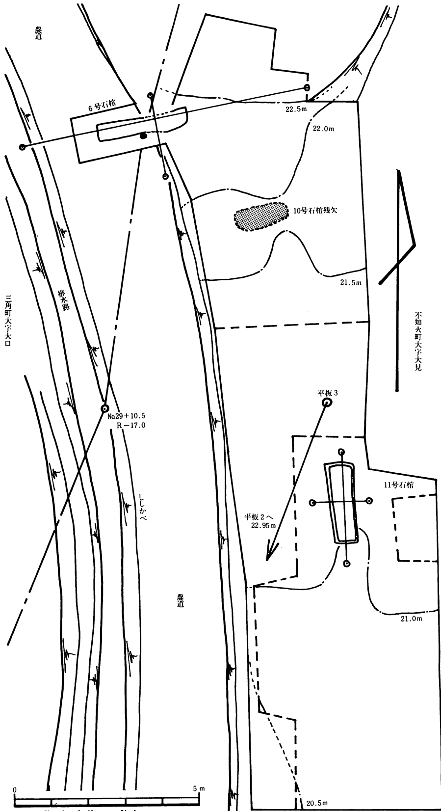
第7図 第6・10・11号石棺発掘区域図
