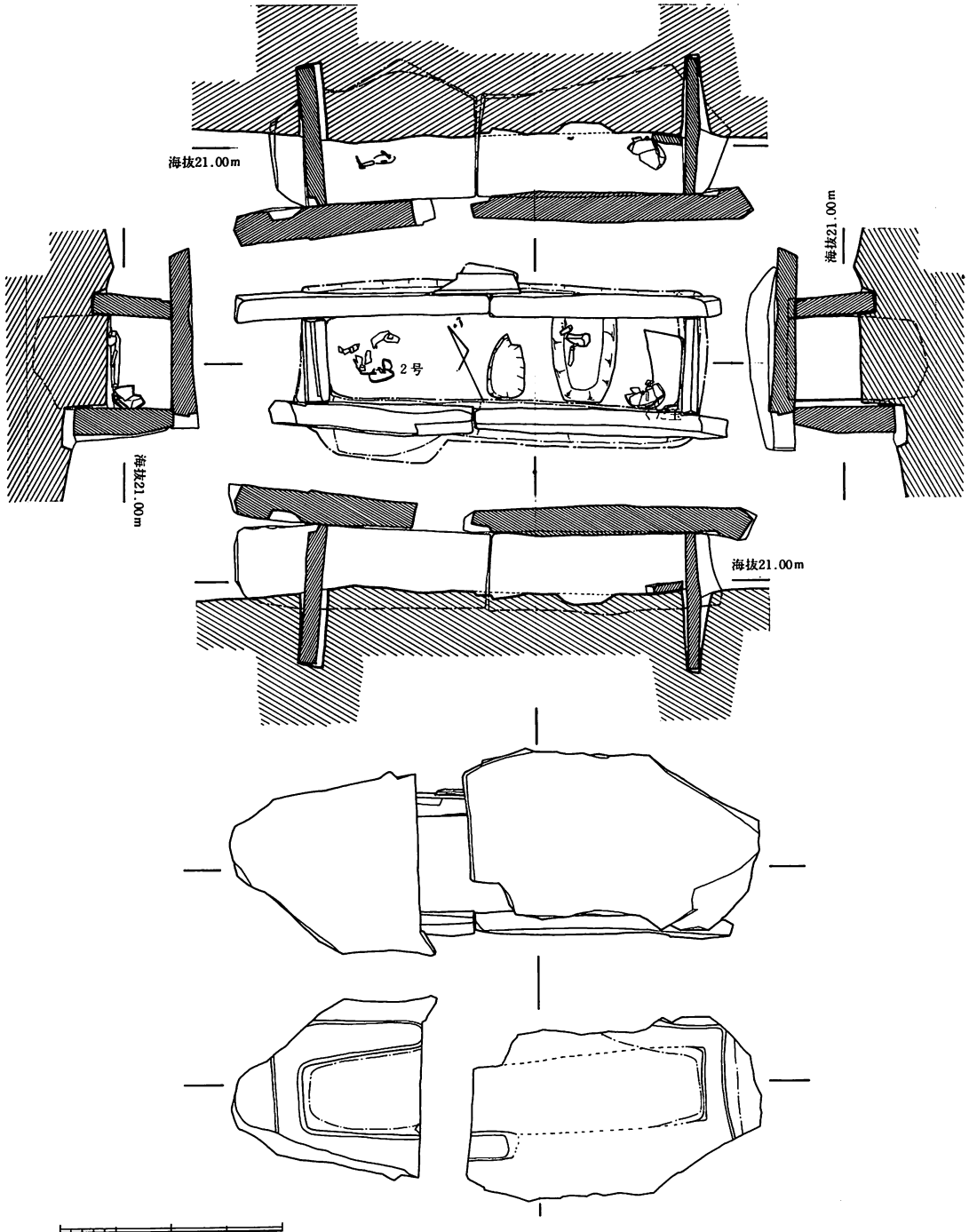
第30図 要古墳群第5号石棺実測図
