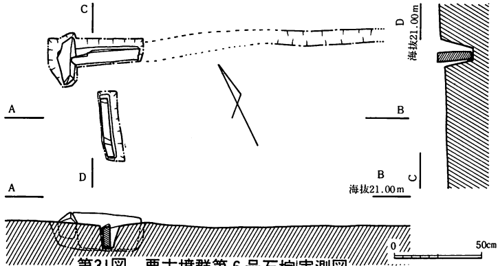
第31図 要古墳群第6号石棺実測図
