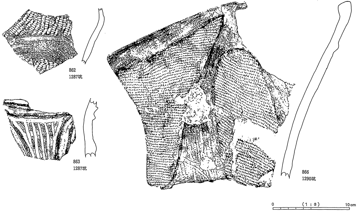
圖版183 土坑出土土器(39) (859 1:6、864 1:4、他 1:3)
