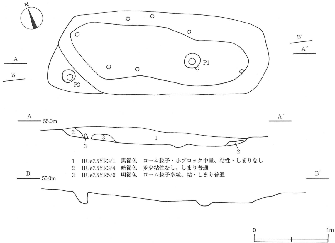
第9図 A調査区土坑遺構実測図
