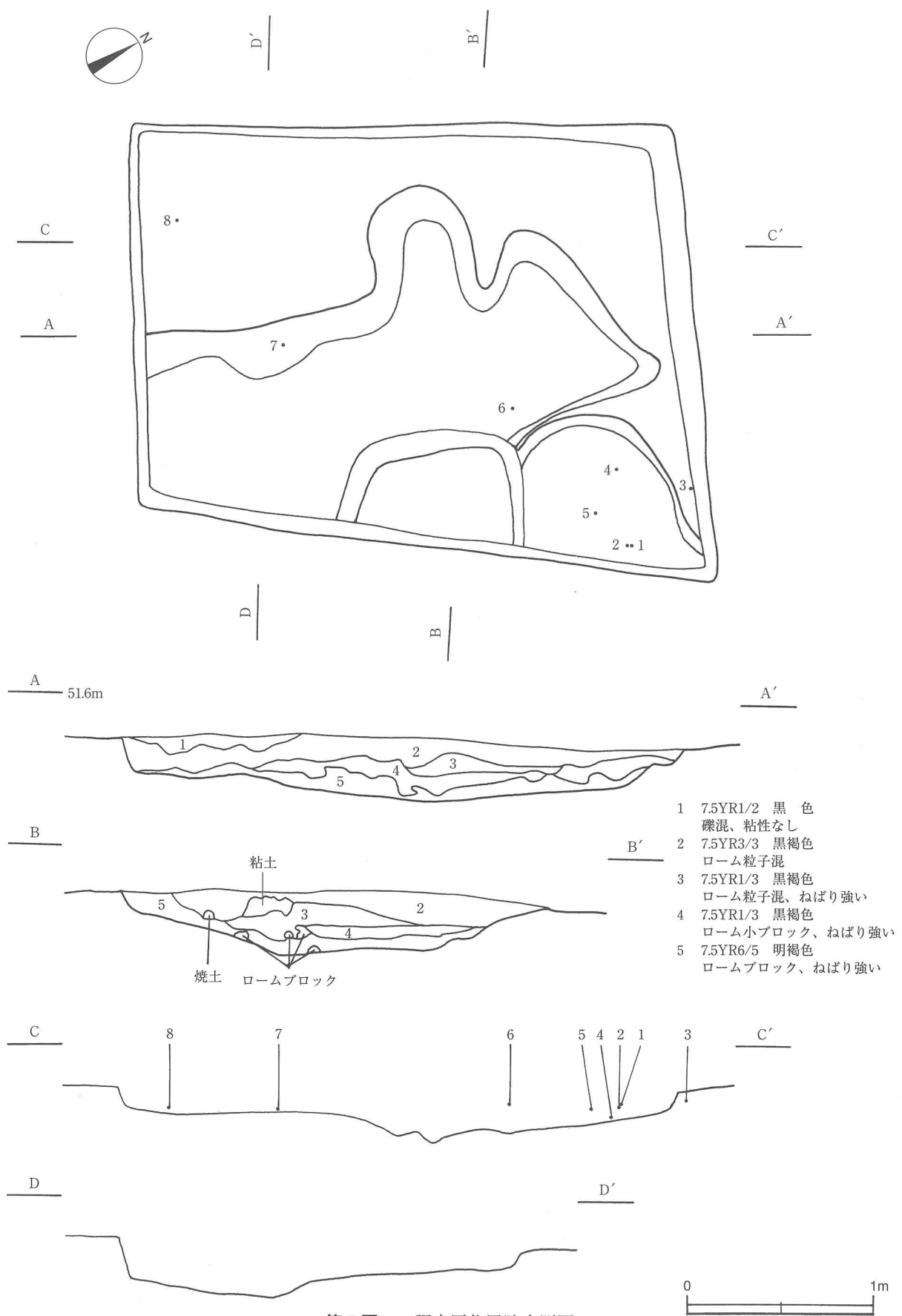
第5図 B調査区住居跡実測図
