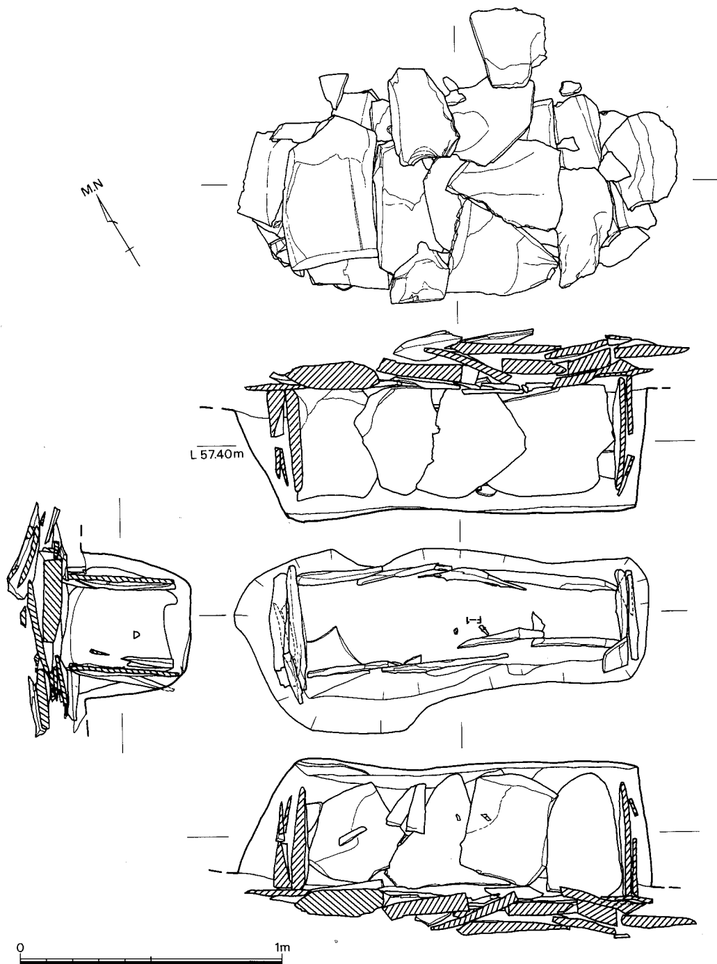
第13图 19号石棺实测图 (1/20)
