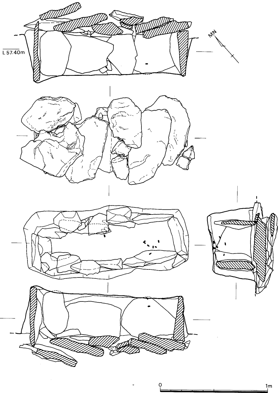
第 5 图 11号石棺实测图 (1/20)
