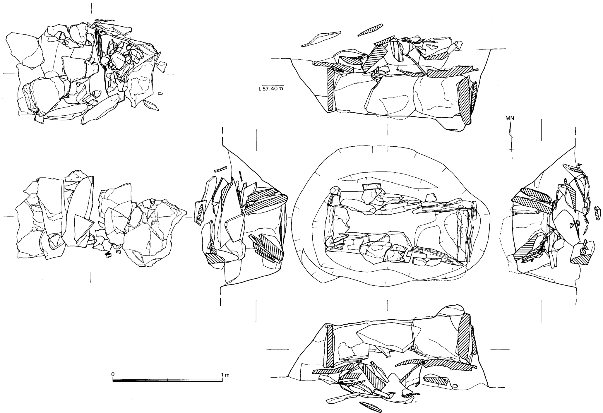
第10图 16号石棺实测图
