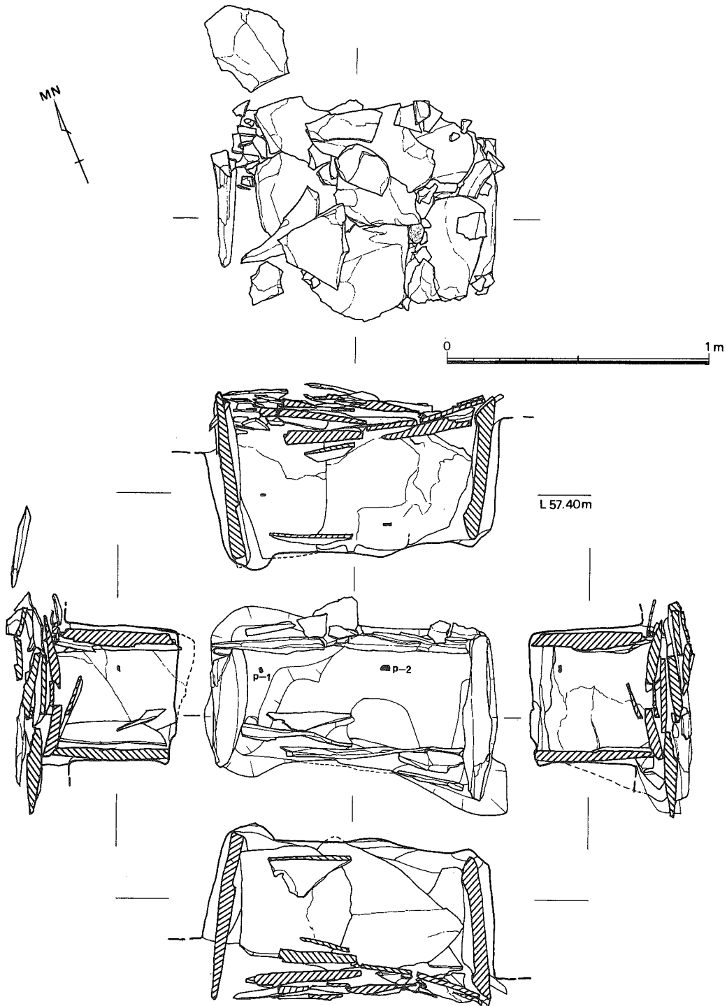
第12图 18号石棺实测图 (1/20)
