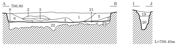
カマド図
