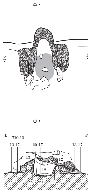
カマド図
