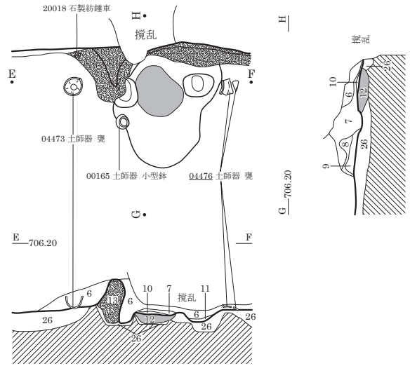
カマド図
