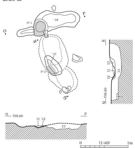
鍛冶炉図
