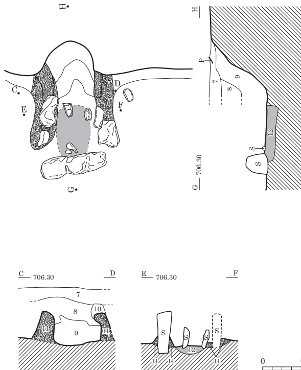
カマド図
