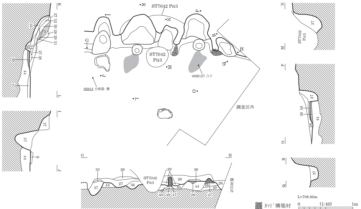
カマド図
