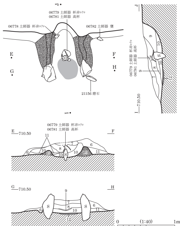
カマド図
