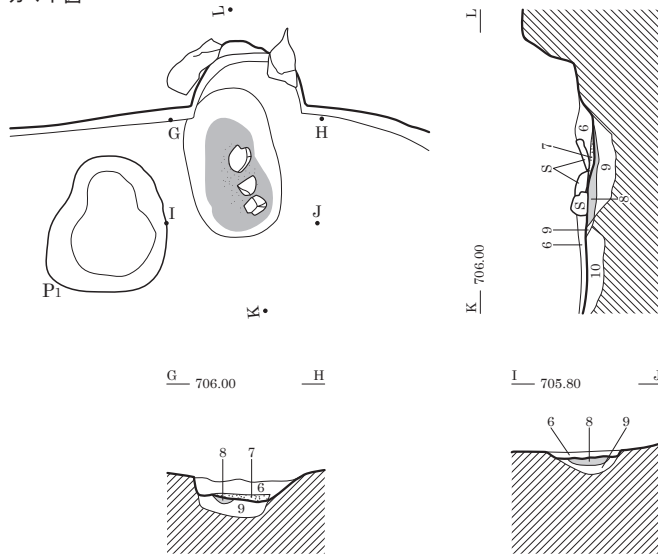
カマド図
