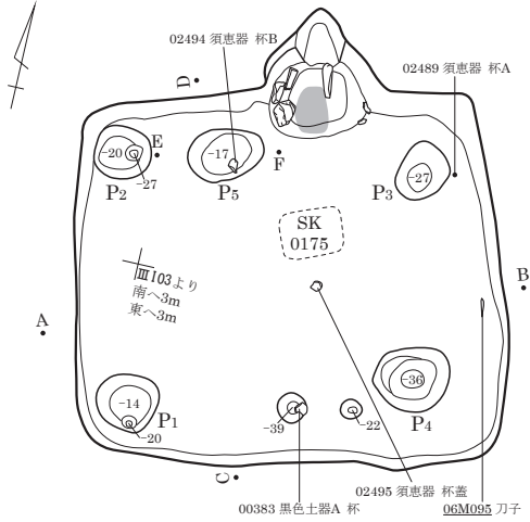
掘方平面図
