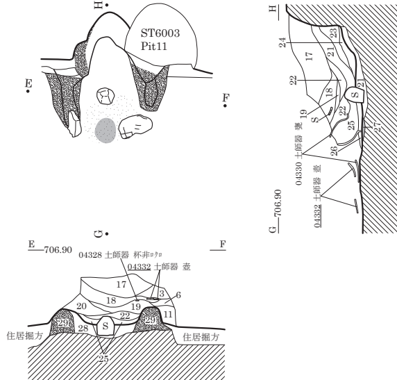
カマド図
