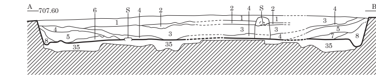
カマド図
