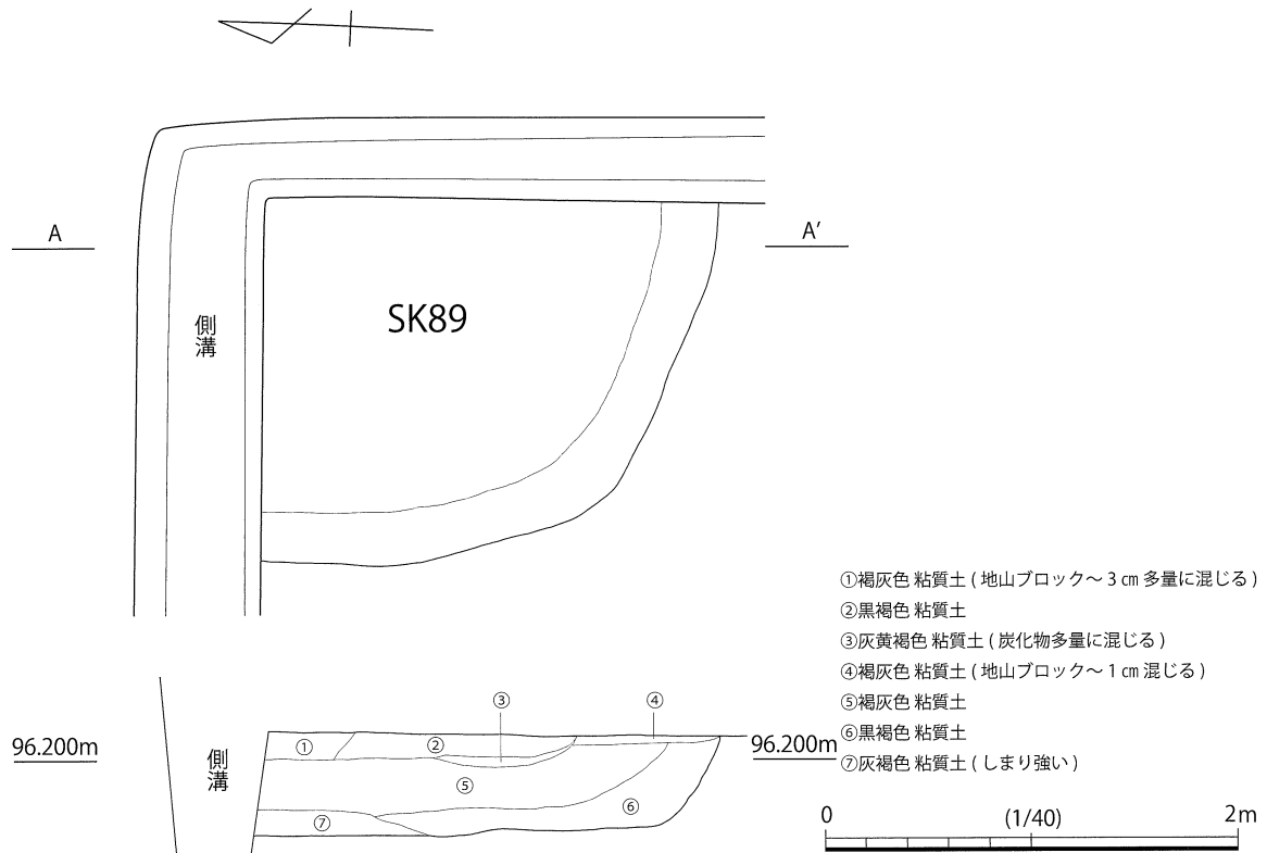
図13 土坑 (SK89) 平面図・断面図
