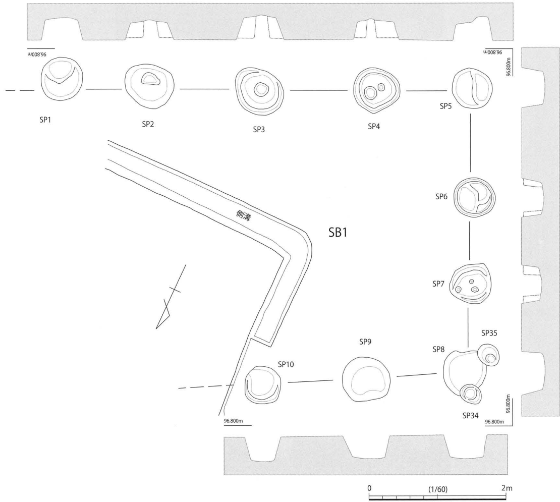
図9 掘立柱建物 (SB1) 平面図・断面図
