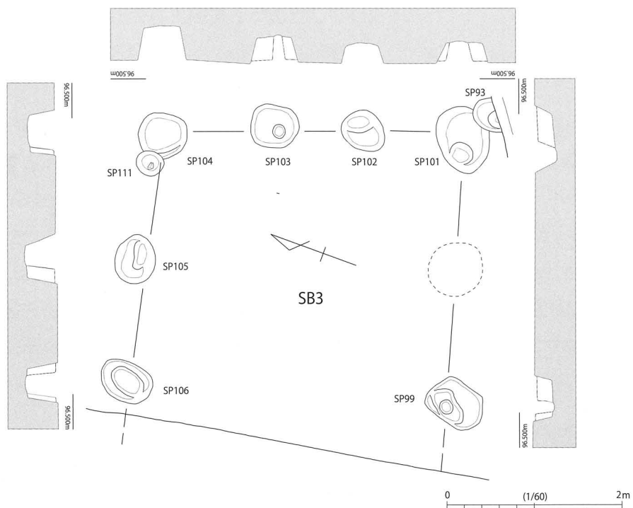
図10 掘立柱建物 (SB3) 平面図・断面図
