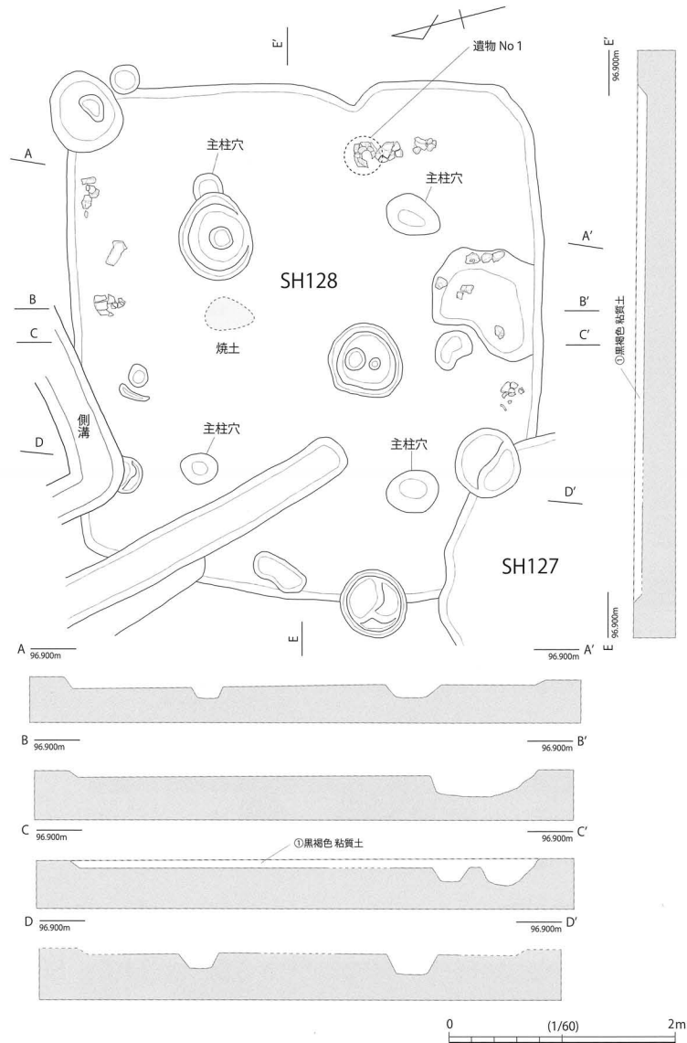
図7 竪穴建物 (SH128) 平面図・断面図
