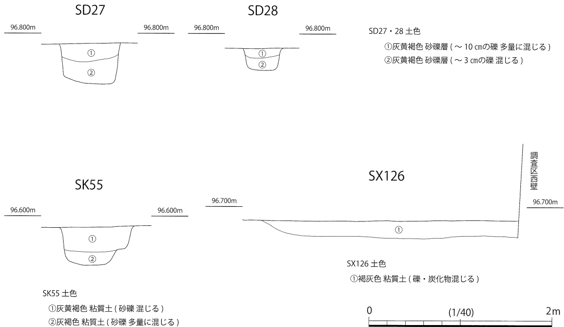
図14 各遺構 (SD27・SD28・SK55・SX126) 断面図
