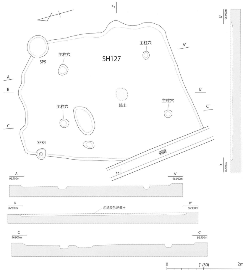
図8 竪穴建物 (SH127) 平面図・断面図
