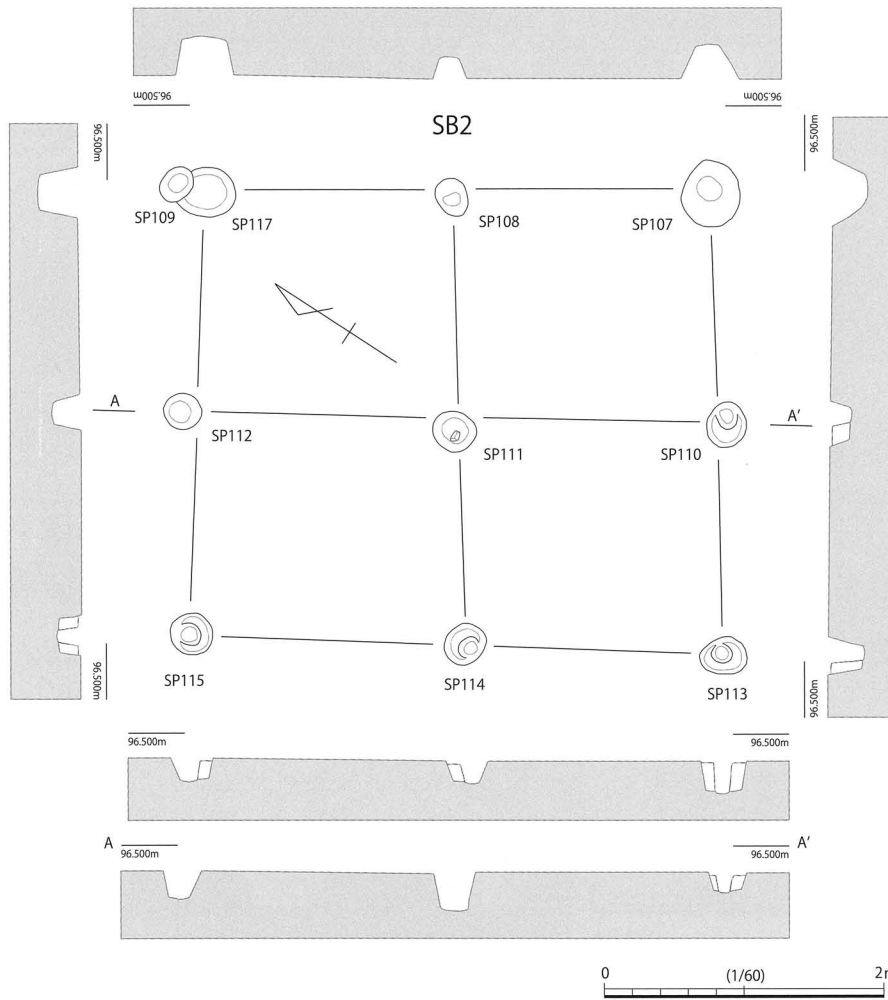
図11 掘立柱建物 (SB 2) 平面図・断面図
