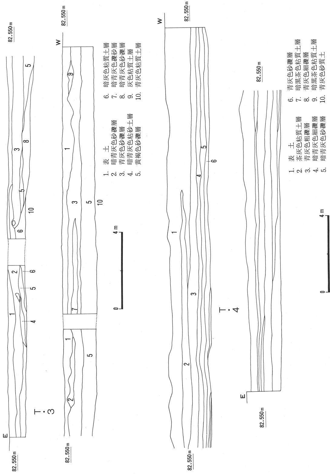
第6図 トレンチ断面図(2)
