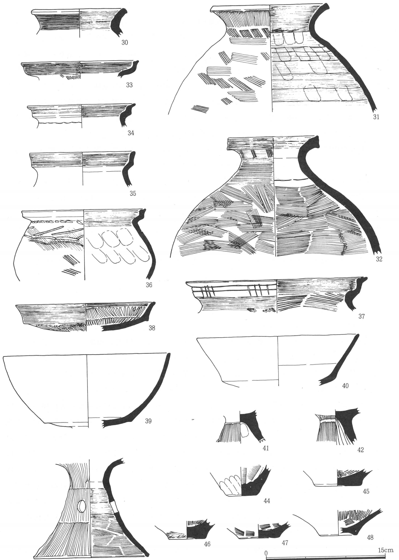
第13图 T-4 出土遺物実測図
