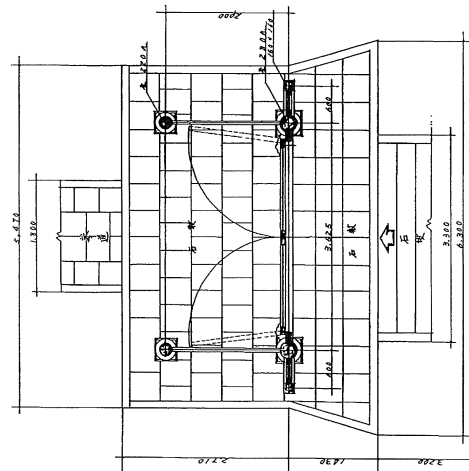
平面圖
