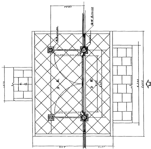
平面图
