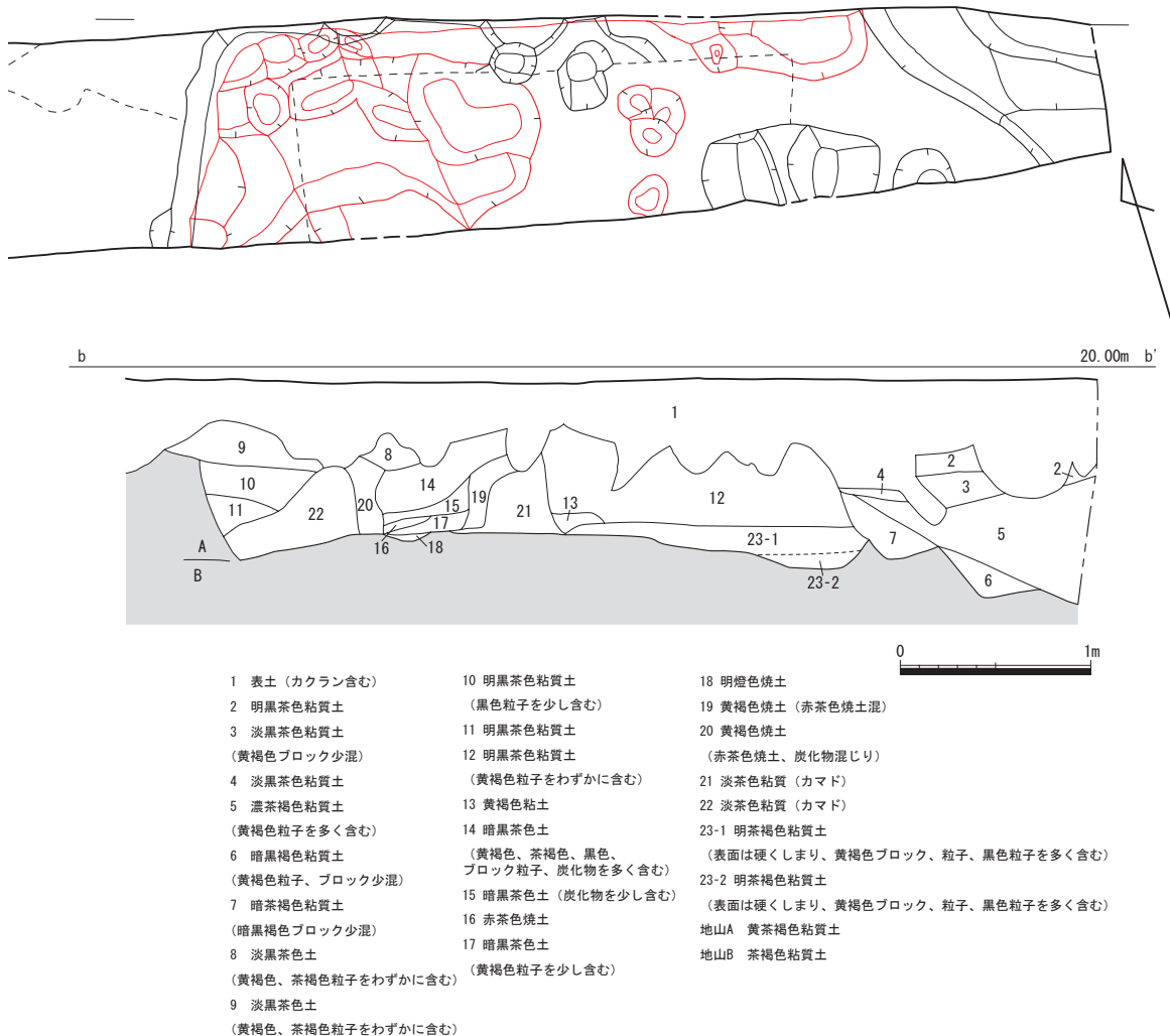
Fig.3 4SI05 実測図 (1/40)
