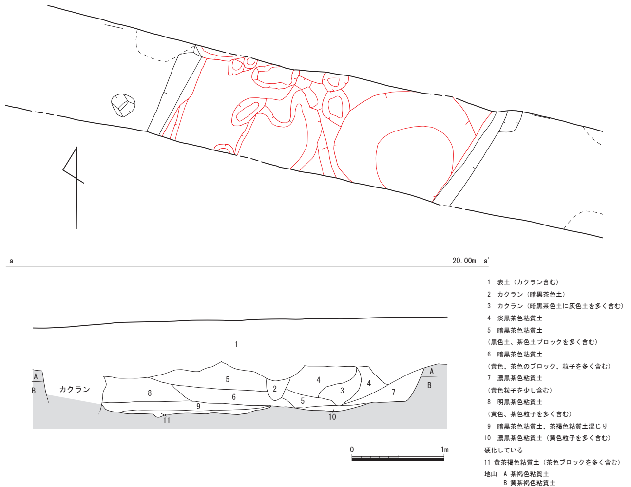
Fig.4 4SI10 実測図 (1/40)
