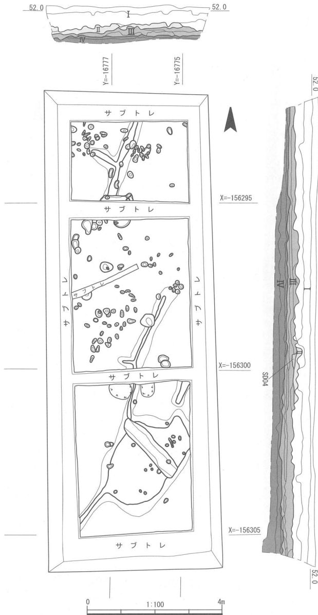
第11図 下層遺構面平面図および東・北壁断面図
