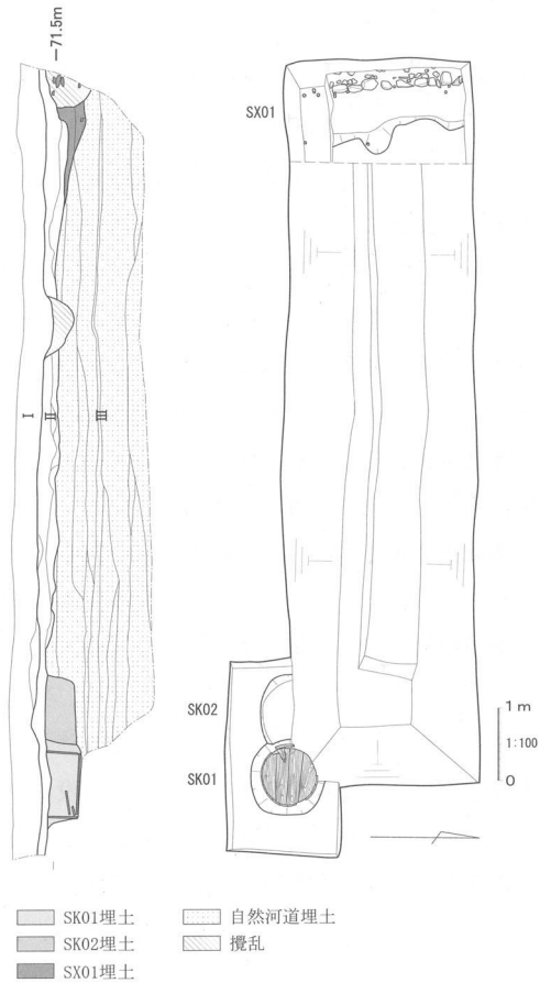
第4図 調査区平面図・土層図
