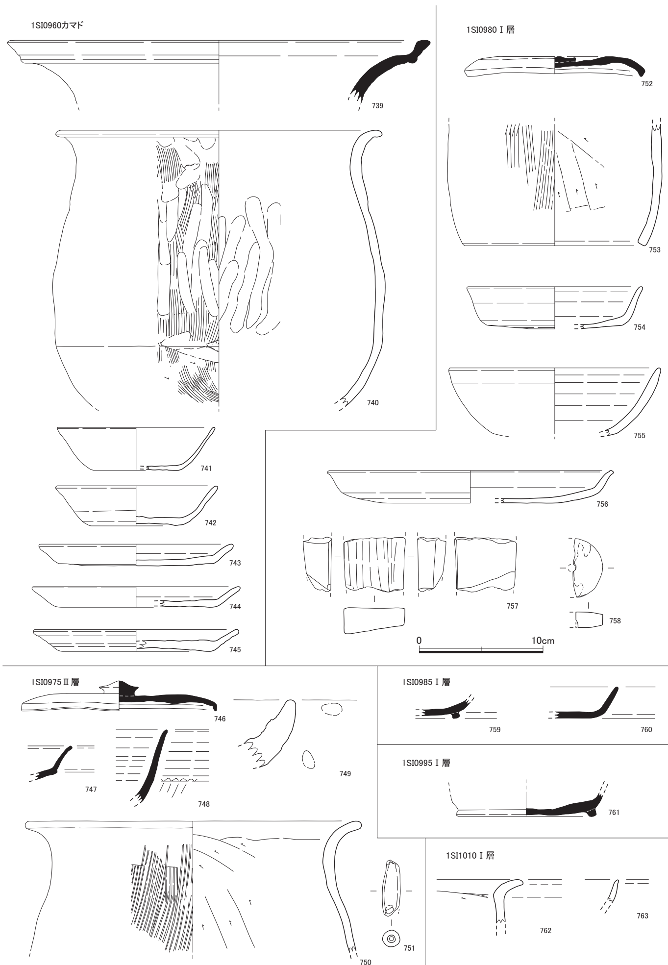
Fig.38 若菜森坊遺跡第1次調査 出土遺物実測図36 (1/3)
