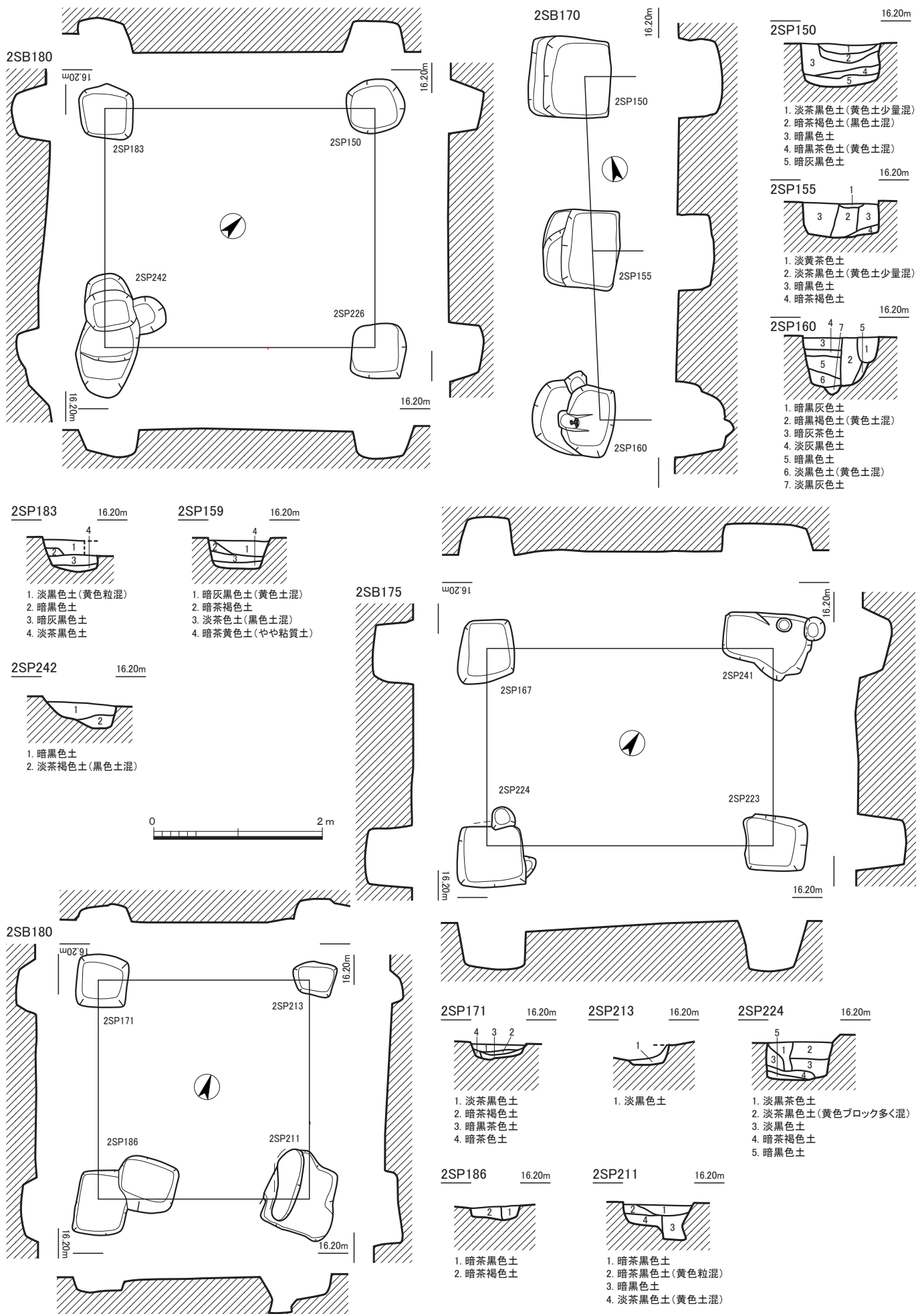
Fig.63 若菜森坊遺跡第2次調査 遺構実測図2 (1 / 60)
