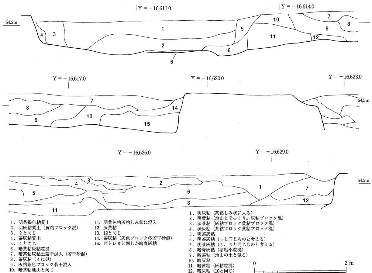
Fig. 6 SX031土層観察図 (1/50)
