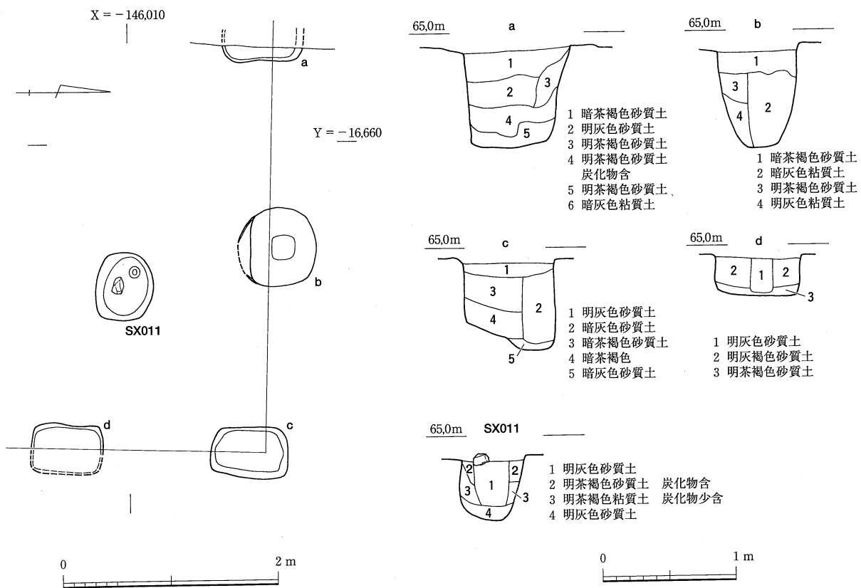
Fig. 4 SB010実測図 (1/50) 及び柱堀方土層観察図 (1/40)
