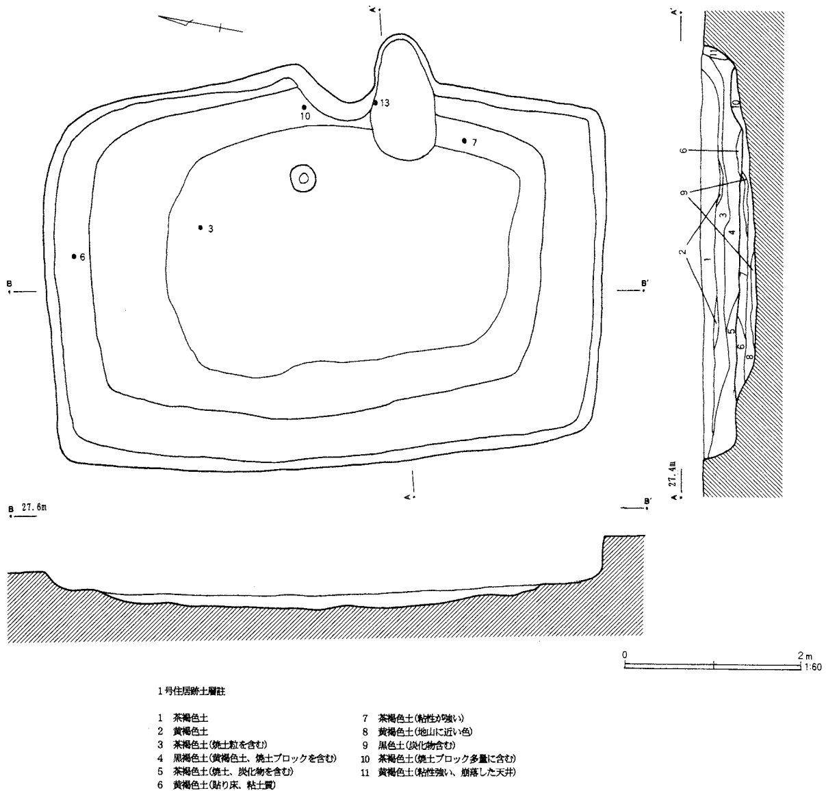
第4図 第1号住居跡全測図
