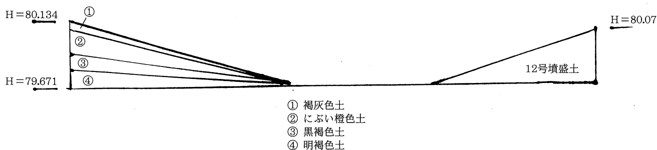
第9図 トレンチ断面図
