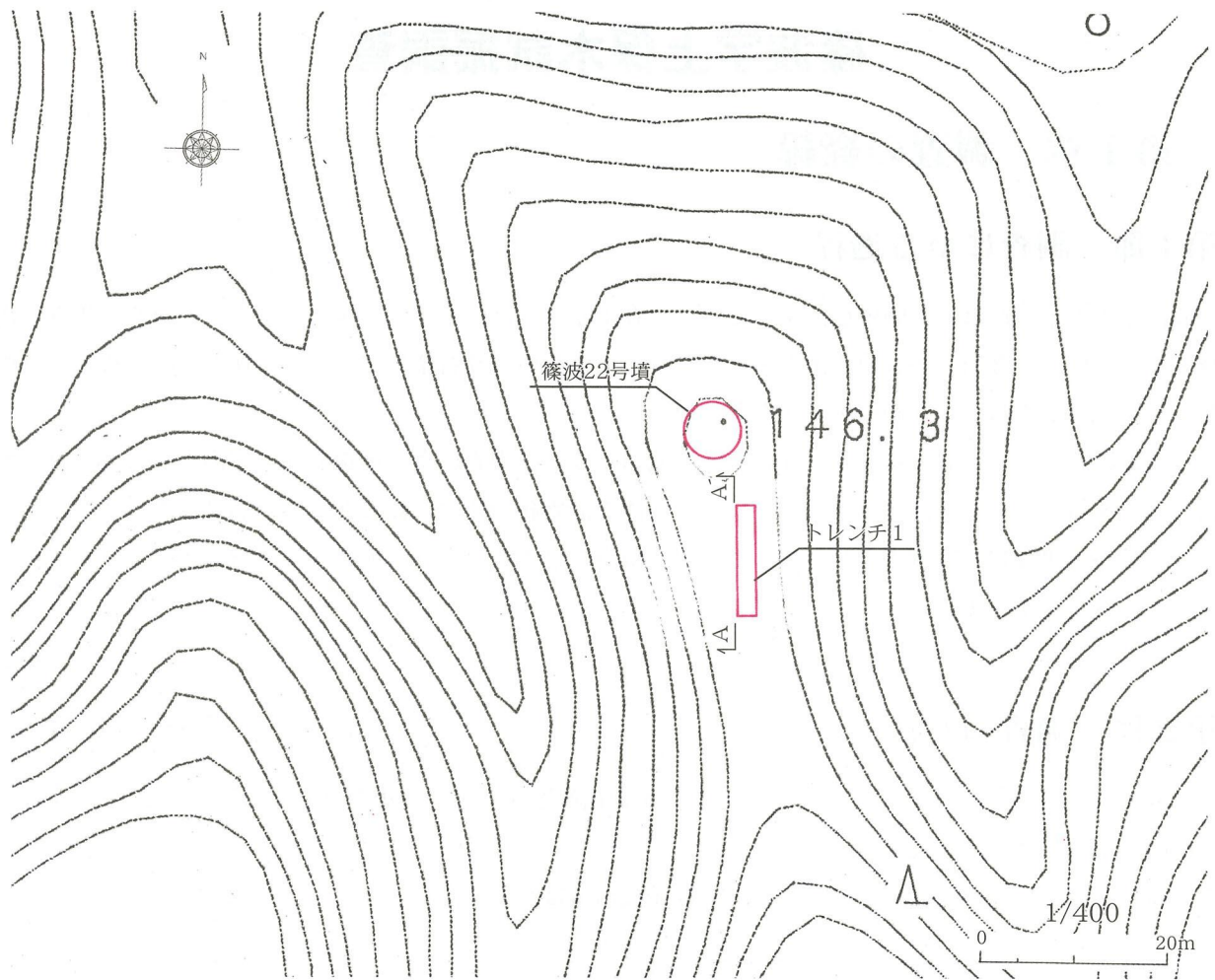
第4図 トレンチ配置図
