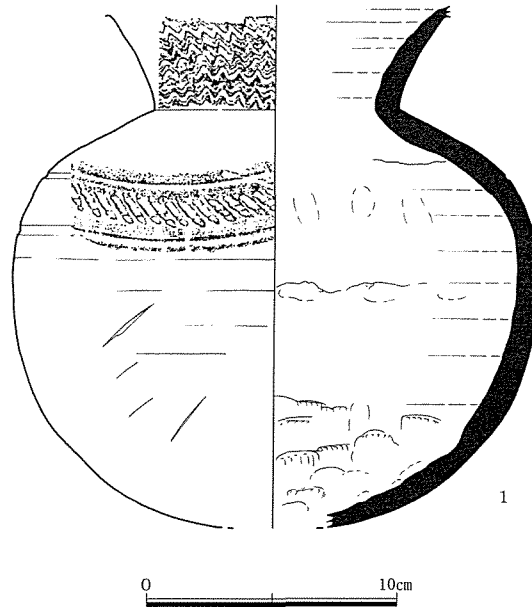
第9図 墳丘外出土遺物実測図
