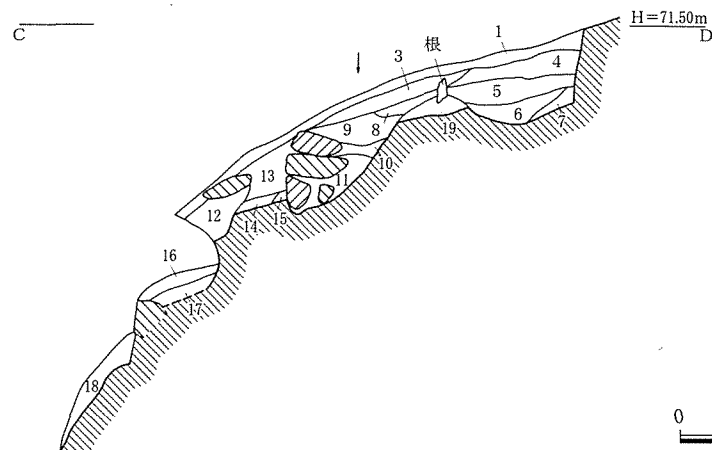
第4図 墳丘断面図 (S=1:80)
