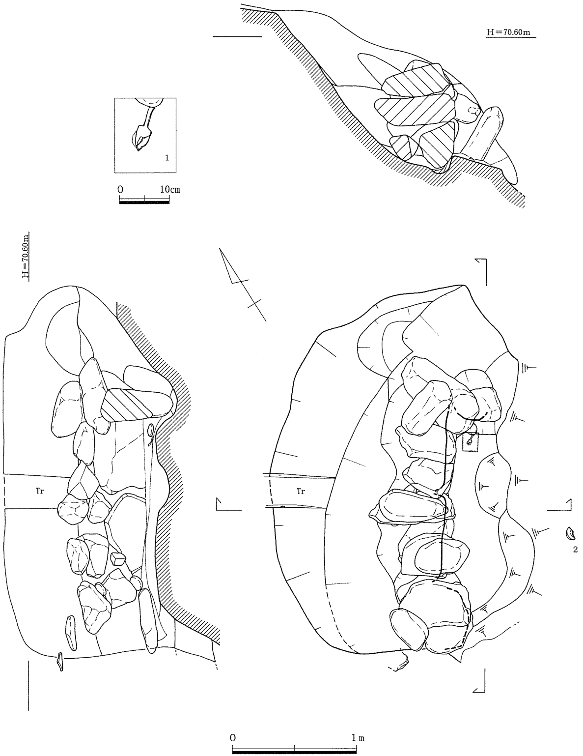
第6図 石室実測図 (S=1:30)
