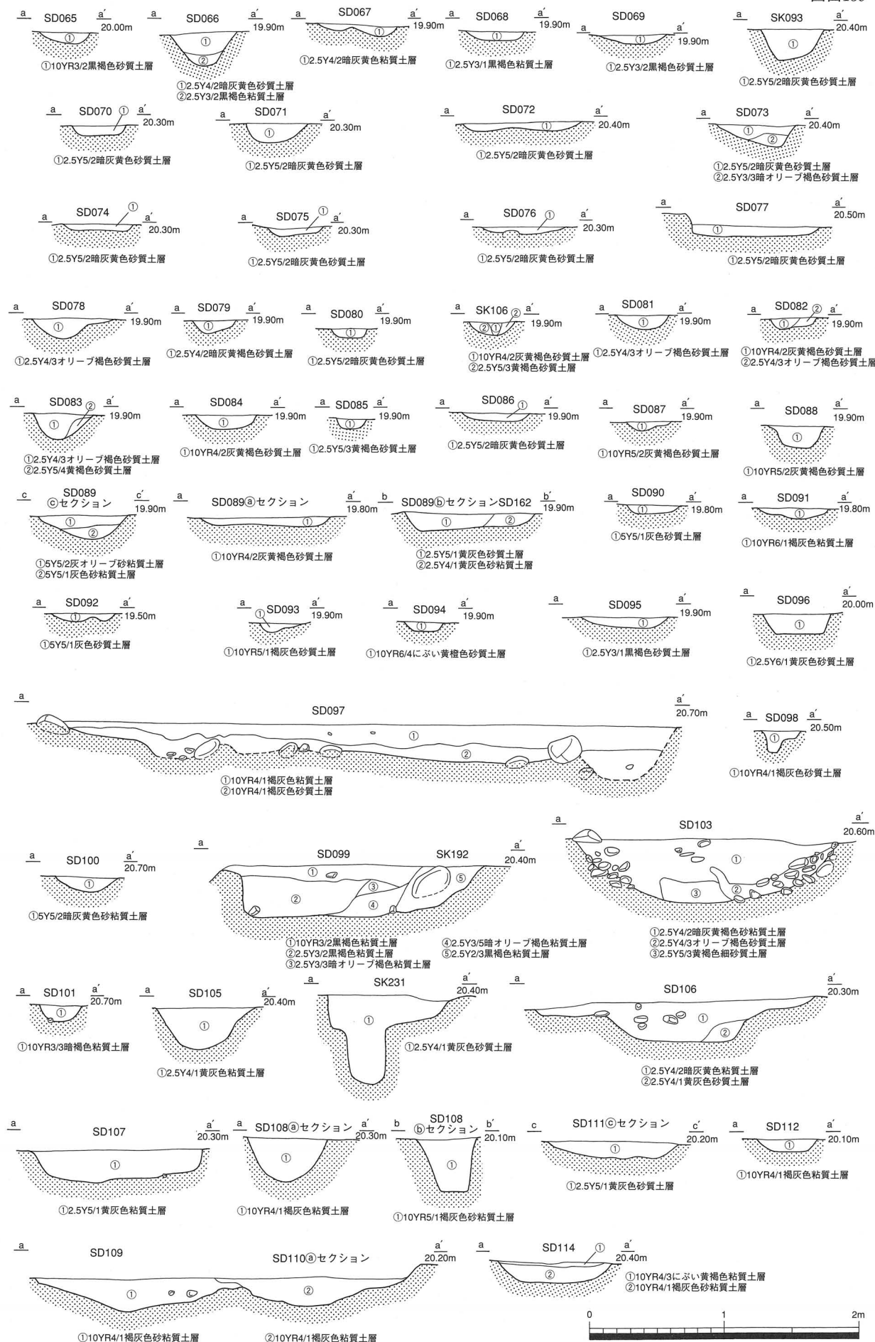
A地区溝・土坑断面図(7)
