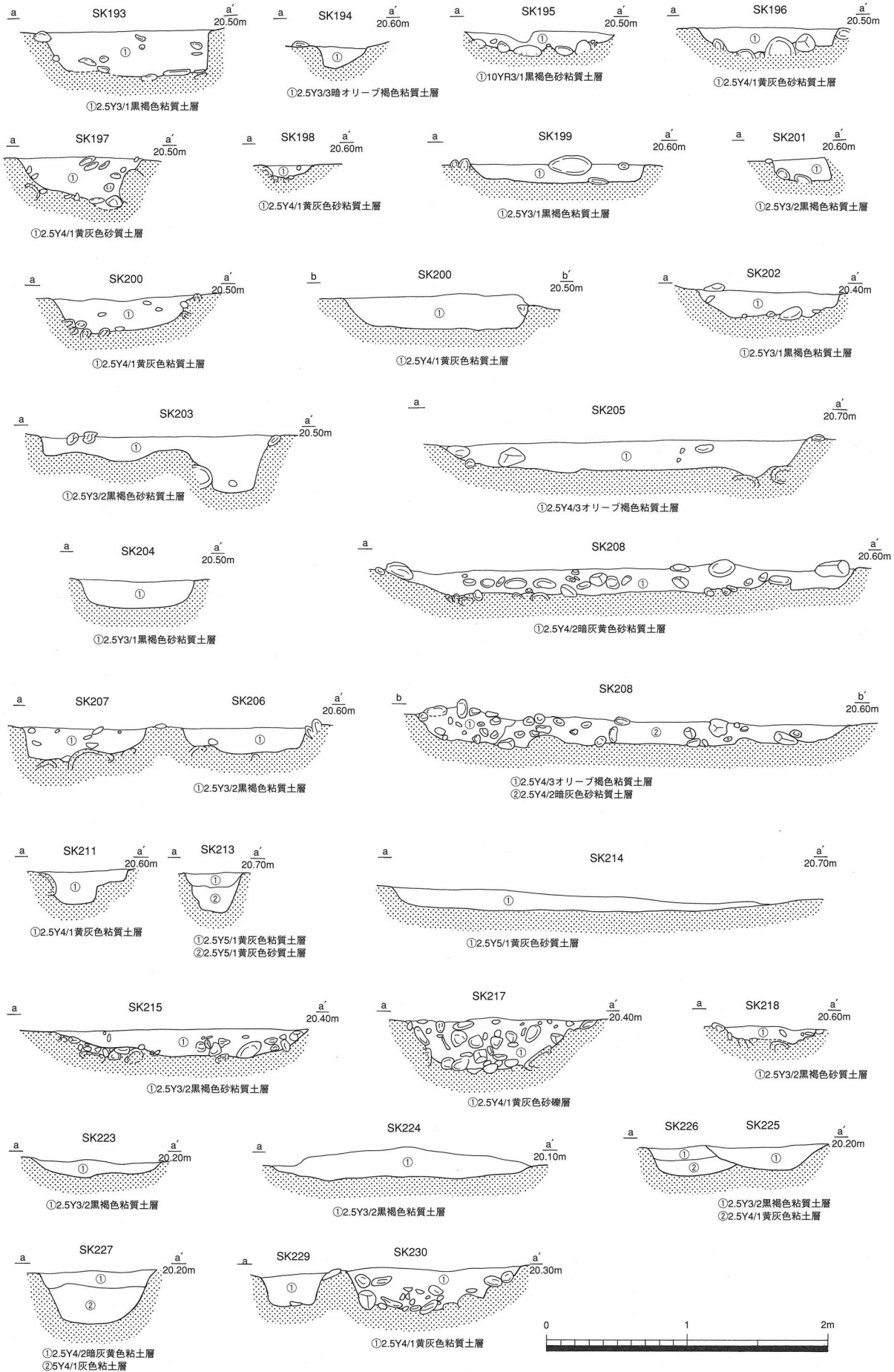
A地区溝・土坑断面図(2)
