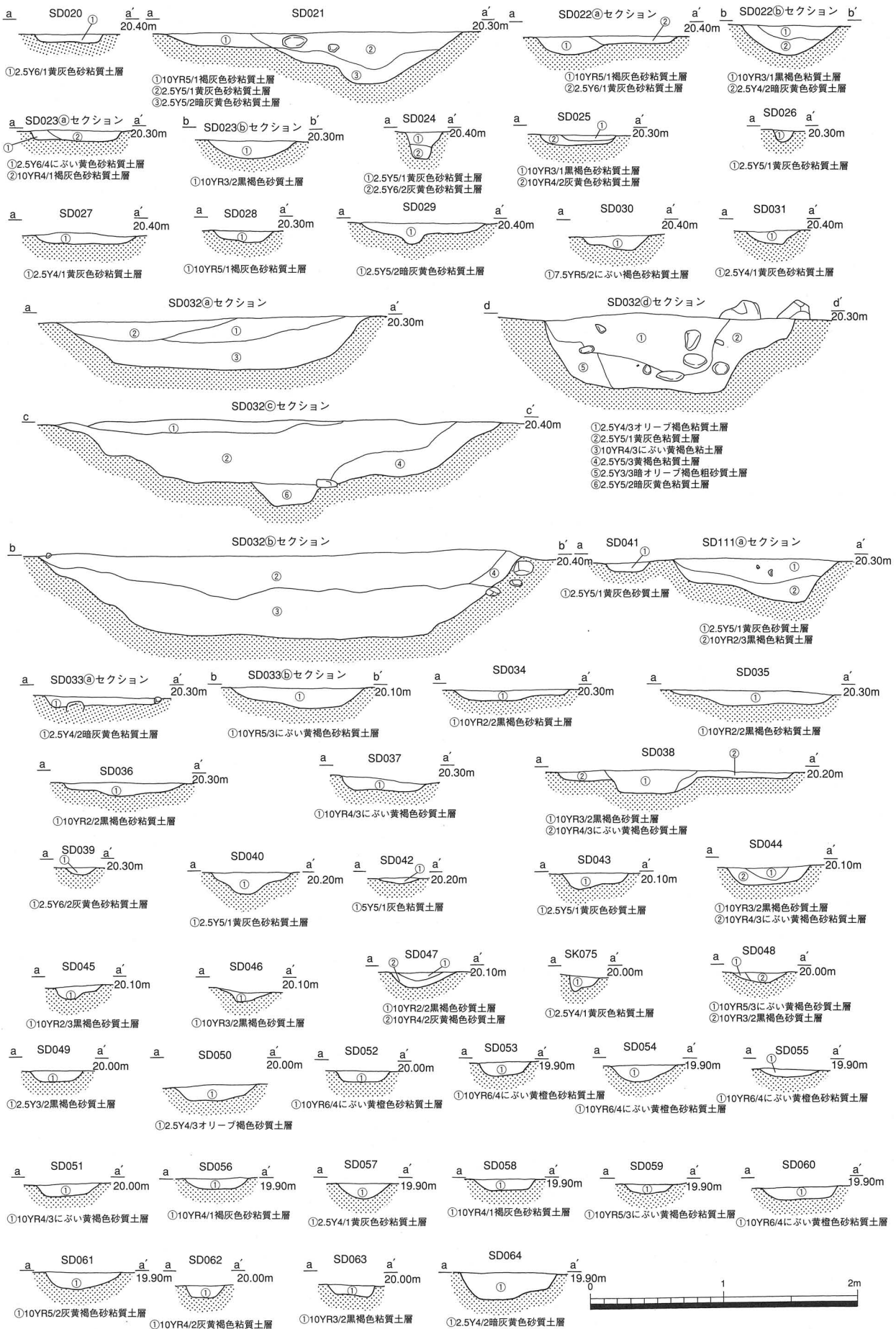
A地区溝・土坑断面図(6)
