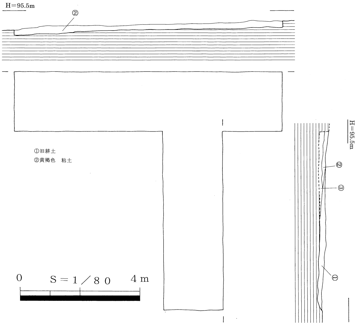
上種地区 トレンチ断面図
