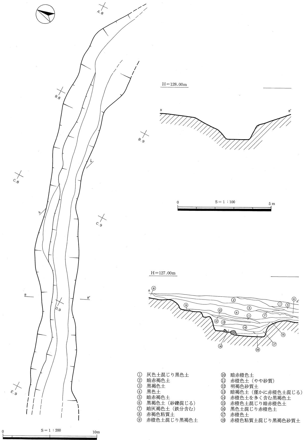
第21図 S D - 11実測図
