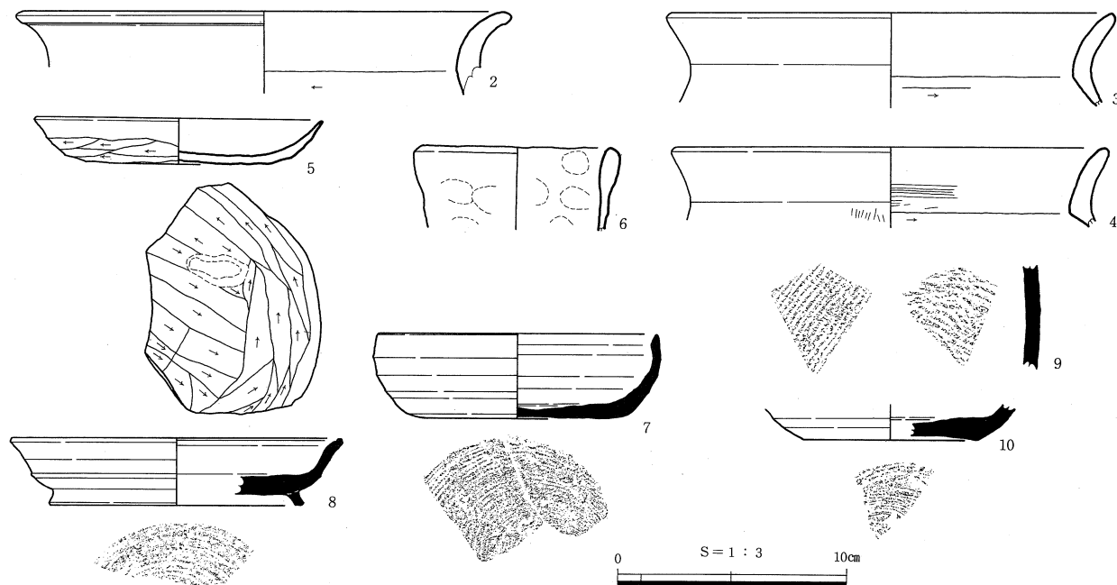
第15図 SS-1、3出土遺物実測図
