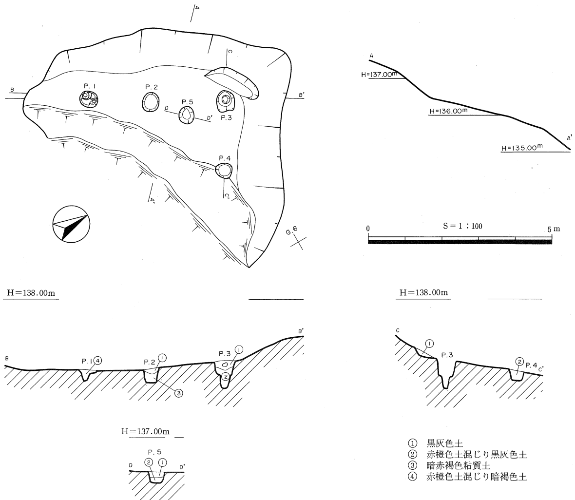
第17図 SS-2 実測図
