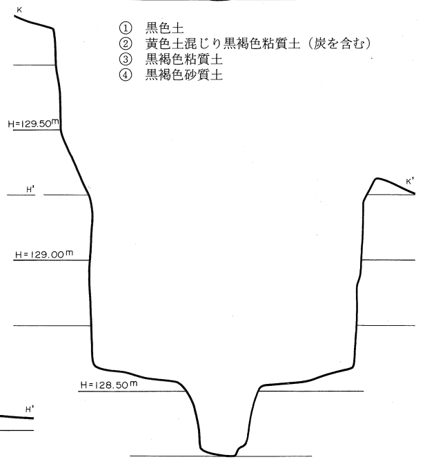
第18図 SK-10~12実測図
