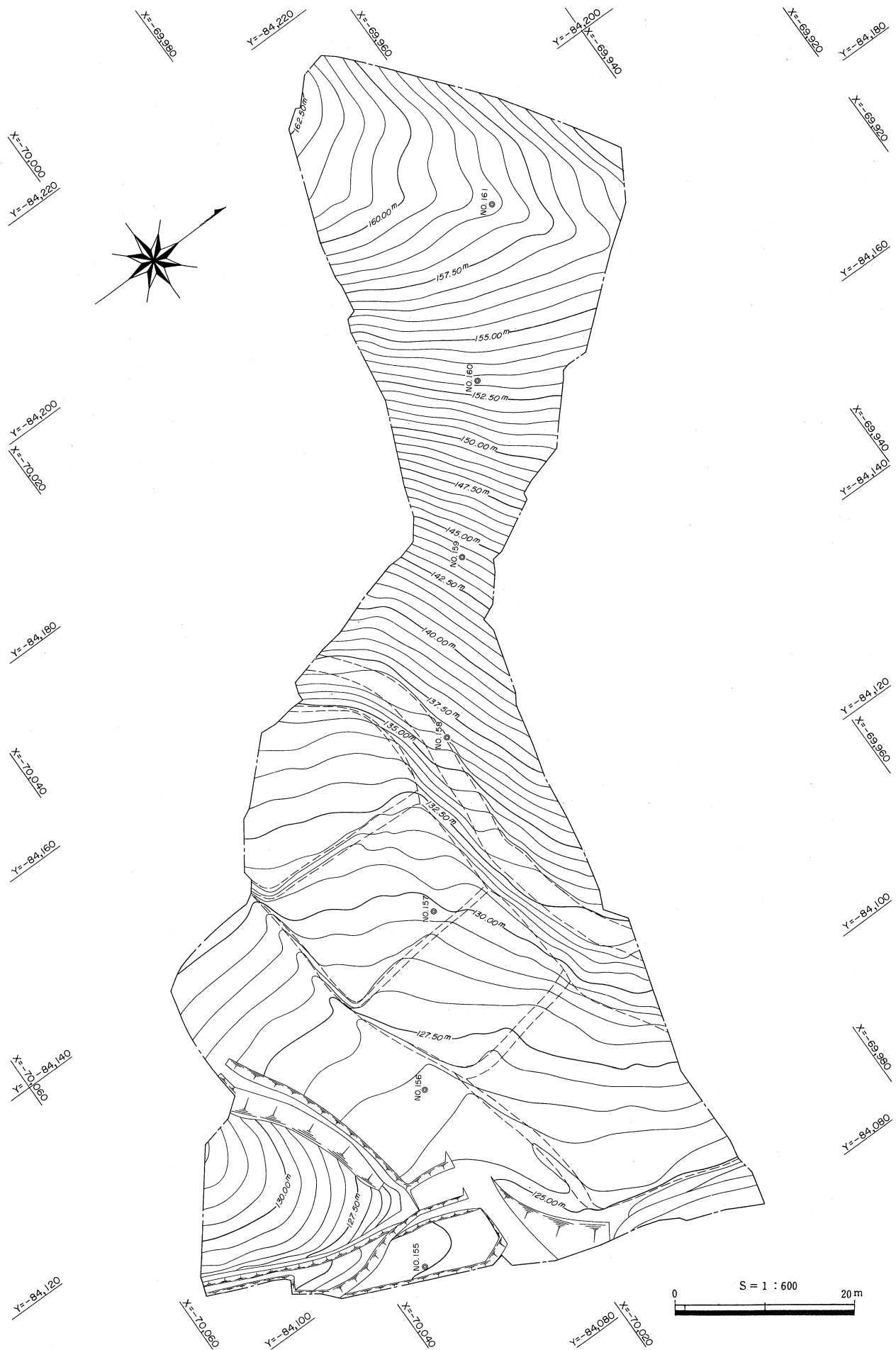
第 6 図 調査地調査前地形実測図
