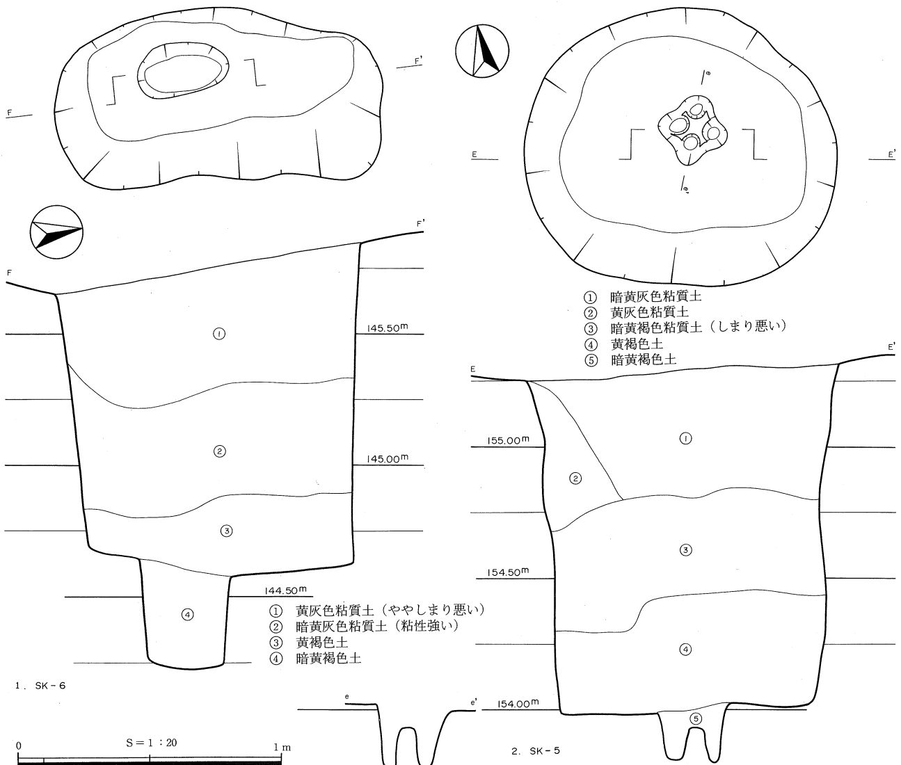
第13図 SK-5、6 実測図
