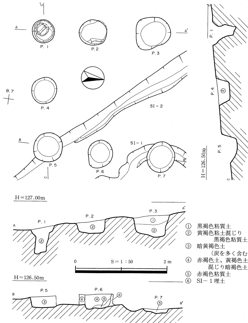
第24図 SB-1 実測図
