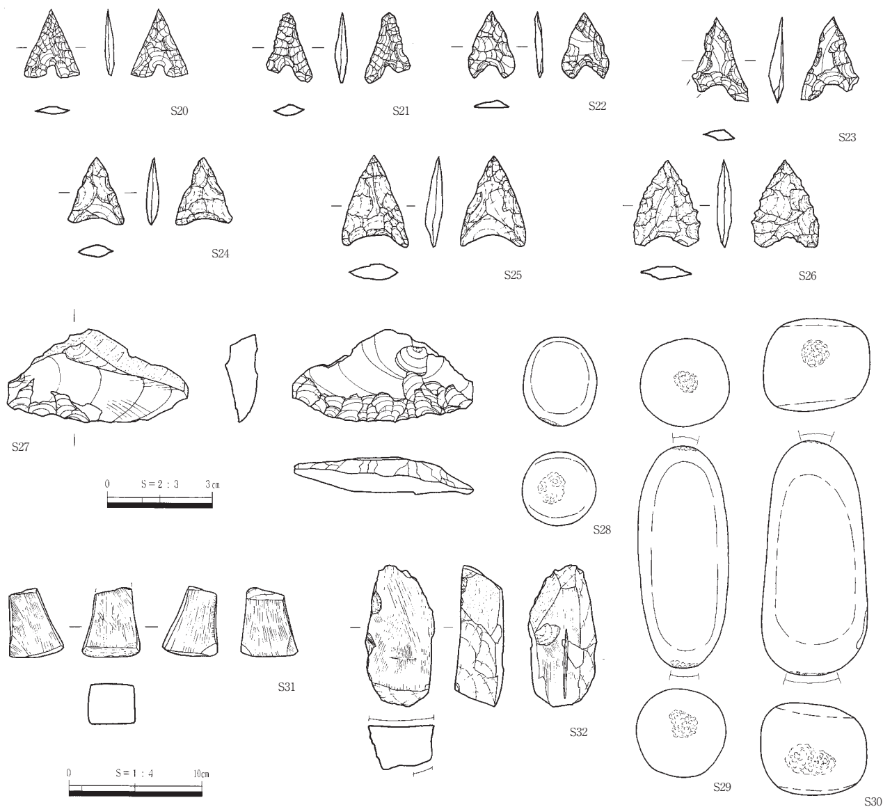
第114図 遺構外出土石器
