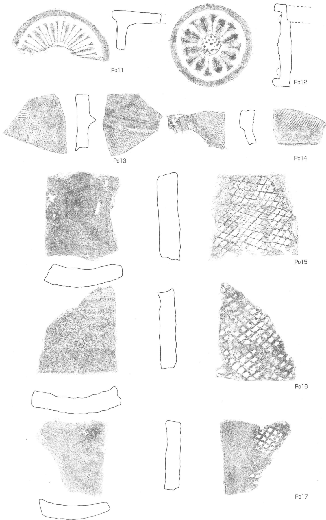
第10図 岩井地区出土遺物実測図(軒丸瓦、鴟尾、平瓦)
