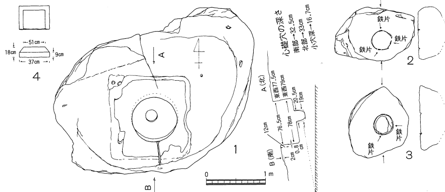
第4図 岩井廃寺関連礎石等実測図
