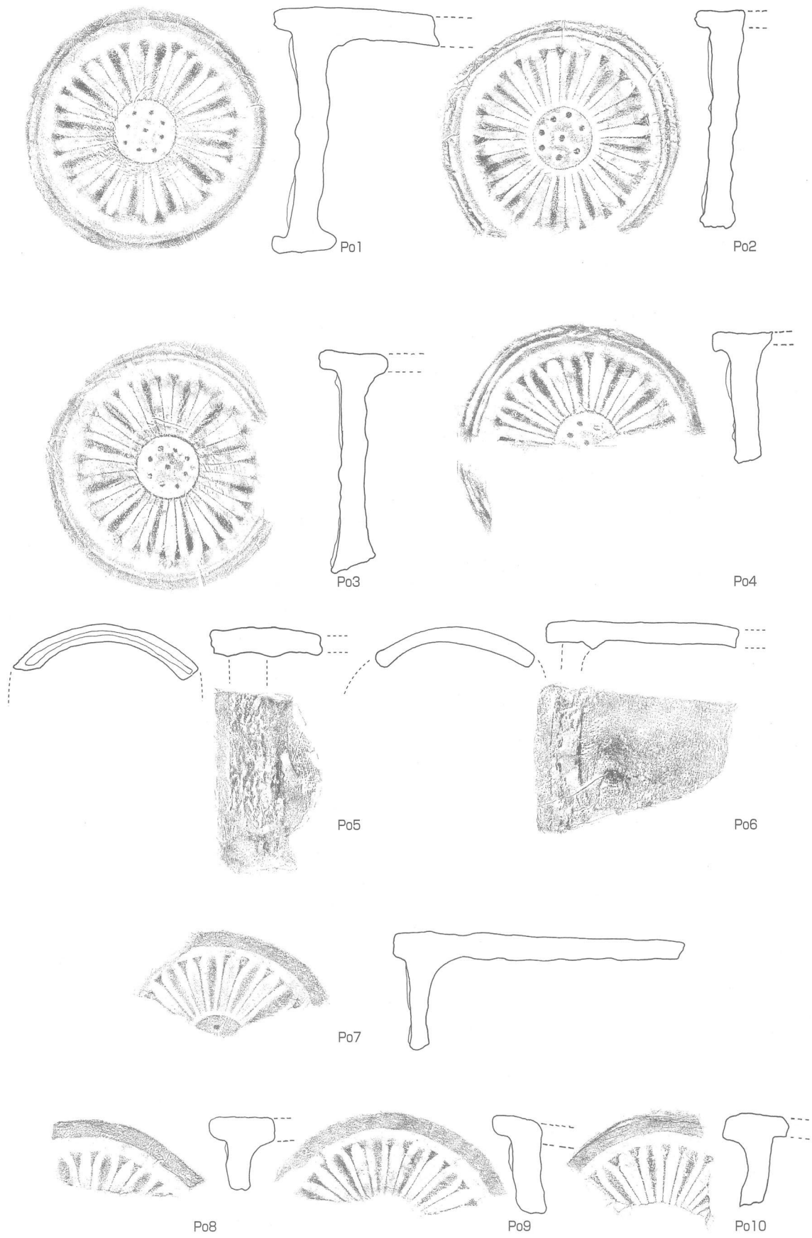
第9図 岩井地区出土遺物実測図(軒丸瓦)
