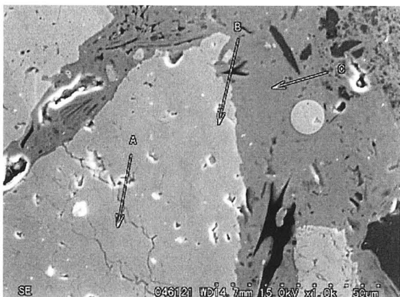
図版 5 SEM 観察組織と EDX 鉱物相微小部分析
