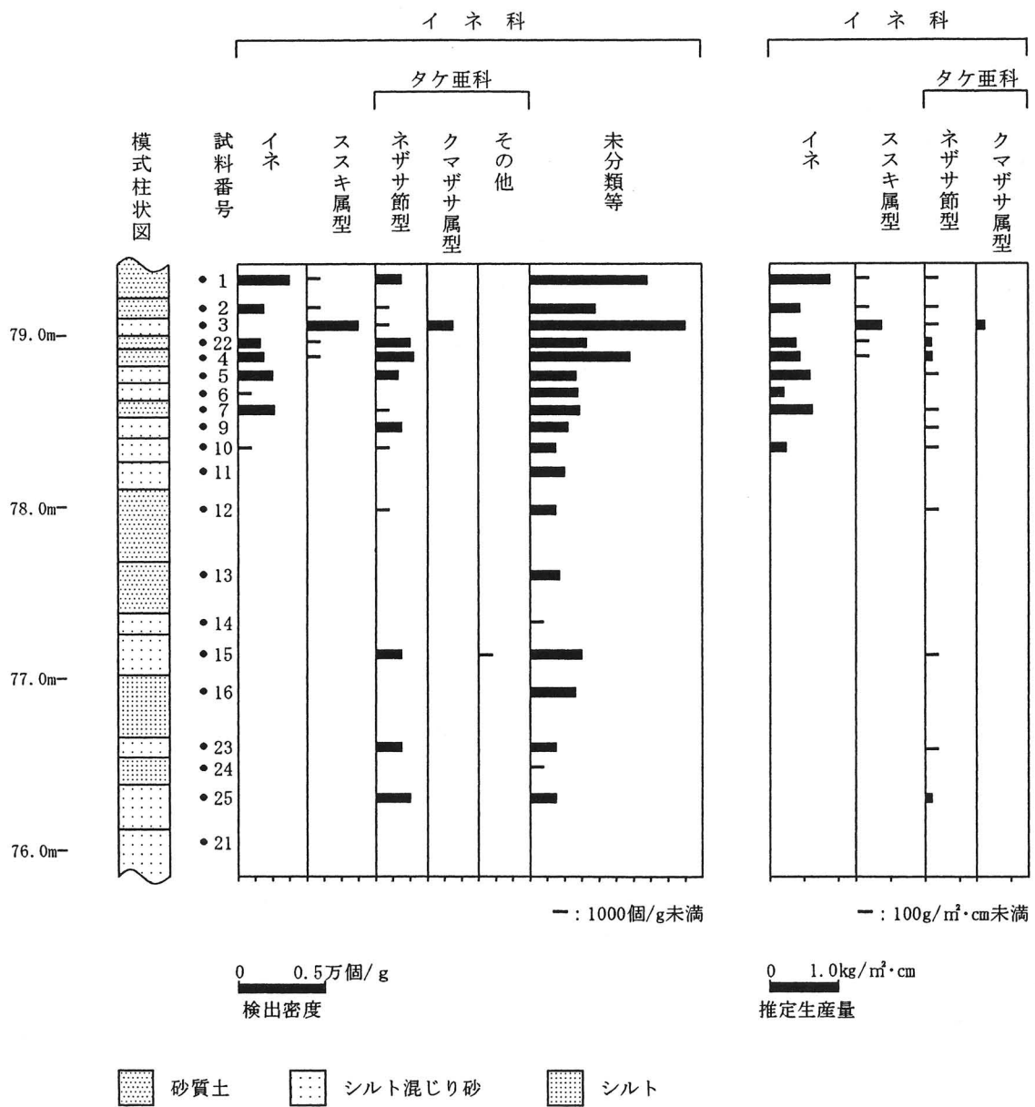
図2 A-11区地点におけるプラント・オパール分析結果
