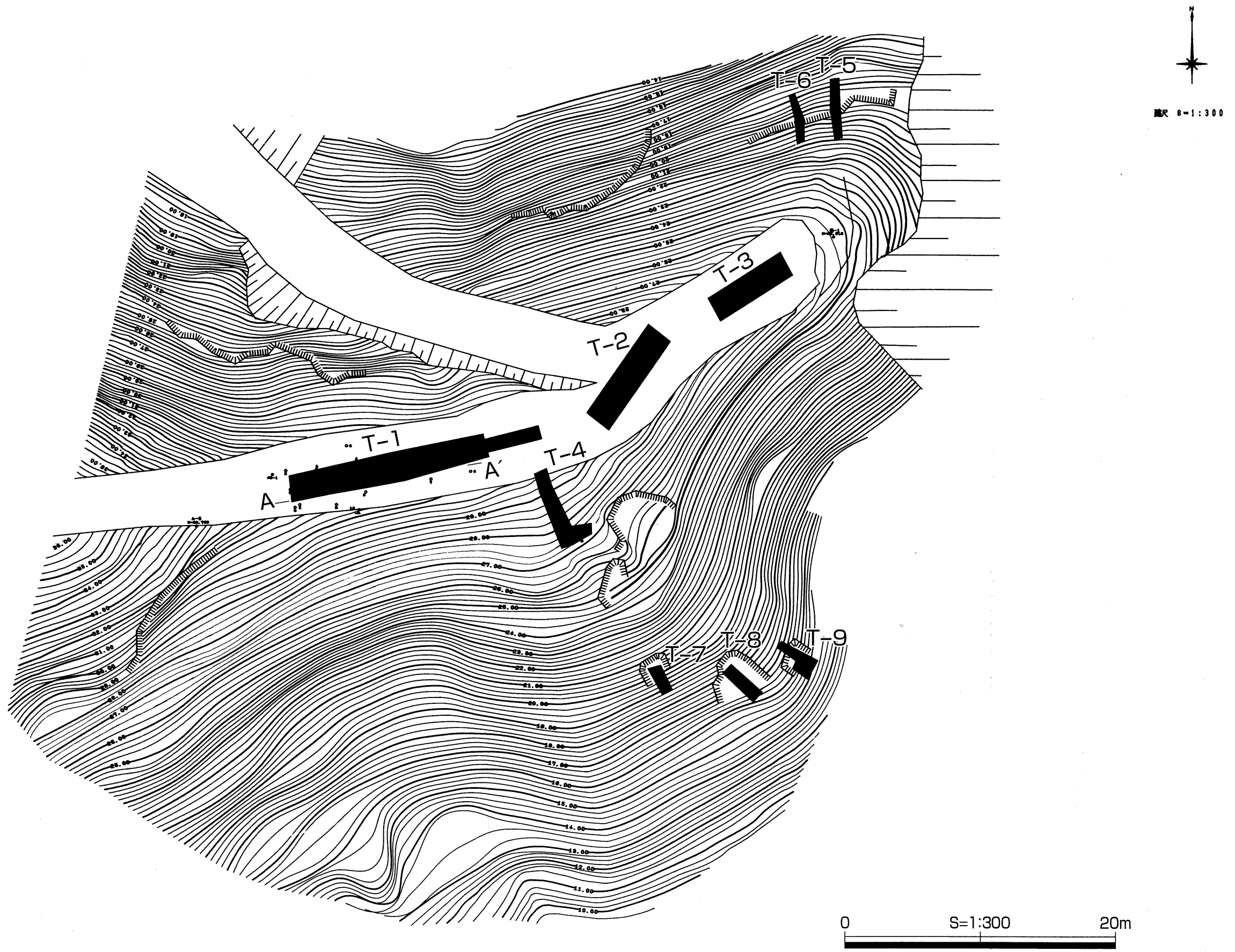
第3図 浦富地区試掘トレンチ配置図
